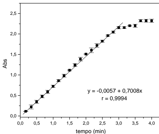
Figura 19. Gráfico Abs versus tempo para determinação da atividade enzimática da Lac.
