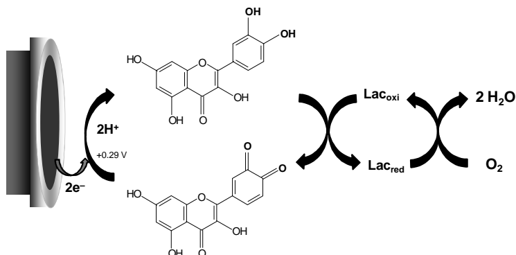
Figura 34. Esquema da reação de oxidação da quercetina catalisada pela enzima Lac e sua subsequente redução na superfície do eletrodo. Lac_{red} : lacase na forma reduzida e Lac_{oxi} : lacase na forma oxidada.
