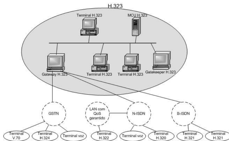
Figura 6: Visão Geral da Arquitetura H.323.
