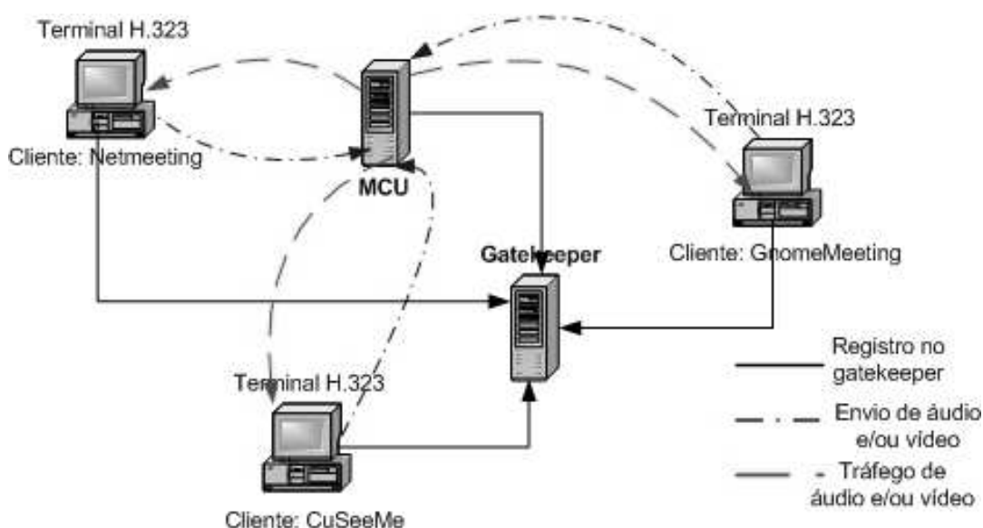
Figura 18: Experimento de validação do ambiente de videoconferência.
