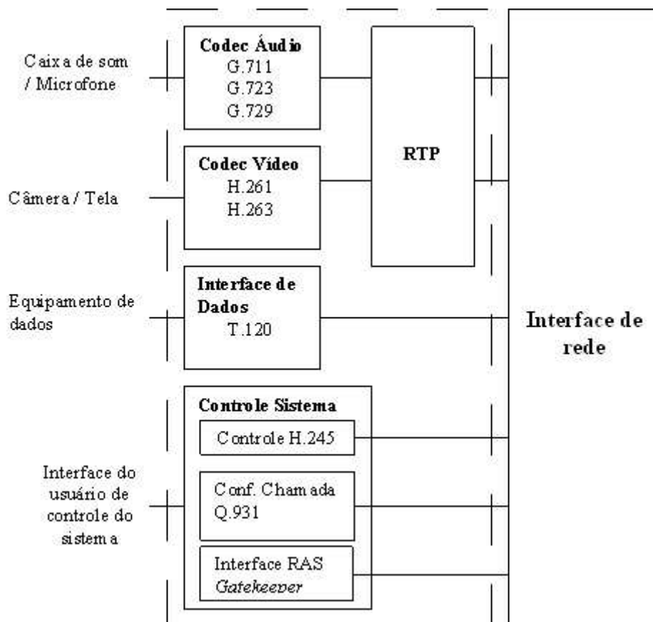
Figura 7: Componentes de um terminal H.323.
