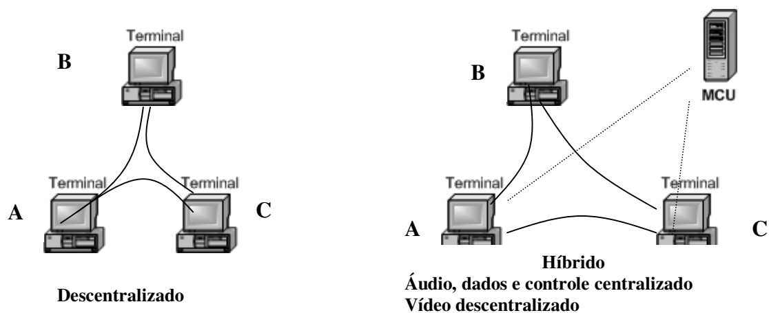
Figura 12: MCU – descentralizado e híbrido
