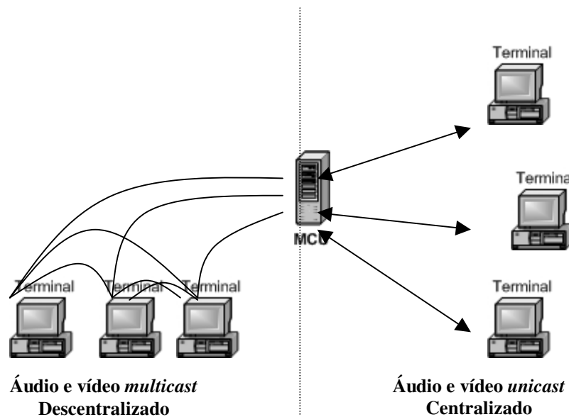
Figura 11: MCU – centralizado e descentralizado.
