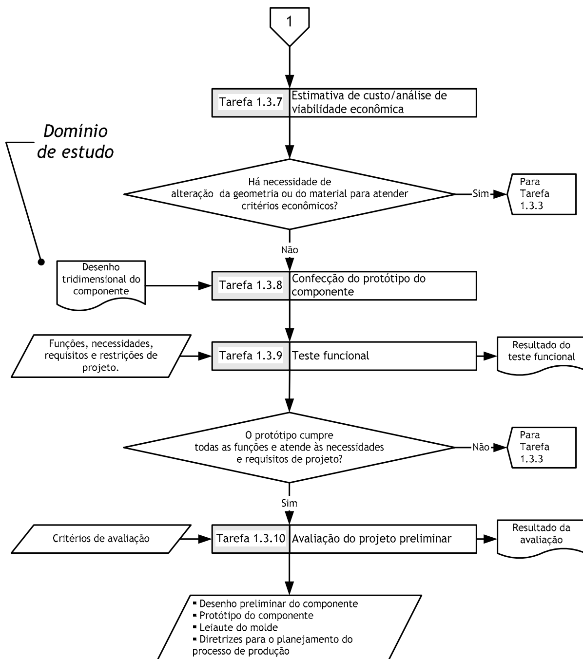
Figura 2-4: Etapa de projeto preliminar de componentes de plástico injetados (continuação) [2]
