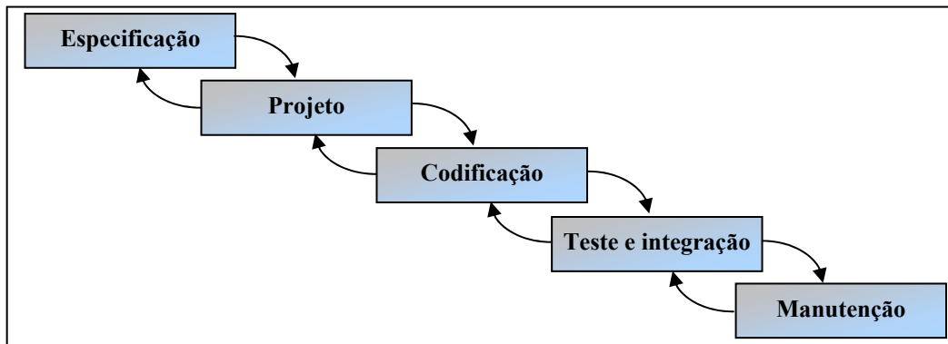
Figura 1: Diagrama simplificado do modelo cascata
