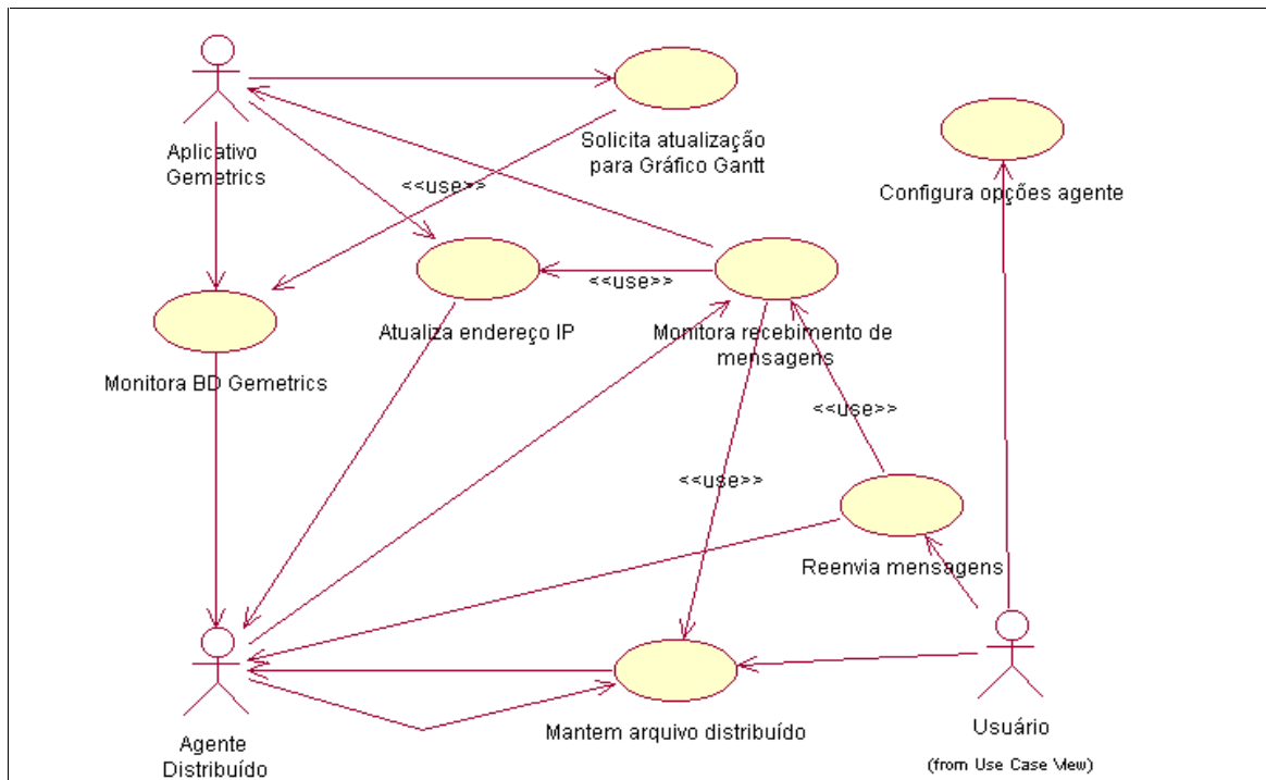
Figura 38: Diagrama de Casos de Uso - Agente para Gerenciamento Distribuído
