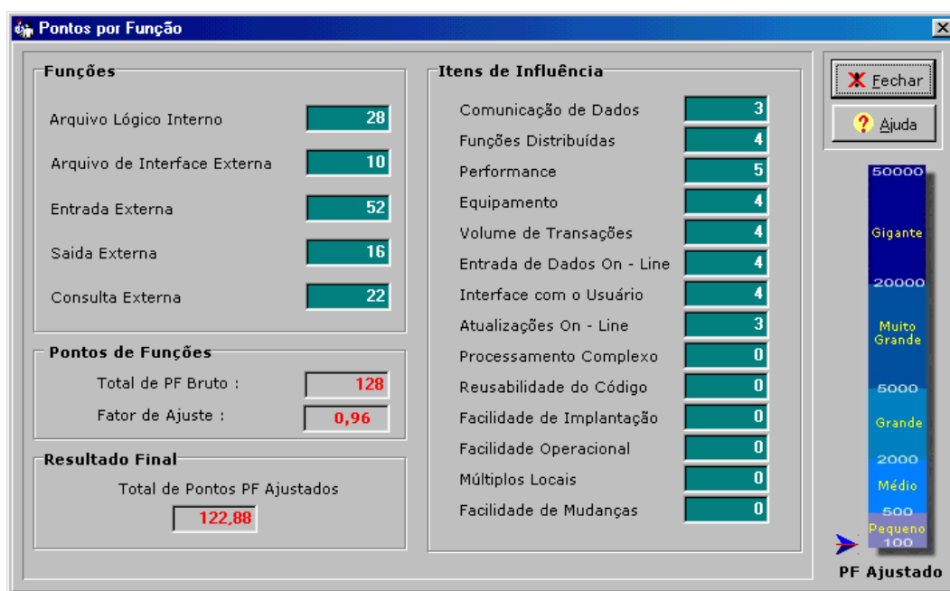
Figura 43: Cálculo de Pontos por Função
