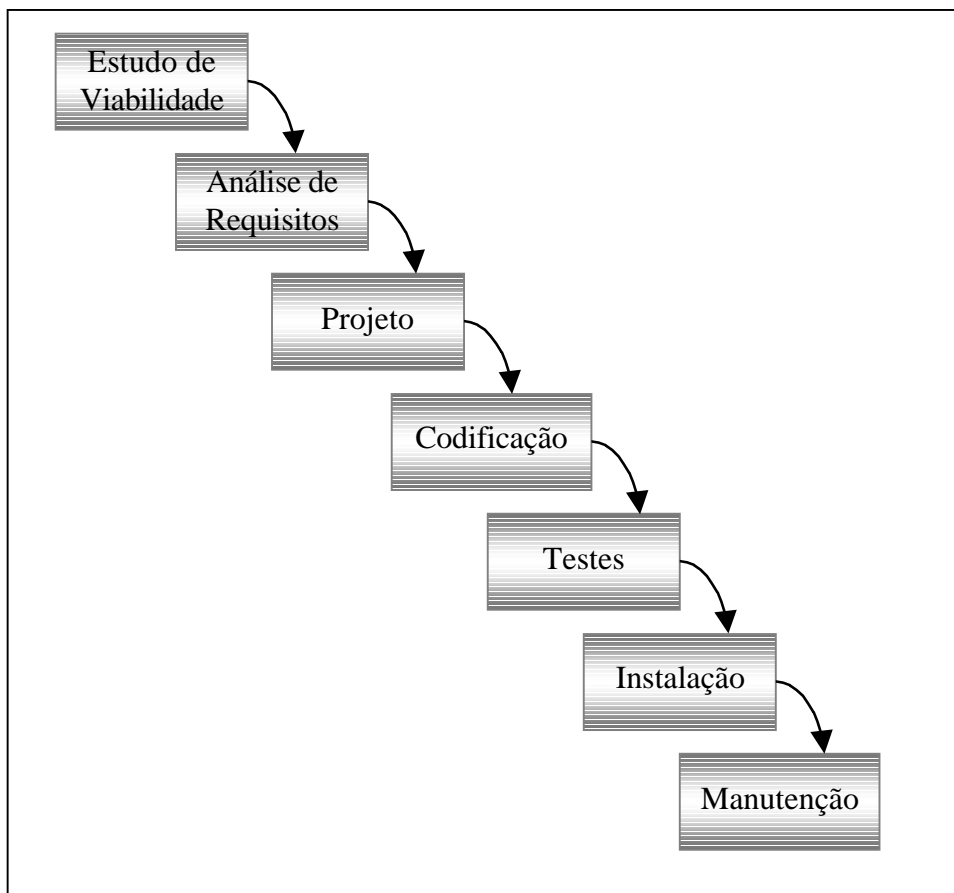
Figura 5: Modelo Cascata
