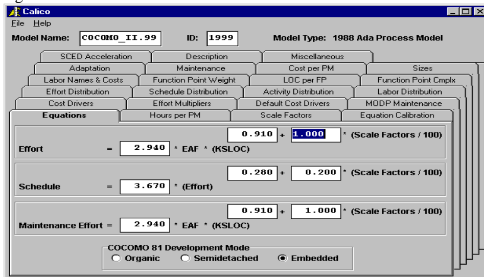
Figura 22: Interface Calico
