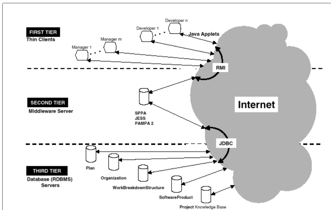
Figura 13: Arquitetura 3 camadas
