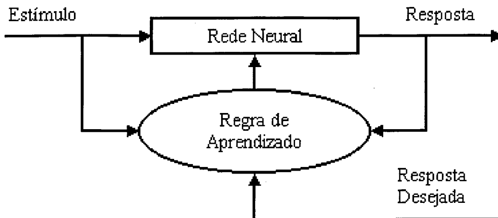
Figura 3.10: Aprendizado supervisionado.
