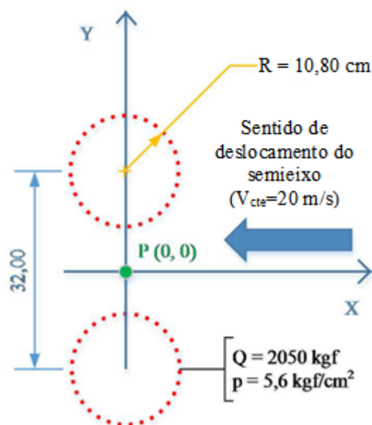
Figura 12: Configuração de carregamento (semieixo de roda dupla)
