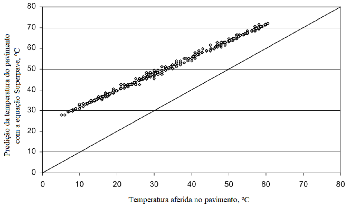
Figura 10: Comparação entre a predição da temperatura do pavimento com a equação do Superpave e medição instrumentada a 2 cm de profundidade
