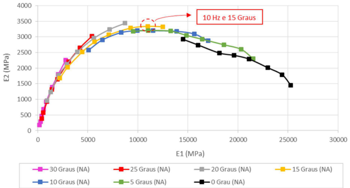
Figura 19: Plano complexo Cole-Cole
