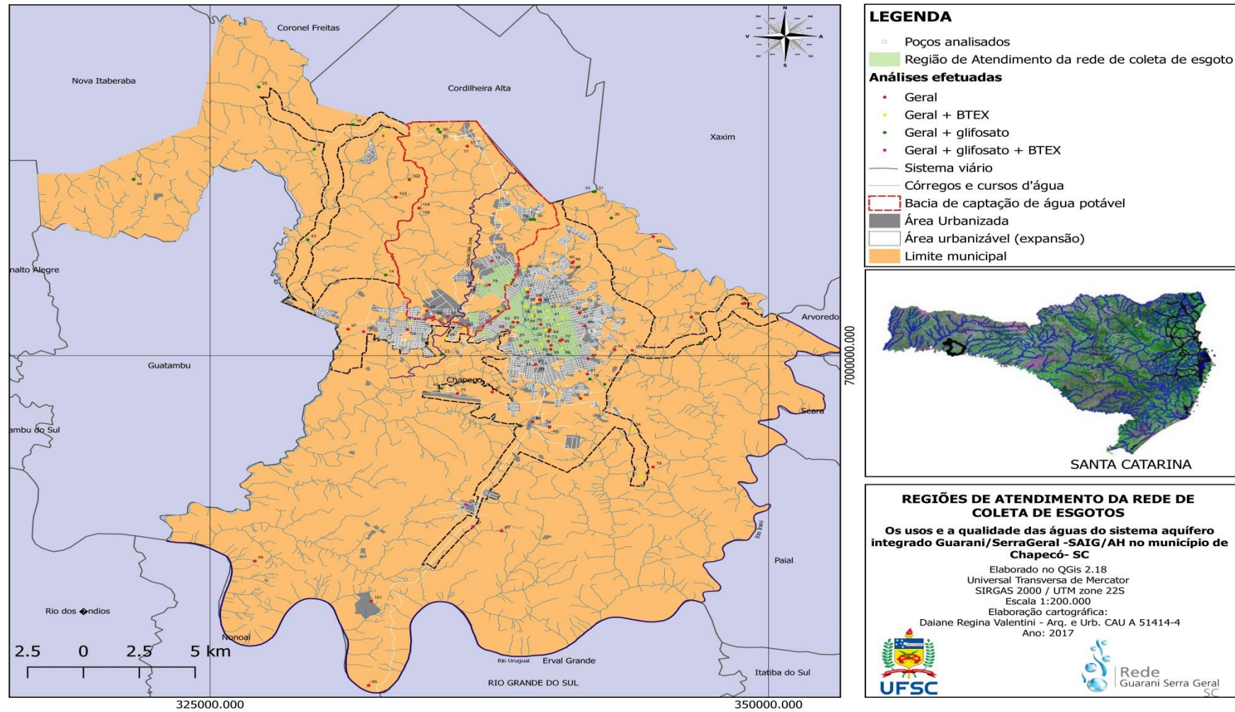
Figura 26 - Rede coletora de esgotamento sanitário de Chapecó-SC
