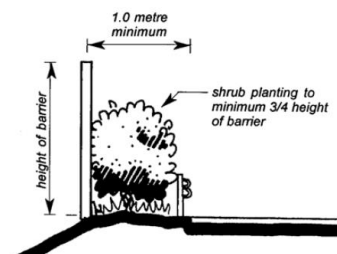
Figura 167: Vegetação mínima para barreira acústica. Fonte: Queensland, 2004, p. B4-9.
