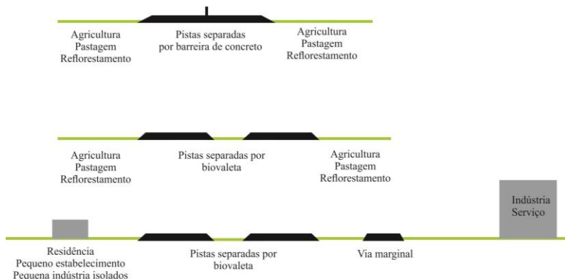
Figura 270: Tipologia de estrada na área rural - pistas no nível do entorno. Inserção de vias marginais quando existe área industrial ou urbanizada (vila, distrito). Dois tipos de separação de pista: blocos de concreto e biovaleta ou canteiro. A segunda opção é melhor sob o aspecto ecológico e visual.
