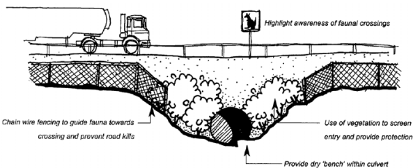
Figura 179: Tratamento de galerias para travessia de fauna. Fonte: Queensland, 2004, p. B8-5.
