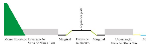
Figura 369 Padrão BR-101/SC Grande Florianópolis acesso às vias marginais e ao viaduto: faixas elevadas em relação à urbanização e às vias marginais. Fonte: Angela Favaretto, 2017.
