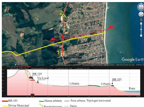
Figura 304: Perfil de elevação, BR-101/SC em Barra Velha, divisa com Piçarras.
