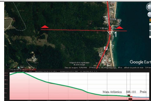
BR-101 Mata Atlântica Mar Figura 329: Perfil de elevação da BR-101/SC em Itapema. Está inserida na planície e seu entorno encontra-se urbanizado com verticalização a leste, próximo da costa. Fonte: Angela Favaretto, 2017, a partir de Google Earth, 2017.
