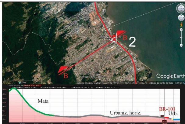
Figura 361: Perfil de elevação da BR-101/SC em São José. A densidade urbana é maior que em Biguaçu e segue assim esse padrão em Palhoça. A rodovia está bastante próxima da costa nesse trecho e possibilita algumas visuais para o mar. São limites para a urbanização a costa e os morros. Fonte: Angela Favaretto, 2017, a partir de Google Earth, 2017.
