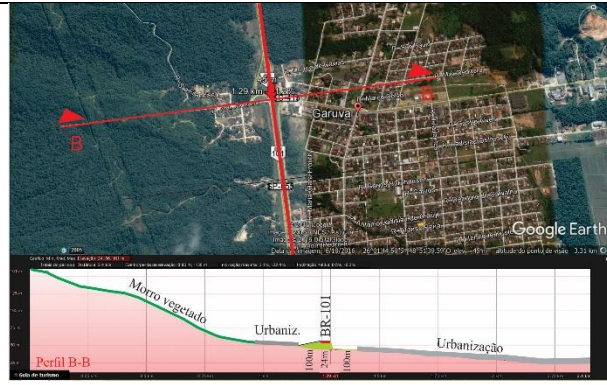
Figura 279: Perfil de elevação B-B, BR-101/SC em área urbana de Garuva.
