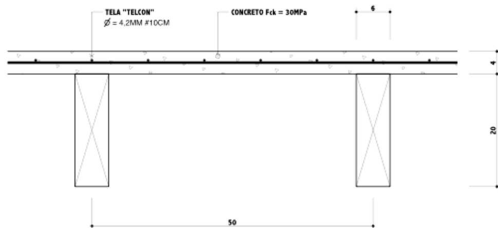
SEÇÃO TRANSVERSAL ESCALA 1:5
