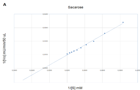
Figura 4.10 – Gráficos duplo-recíprocos da hidrólise de sacarose (A), rafinose (B) e maltotriose (C), pela enzima presente na linhagem GMY08 crescida em meio YP-4% glicose.
