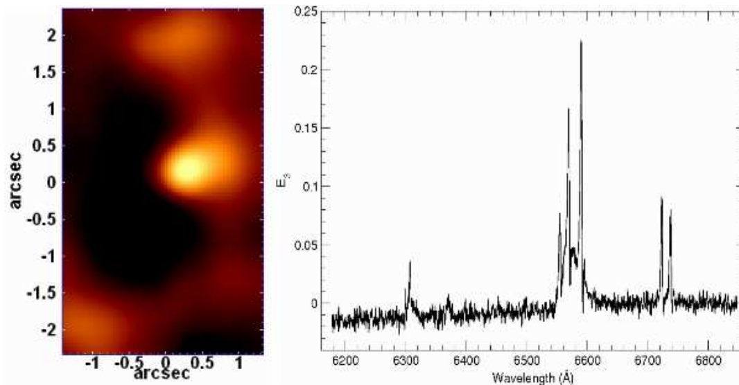
Figura 3.6: Autoespectro 3 e seu respectivo tomograma. Retirado de S09.
