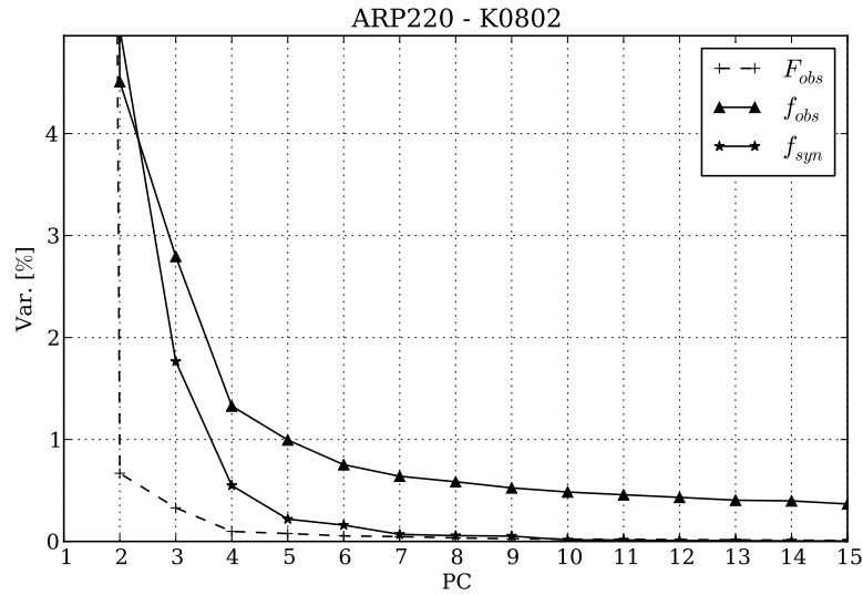
Figura 5.38: Igual a Figura 5.2 para a galáxia ARP 220.
