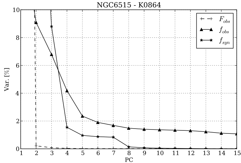
Figura 5.26: Igual a Figura 5.2 para a galáxia NGC 6515.
