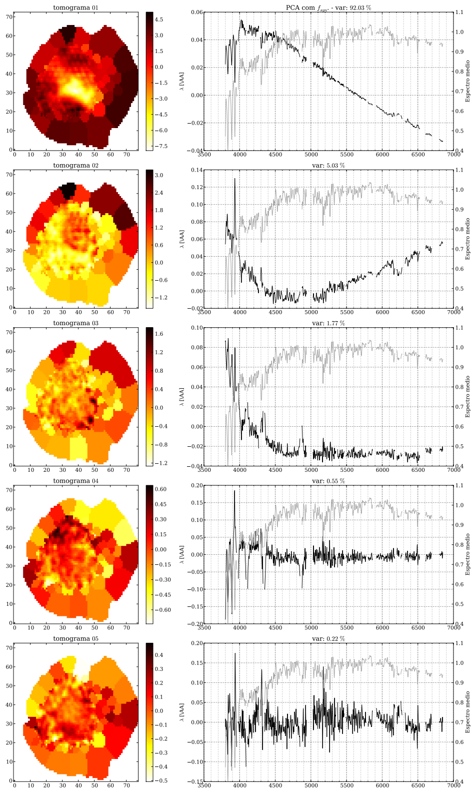
Figura 5.40: Igual a Figura 5.4 para a galáxia ARP 220.
