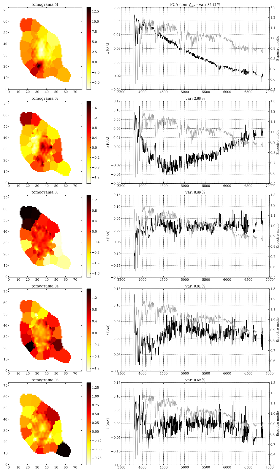
Figura 5.33: Igual a Figura 5.3 para a galáxia NGC 2623.
