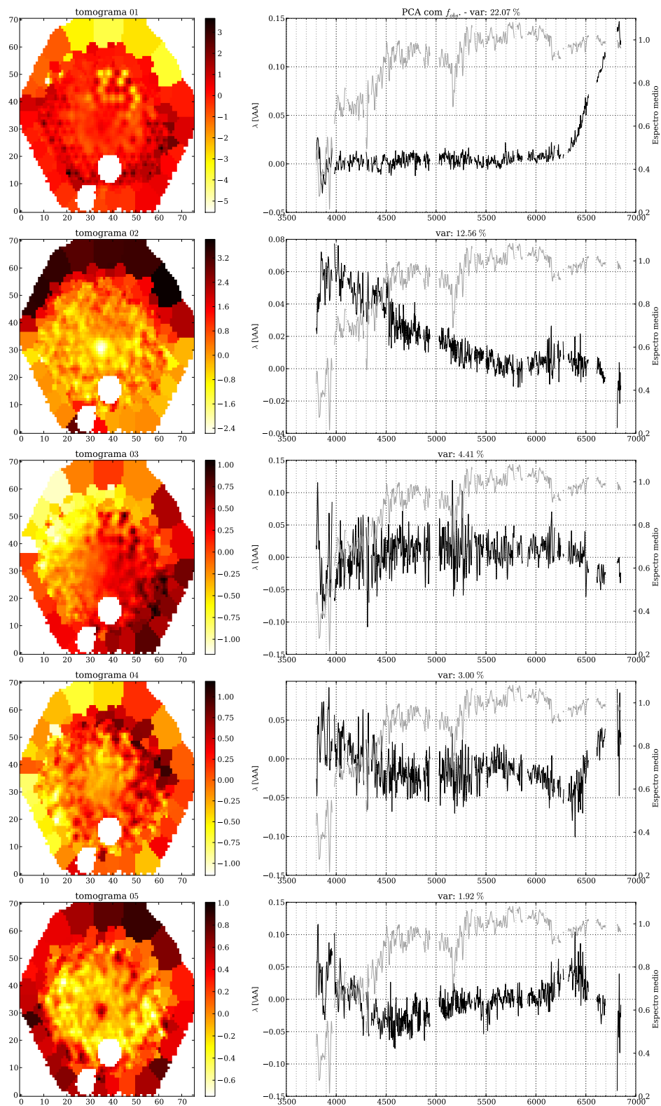
Figura 5.21: Igual a Figura 5.3 para a galáxia NGC 1167.
