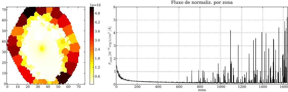
Figura 4.5: Fluxo usado para a normalização de cada espectro, mostrado tanto na forma de imagem (à esquerda) como em função do número da zona (direita).
