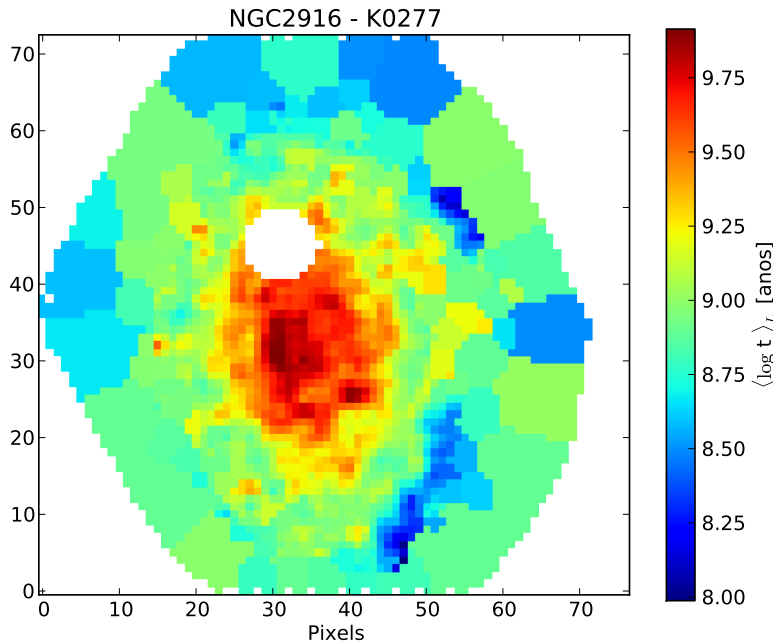
Figura 2.7: Mapa de idade estelar média ponderada pela luminosidade da galáxia NGC 2916 (CALIFA 277) gerado pelo programa da Figura 2.6.
