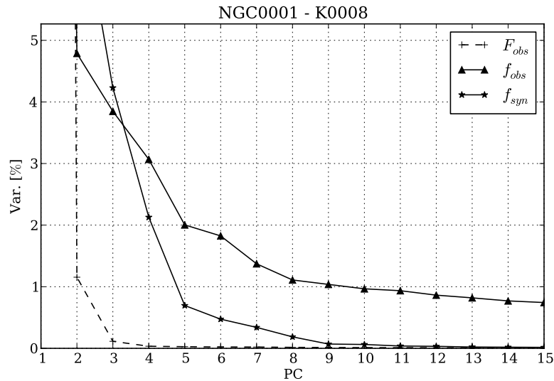
Figura 5.2: Scree test para 3 análises PCA da galáxia NGC 0001 (CALIFA 8). Com marcações de triângulos vemos as PCs resultantes do PCA com os espectros observados normalizados ( f_{obs} ). As variâncias das PCs marcadas com estrela representam o PCA com os espectros sintéticos normalizados ( f_{syn} ). Para comparação plotamos as PCs do caso sem normalização ( F_{obs} ) usando linha pontilhada.
