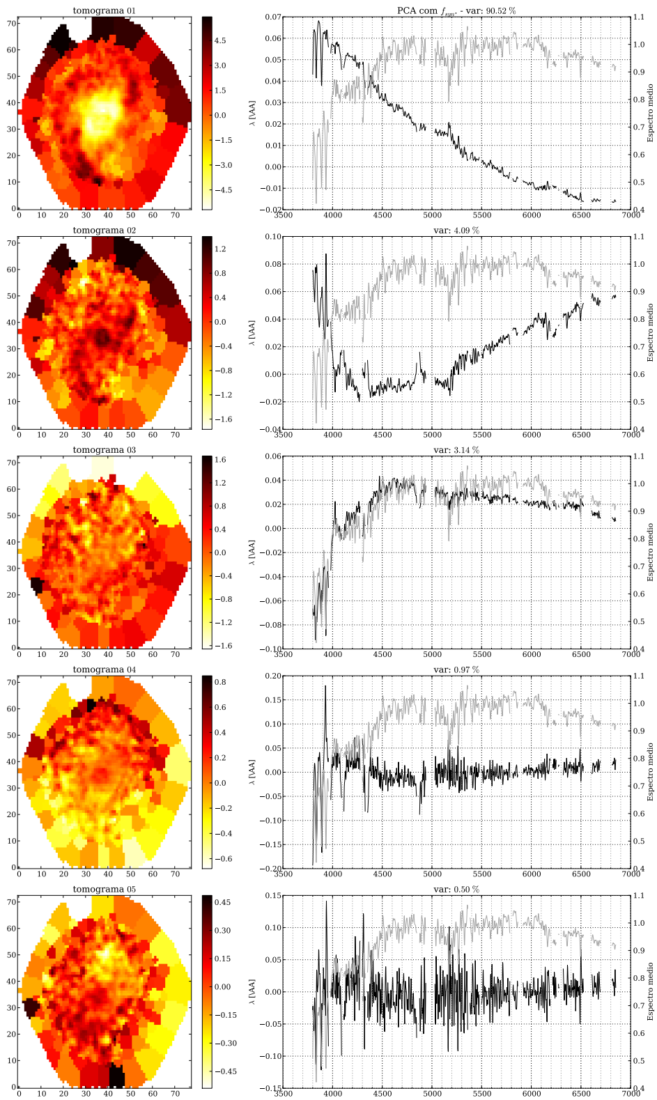
Figura 5.10: Igual a Figura 5.4 para a galáxia NGC 0776.
