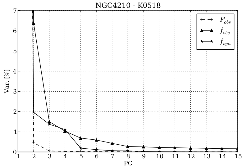
Figura 5.14: Igual a Figura 5.2 para a galáxia NGC 4210.
