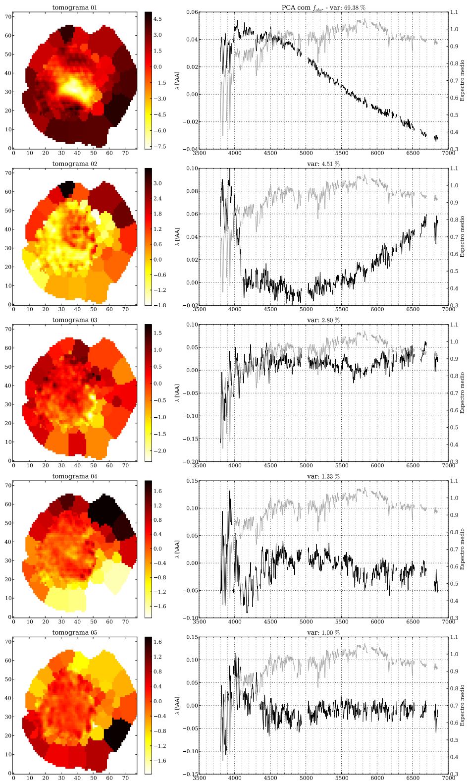
Figura 5.39: Igual a Figura 5.3 para a galáxia ARP 220.
