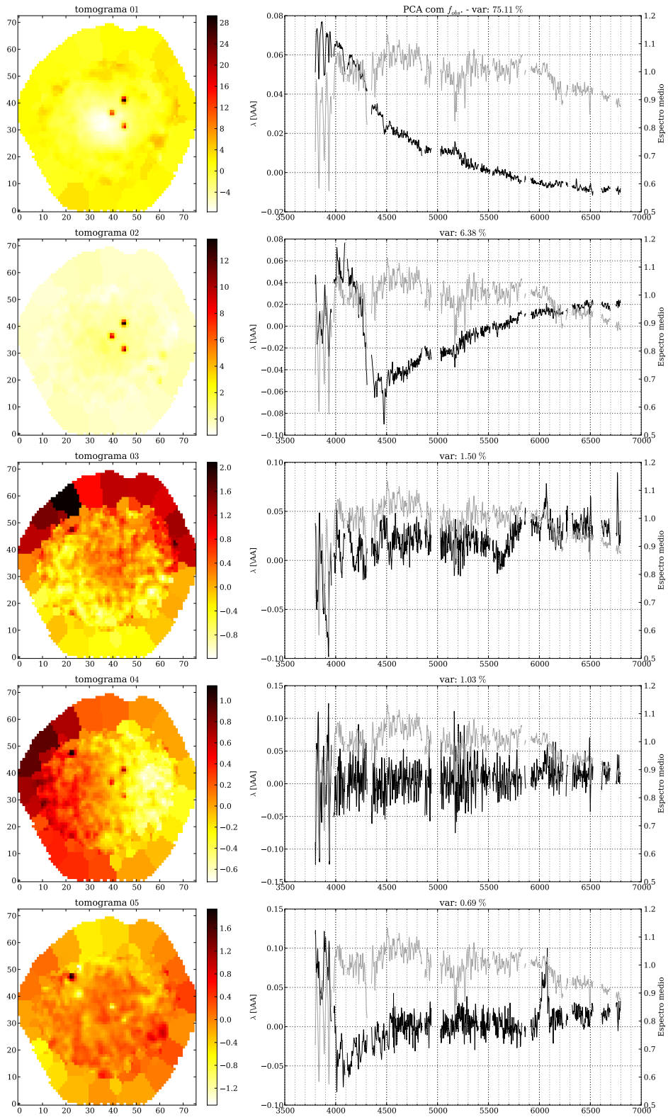
Figura 5.15: Igual a Figura 5.3 para a galáxia NGC 4210.
