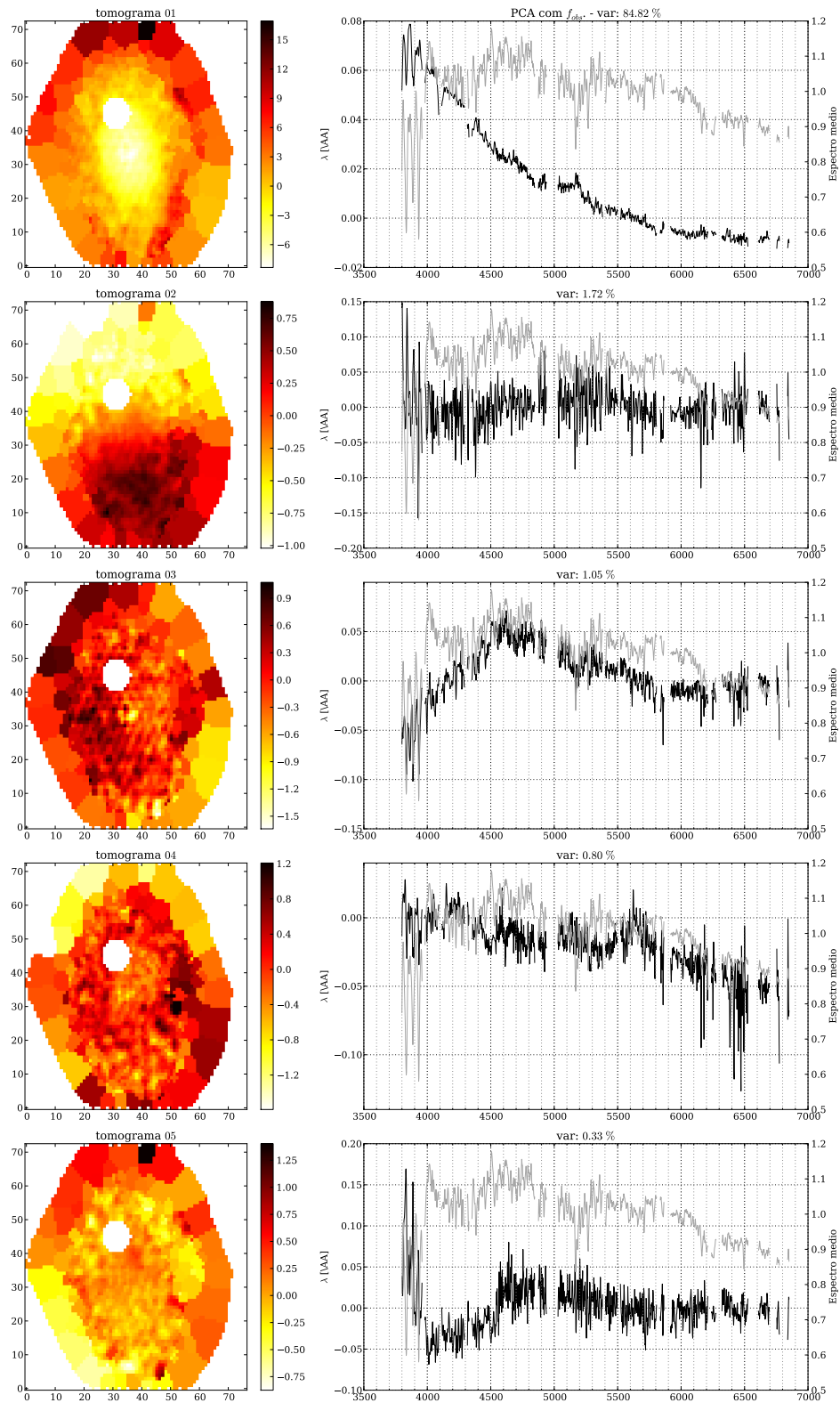
Figura 4.4: Cinco primeiras PCs (em preto à direita) e seus respectivos tomogramas (imagem à esquerda) resultantes da Tomografia PCA aplicado aos espectros observados normalizados ( f_{obs} ) da galáxia NGC 2916. Em cinza o espectro médio para comparação.
