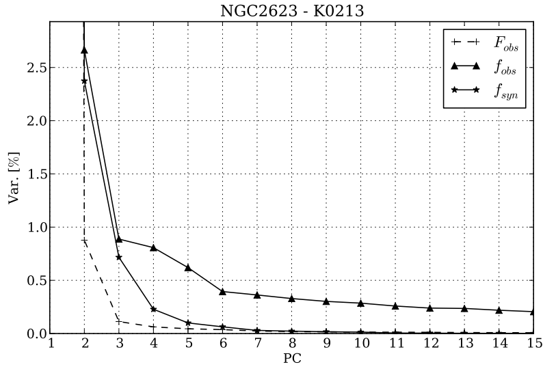
Figura 5.32: Igual a Figura 5.2 para a galáxia NGC 2623.
