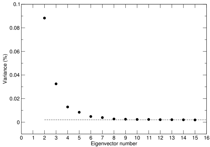
Figura 3.3: Scree test das primeiras 16 PCs do cubo de espectros da região central da galáxia NGC 4736. Retirado de S09.
