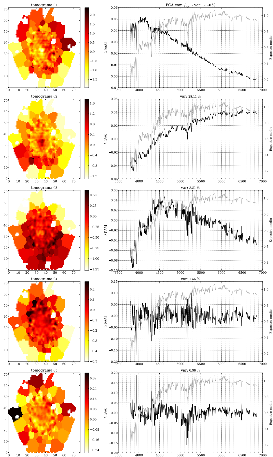
Figura 5.28: Igual a Figura 5.4 para a galáxia NGC 6515.
