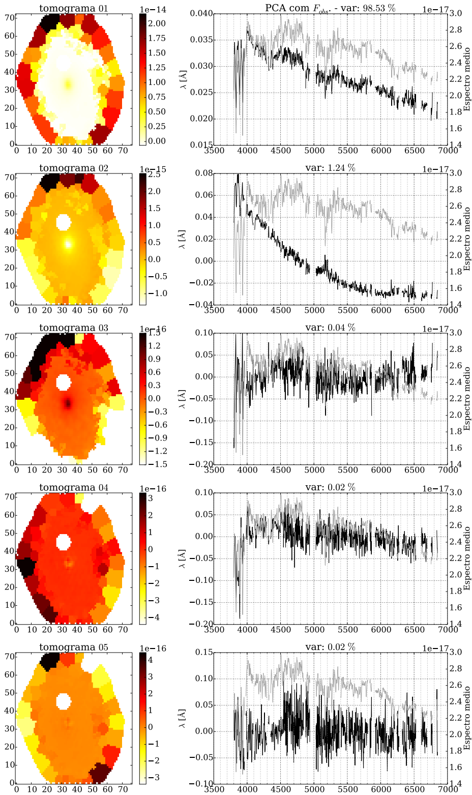
Figura 4.3: Cinco primeiras PCs (em preto à direita) e seus respectivos tomogramas (imagem à esquerda) resultantes da Tomografia PCA aplicado aos espectros sem normalização ( F_{obs} ) da galáxia NGC 2916. Em cinza o espectro médio para comparação.
