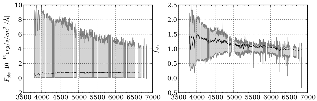
Figura 4.2: Fluxo máximo e mínimo por comprimento de onda para o cubo de espectros da galáxia NGC 2916 (CALIFA 277). O painel à esquerda é para os espectros observados ( F_{obs} ) e o à direita para os espectros observados e normalizados pelo fluxo mediano na janela de 5635 \pm 45 \text{ \AA} ( f_{obs} ). Em destaque o 95º percentil. Todos os espectros do cubo já estão mascarados da mesma forma que o terceiro painel da Figura 2.3
