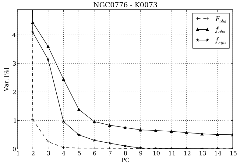
Figura 5.8: Igual a Figura 5.2 para a galáxia NGC 0776.
