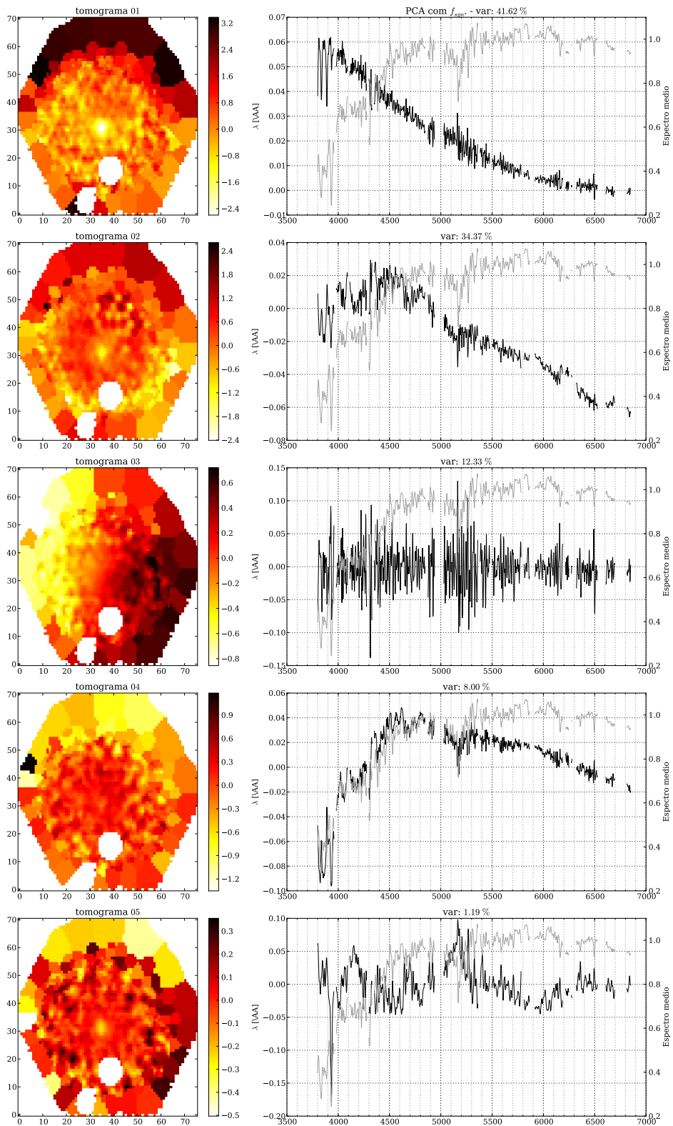
Figura 5.22: Igual a Figura 5.4 para a galáxia NGC 1167.
