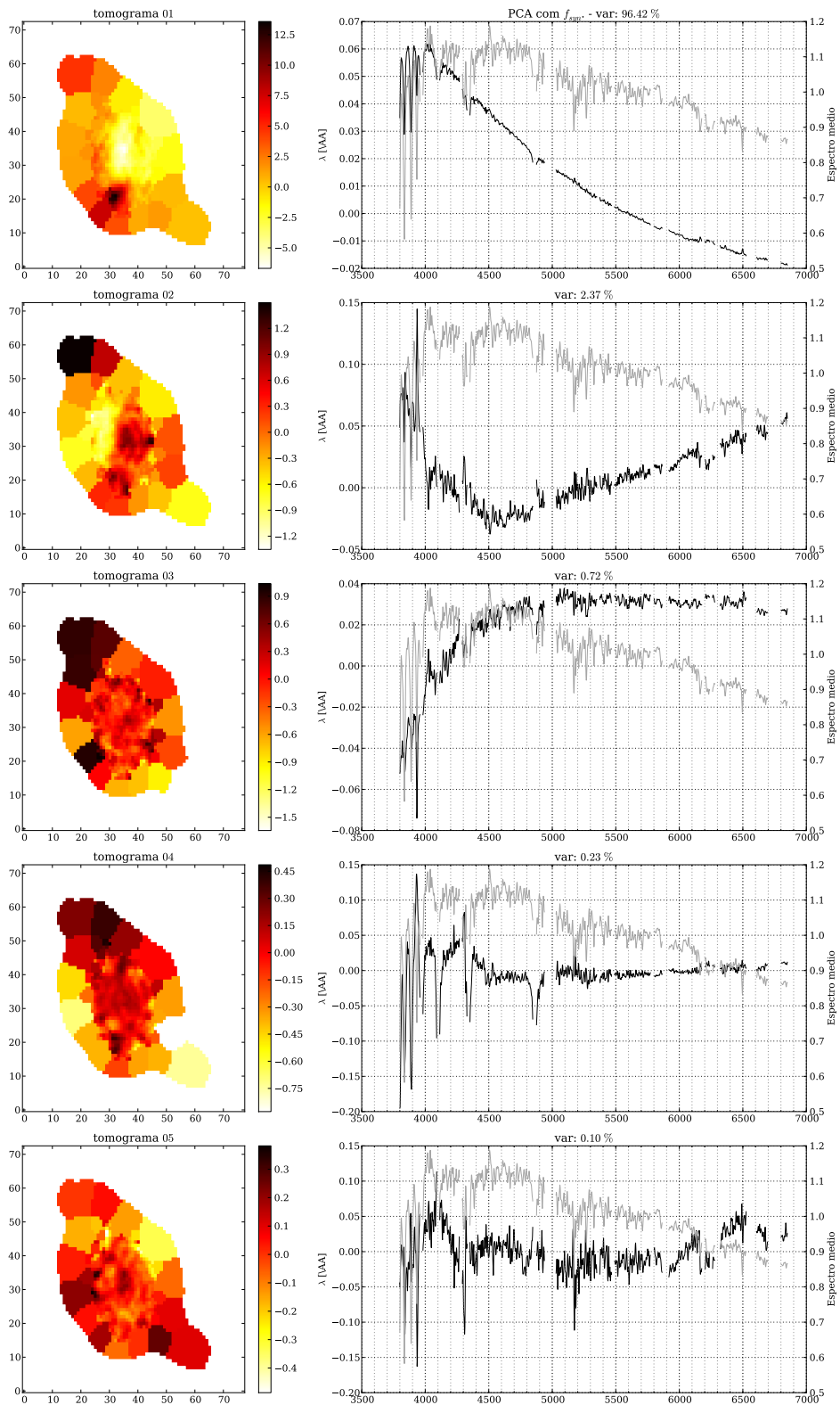
Figura 5.34: Igual a Figura 5.4 para a galáxia NGC 2623.
