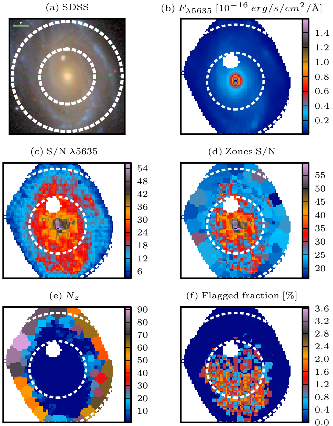
Figura 2.4: (a) Imagem SDSS para a galáxia NGC 2916 (CALIFA 277). (b) Fluxo no intervalo de 5635 \pm 45 Å depois da aplicação da máscara espacial. (c) Mapa da relação S/N em 5635 Å. (d) Mapa da relação S/N depois da zonificação de Voronoi. (e) Número de spaxels em cada zona de Voronoi. (f) Percentagem de bad pixels no intervalo de 3800–6850 Å. Retirado de CF13.
