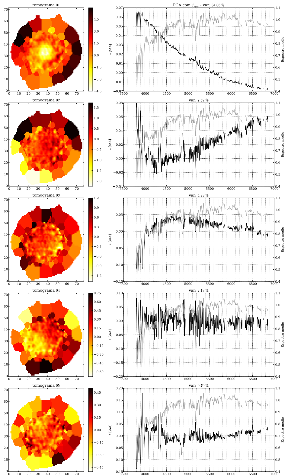
Figura 5.4: Cinco primeiras PCs (e seus respectivos tomogramas) resultantes da Tomografia PCA aplicado aos espectros sintéticos normalizados ( f_{syn} ) da galáxia NGC 0001.
