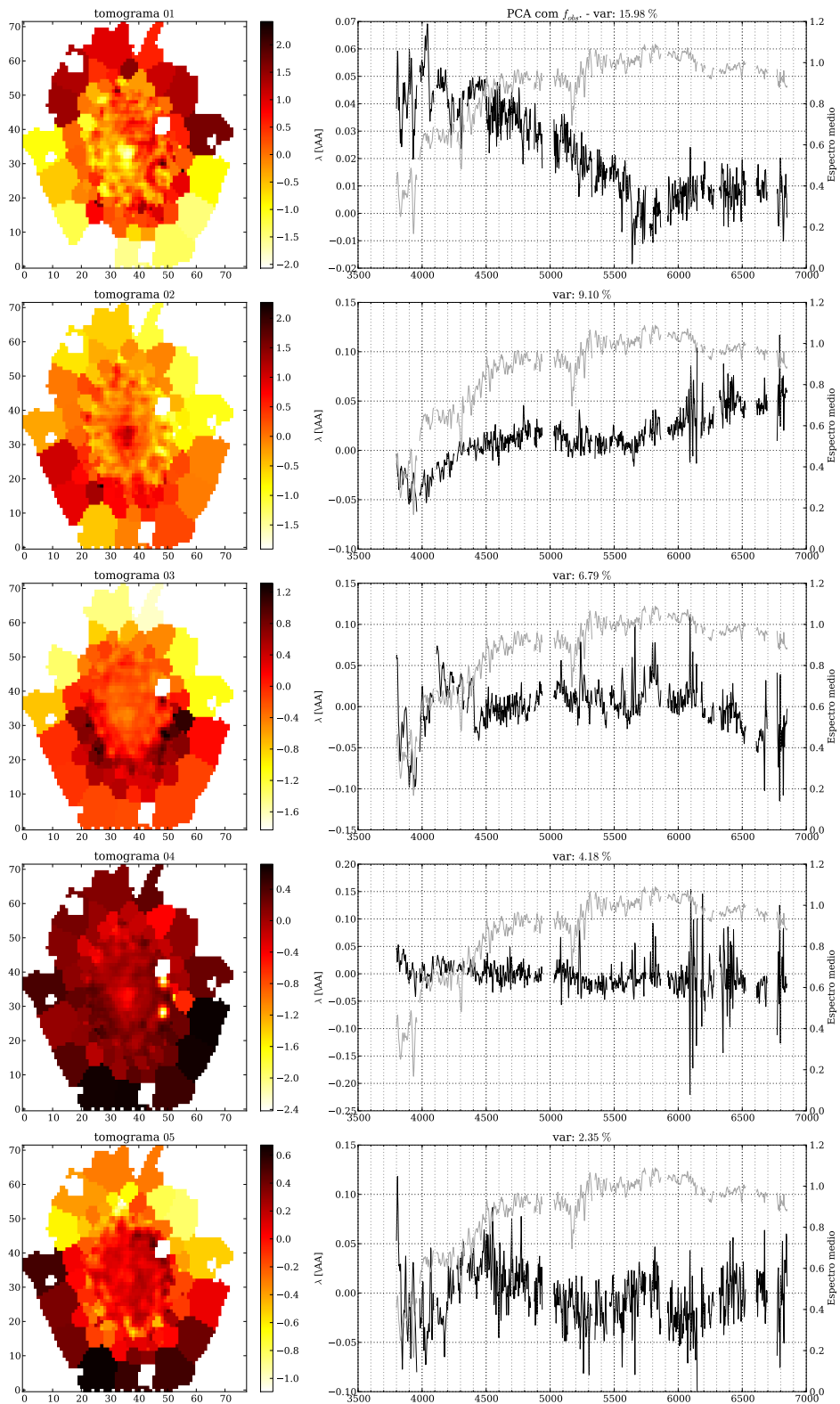
Figura 5.27: Igual a Figura 5.3 para a galáxia NGC 6515.
