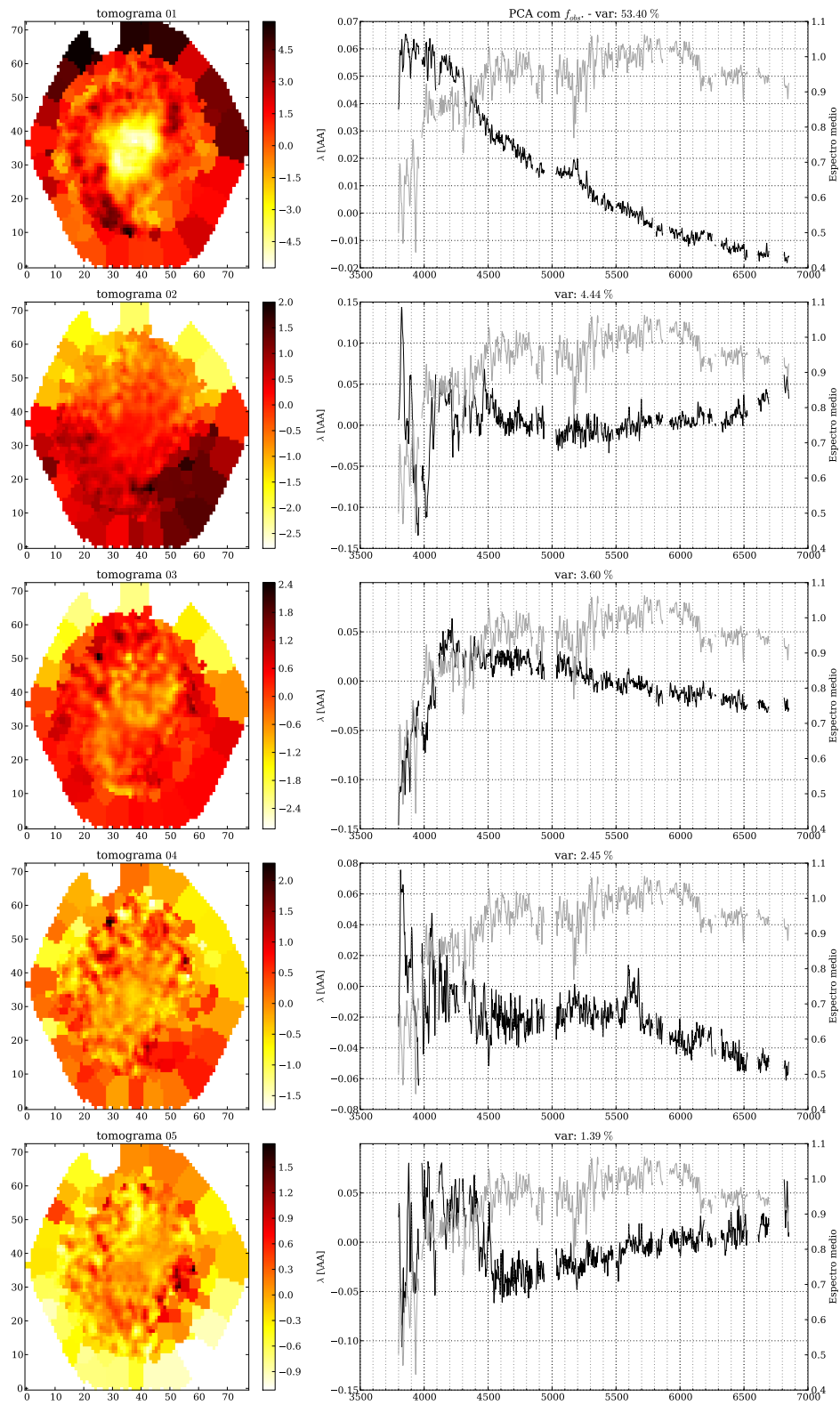
Figura 5.9: Igual a Figura 5.3 para a galáxia NGC 0776.
