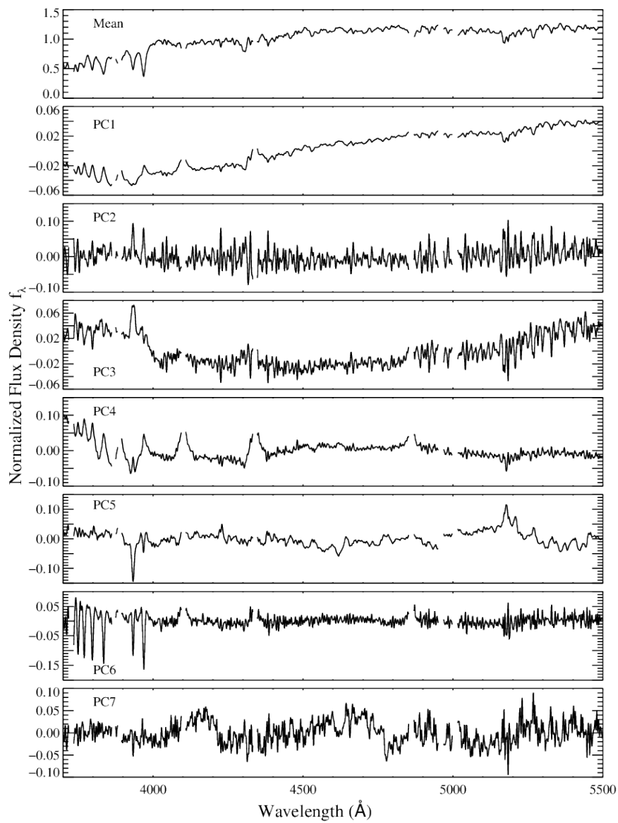
Figura 1.1: De cima para baixo: O espectro médio da biblioteca de espectros modelos seguido dos sete primeiros autoespectros da análise PCA. Retirado de Chen et al. (2012).
