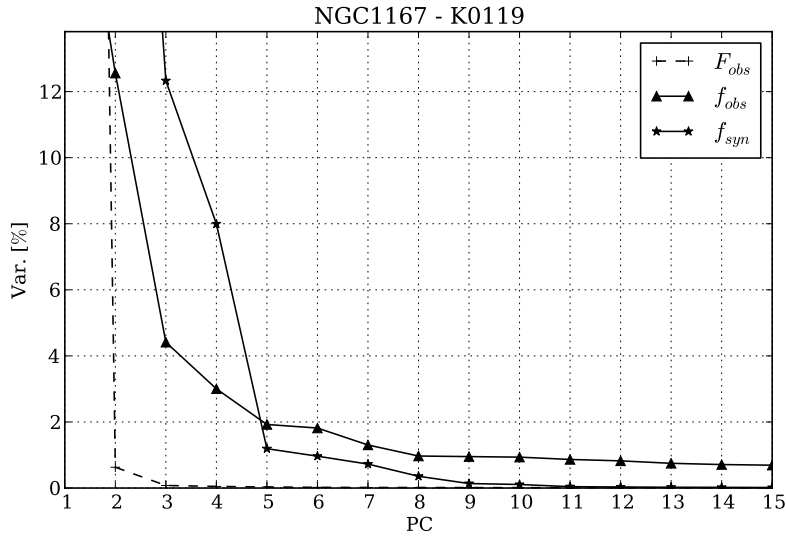
Figura 5.20: Igual a Figura 5.2 para a galáxia NGC 1167.
