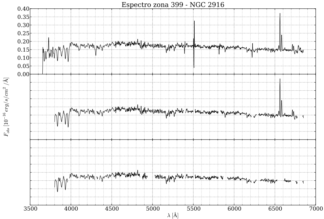
Figura 2.3: Espectro da zona 399 da galáxia NGC 2916 (CALIFA 277). Acima está o espectro completo. No segundo vemos o espectro com linhas telúricas e pixels problemáticos removidos, além do limite de intervalo em comprimento de onda de 3800 a 6850 Å. No espectro mais abaixo, além das partes removidas no segundo, foram removidas também as mesmas linhas de emissão mascaradas na síntese de populações estelares.
