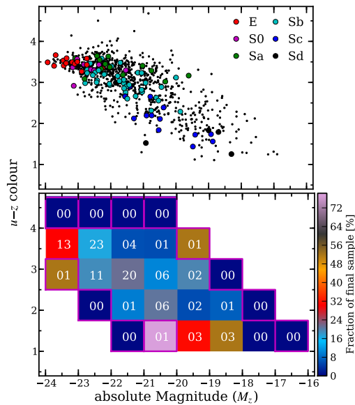
Figura 2.1: Distribuição das galáxias do CALIFA no diagrama cor magnitude u-z vs. M_z . Painel superior: Em pontos pretos estão as galáxias pertencente a amostra-mãe e em cores as galáxias presentes no CALIFA DR1. As diferentes cores representam os diferentes tipos morfológicos. Painel inferior: A fração de galáxias observadas pelo DR1 em relação a amostra-mãe. Retirado de Husemann et al. (2013).
