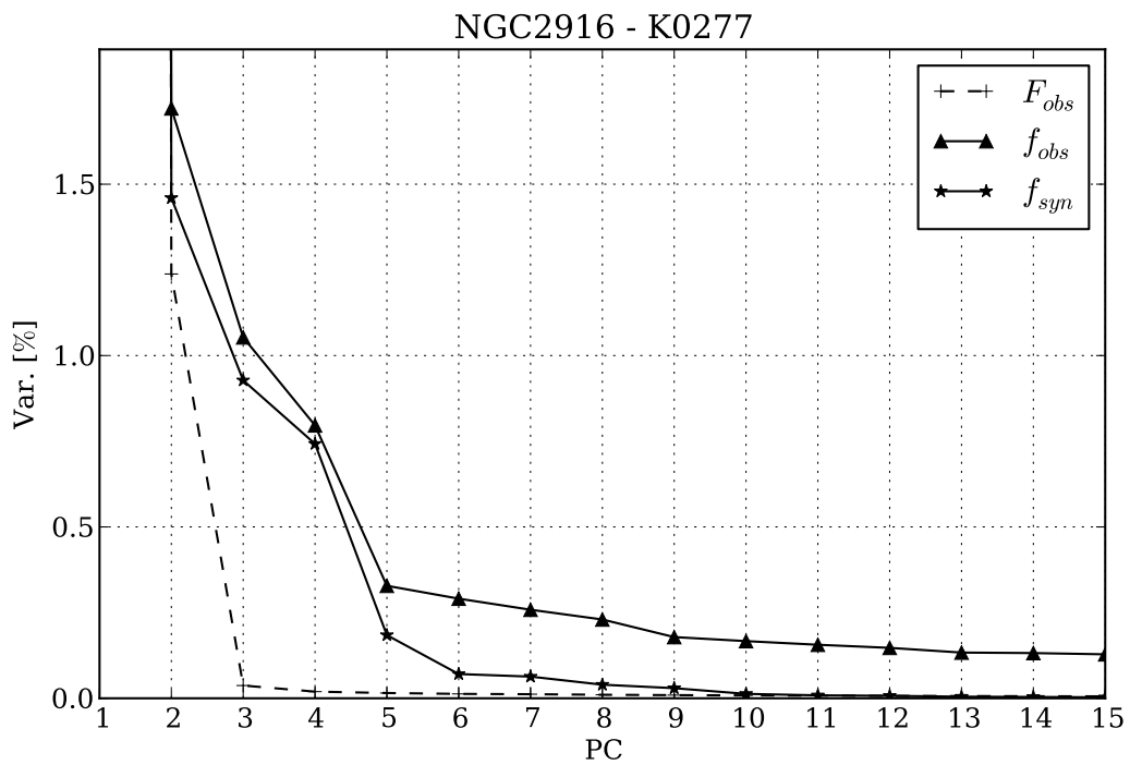
Figura 4.6: Scree test para 3 PCAs da galáxia NGC 2916 (CALIFA 277). Com marcações de triângulos vemos as PCs resultantes da PCA com os espectros observados normalizados ( f_{obs} ). As variâncias das PCs marcadas com estrela representam a PCA com os espectros sintéticos normalizados ( f_{syn} ). Para comparação plotamos as PCs do caso sem normalização ( F_{obs} ) usando linha pontilhada.
