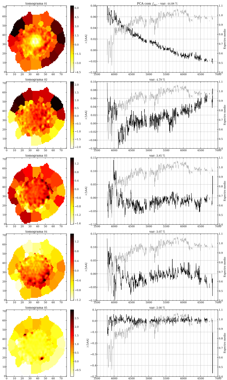
Figura 5.3: Cinco primeiras PCs (e seus respectivos tomogramas) resultantes da Tomografia PCA aplicado aos espectros observados normalizados ( f_{obs} ) da galáxia NGC 0001.
