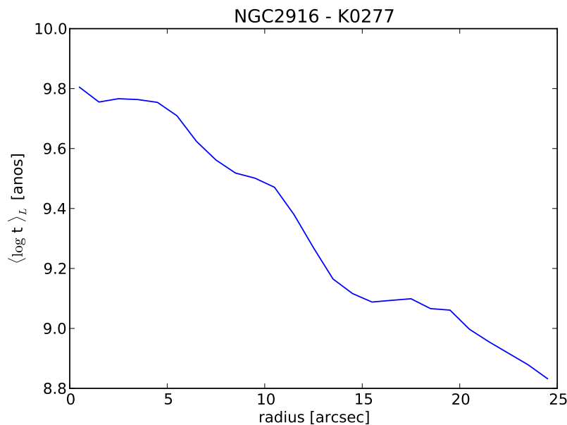
Figura 2.9: Perfil radial da idade estelar média ponderada pela luminosidade da galáxia NGC 2916 (CALIFA 277) gerado pelo programa da Figura 2.8.
