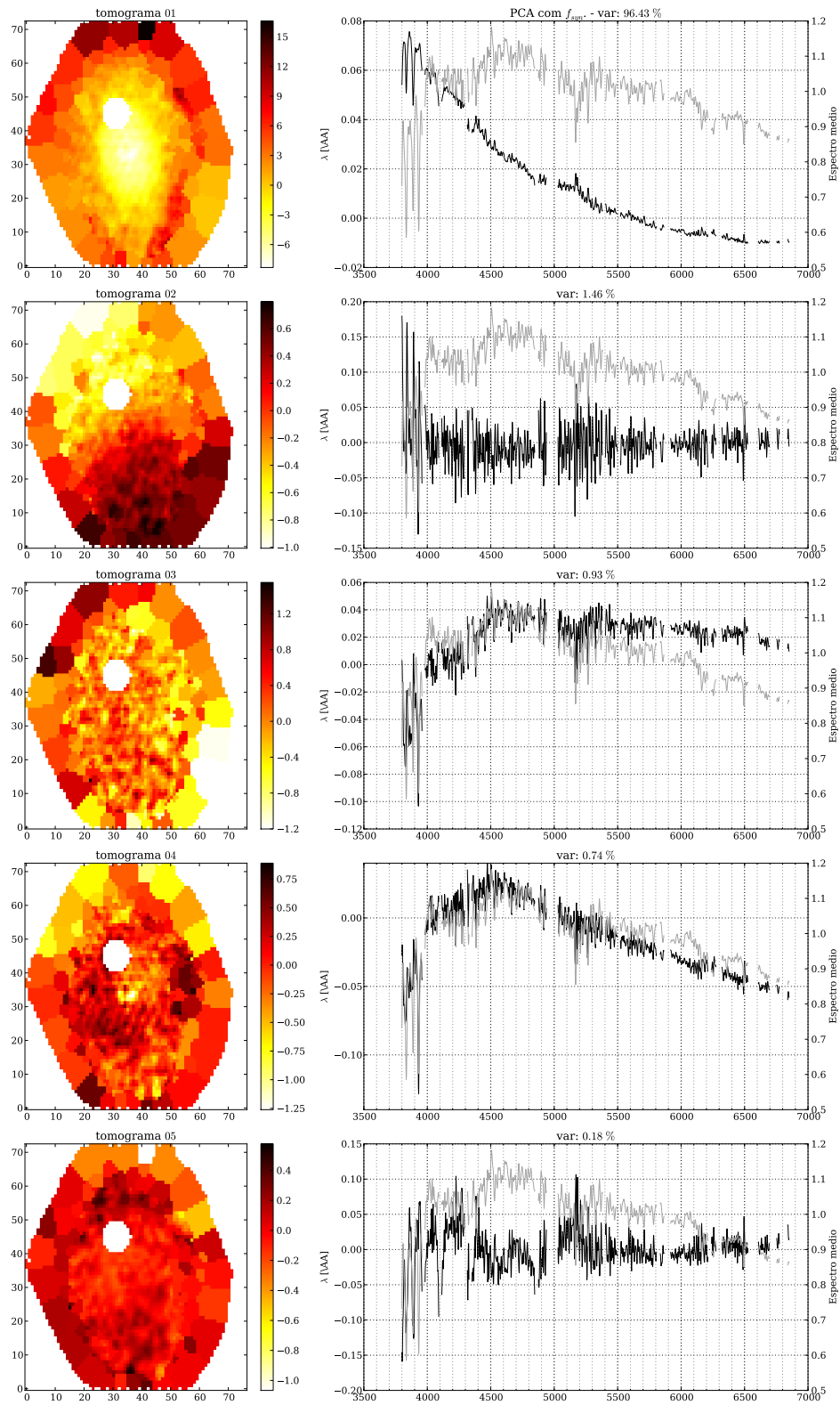
Figura 4.7: Cinco primeiras PCs (e seus respectivos tomogramas) resultantes da Tomografia PCA aplicado aos espectros sintéticos normalizados ( f_{syn} ) da galáxia NGC 2916.
