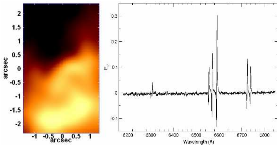
Figura 3.5: Autoespectro 2 e seu respectivo tomograma. Retirado de S09.
