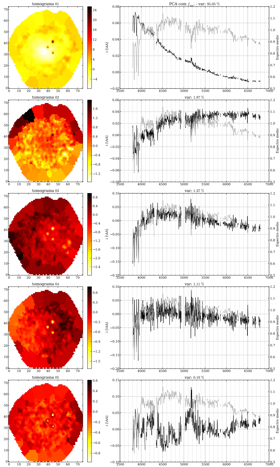
Figura 5.16: Igual a Figura 5.4 para a galáxia NGC 4210.
