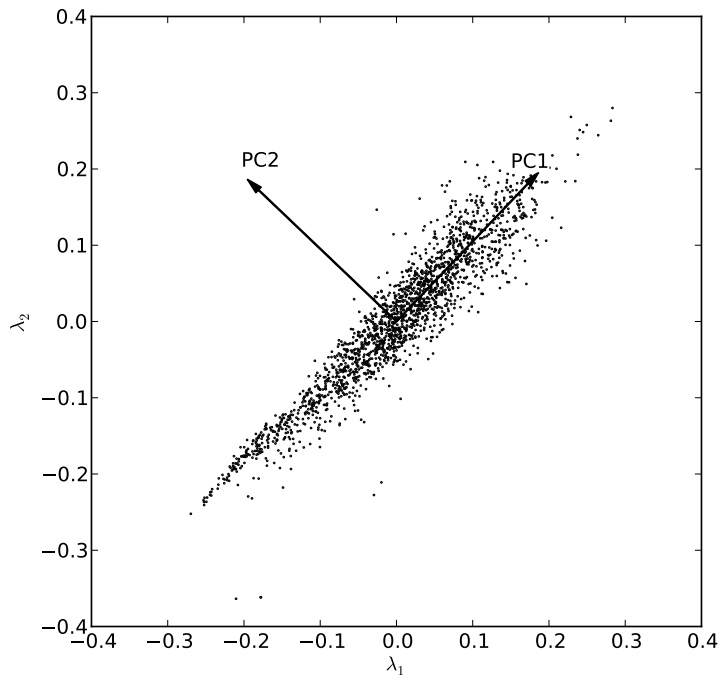
Figura 3.1: Análise PCA para espectros contendo apenas dois comprimentos de onda. Cada ponto no gráfico representa um espectro observado em dois comprimentos de onda, \lambda_1 e \lambda_2 . A PC1 representa a direção onde está contida a maior variância nos dados. A segunda PC (PC2) é a segunda direção com maior variância calculada com as restrições de ser ortonormal à primeira.
