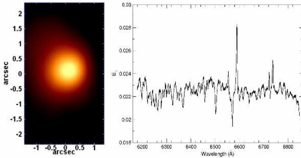
Figura 3.4: Autoespectro 1 e seu respectivo tomograma. Retirado de S09.
