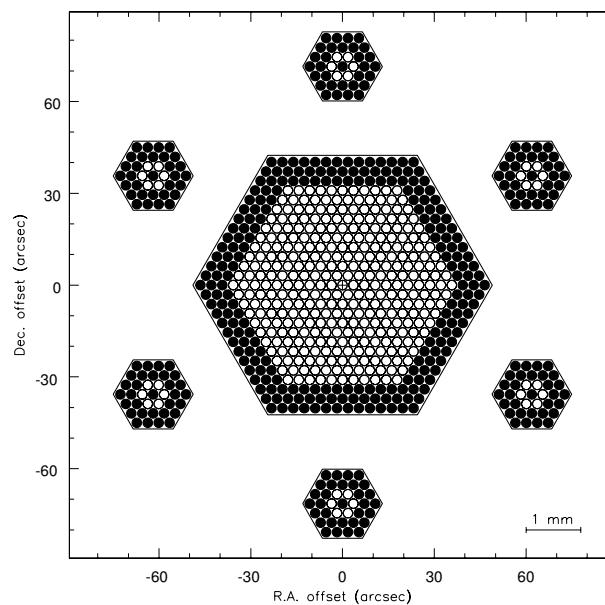
Figura 2.2: Este é o esquema com o bundle hexagonal com as 331 fibras de observação e mais 36 de amostra de céu. Retirado de Verheijen et al. (2004).
