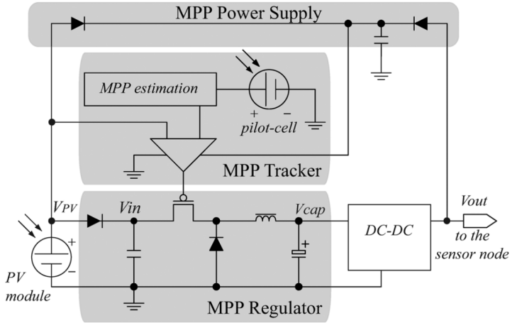
Figura 12 – Diagrama da proposta MPPT com célula piloto.
