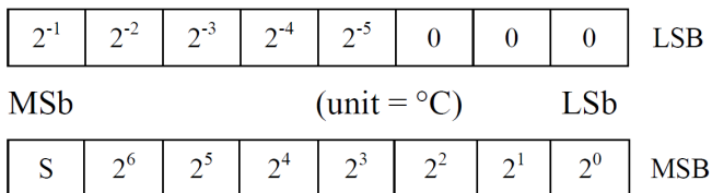
Figura 23 – Registrador de temperatura do DS2438.
