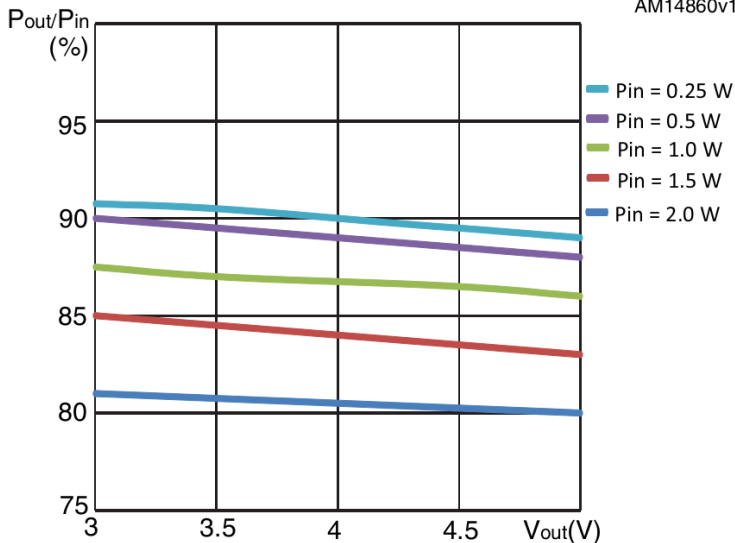
Figura 54 – Eficiência do SPV1040 para tensão de entrada de 1,5 V. AM14860v1
