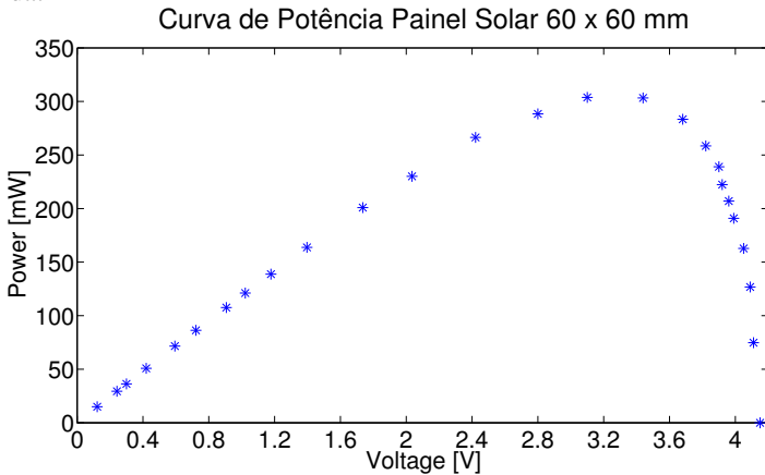
Figura 18 – Caracterização do painel solar 60 x 60 mm - curva potência fornecida.
