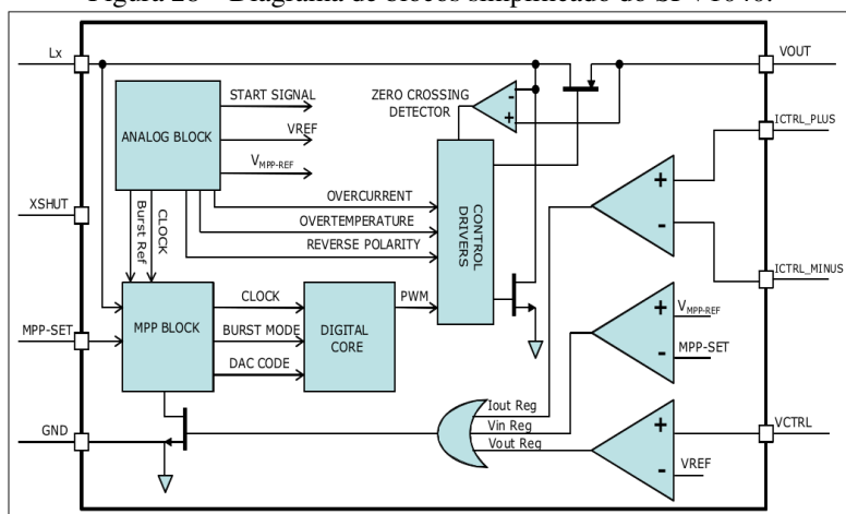
Figura 28 – Diagrama de blocos simplificado do SPV1040.
