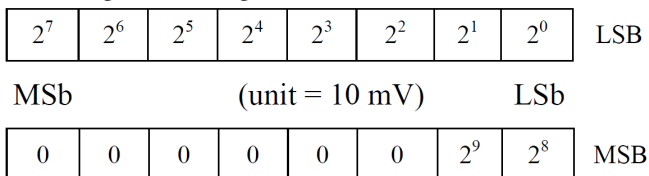
Figura 24 – Registrador de tensão do DS2438.
