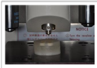
Fig.16-17 - Execução do teste de microdureza Vickers
