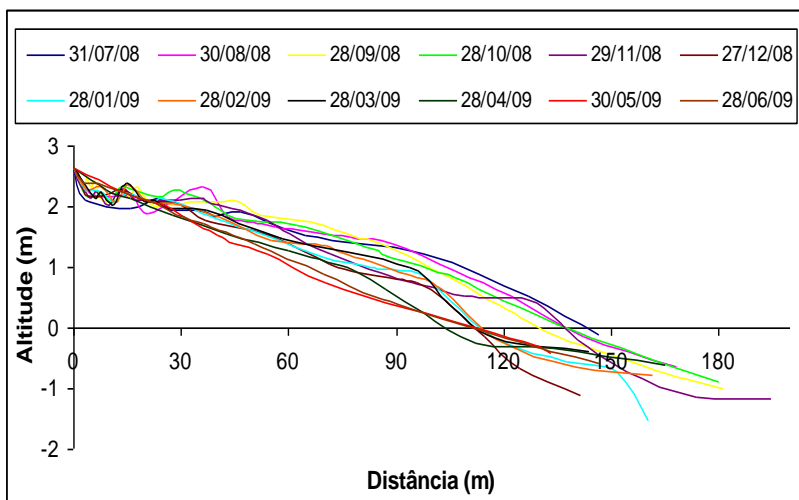
Figura 19. Morfologia praial observada no perfil 6, setor norte da praia de Itapirubá.
