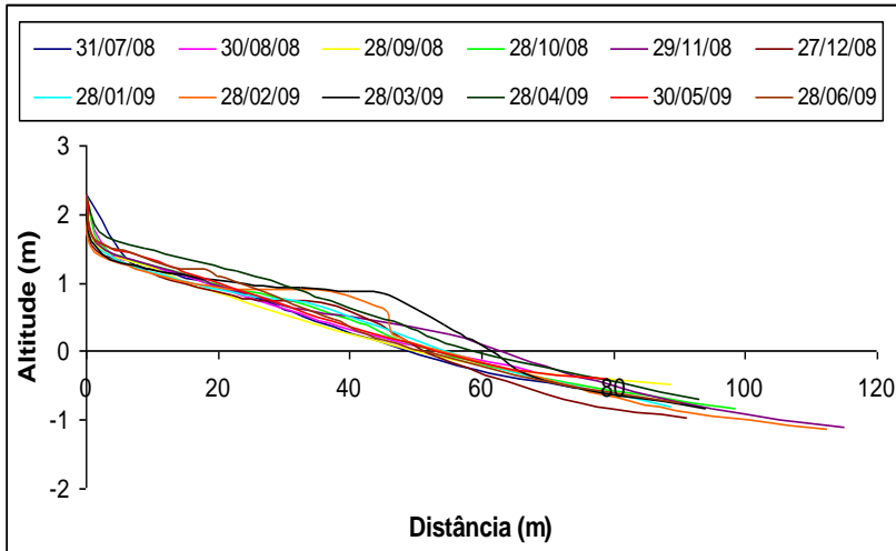
Figura 9. Morfologia praial observada no perfil 1, setor norte da praia de Itapirubá.
