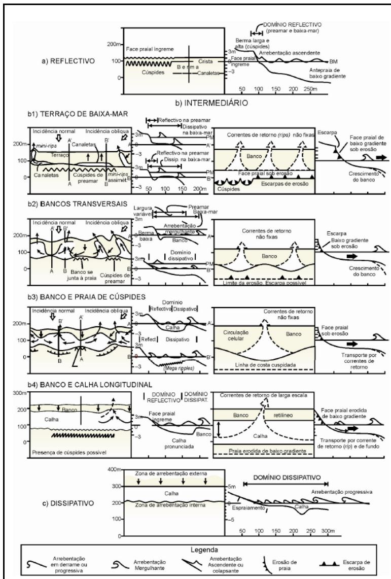
Figura 3. Representação dos estágios morfo-dinâmicos de praias arenosas oceânicas (Fonte: CALLIARI et al. , 2003).
