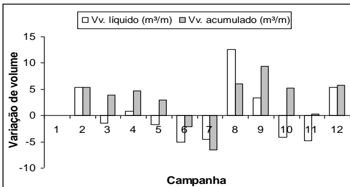
Figura 16. Variação do volume líquido e volume acumulado no Perfil 4.
