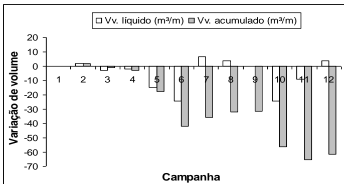
Figura 20. Variação do volume líquido e volume acumulado no perfil 6.
