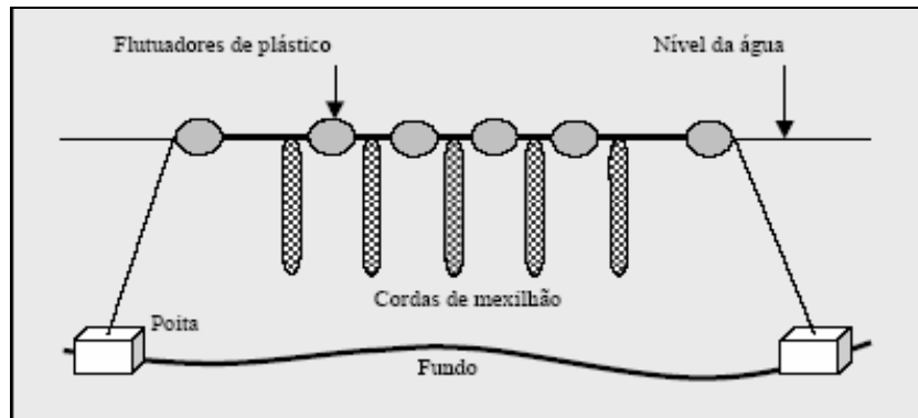
Figura 8 - Sistema de cultivo long-line ou espinhel Fonte: Arana (2000)
