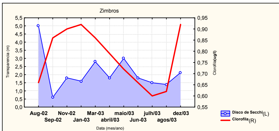
Figura 25g - Variação da concentração de clorofila "a" ( \mu\text{g/l} ) de superfície e da transparência (m) na coluna d'água entre 2002 e 2003, em "Zimbros", do setor Centro-Norte do litoral de Santa Catarina
