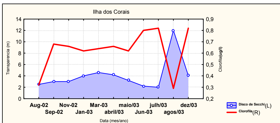
Figura 27a - Variação da concentração de clorofila "a" ( \mu\text{g/l} ) de superfície e da transparência (m) na coluna d'água entre 2002 e 2003, em "I. Corais", do setor Centro-Sul do litoral de Santa Catarina
