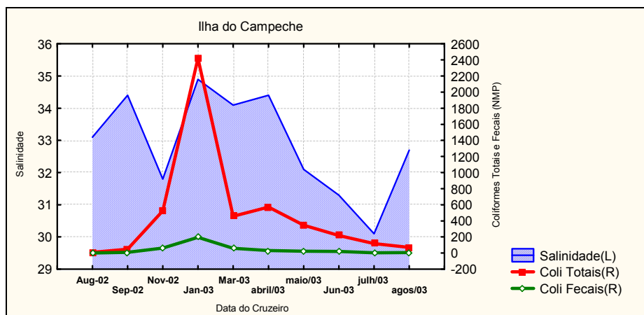
Figura 41b - Relação exibida entre os parâmetros Coliformes Totais e Fecais (NMP/100ml) e Salinidade (‰), no ponto amostral "I. Campeche" (20 m), setor Centro, no período 2002-2003
