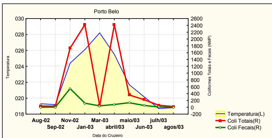
Figura 34a - Relação exibida entre os parâmetros Coliformes Totais e Fecais (NMP/100ml) e Temperatura Superficial da Água (°C), no ponto amostral “Porto Belo”, setor Centro-Norte, no período 2002-2003
