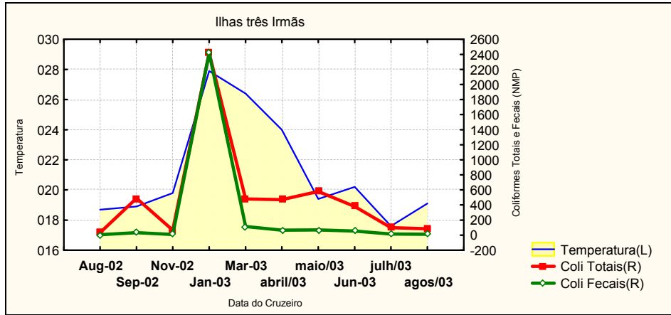
Figura 44a - Relação exibida entre os parâmetros Coliformes Totais e Fecais (NMP/100ml) e Temperatura Superficial da Água (°C), no ponto amostral “I. Três Irmãs”, setor Centro, no período 2002-2003
