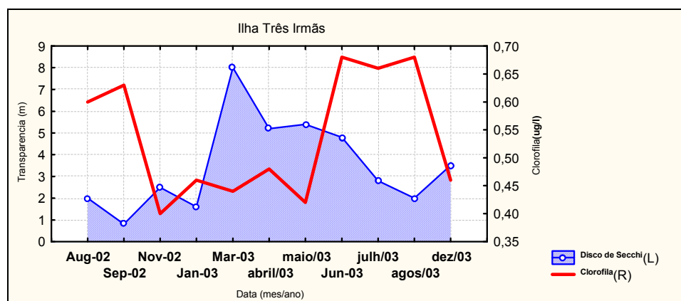
Figura 26i - Variação da concentração de clorofila “a” ( \mu\text{g/l} ) de superfície e da transparência (m) na coluna d’água entre 2002 e 2003, em “I. Três Irmãs”, do setor Centro do litoral de Santa Catarina
