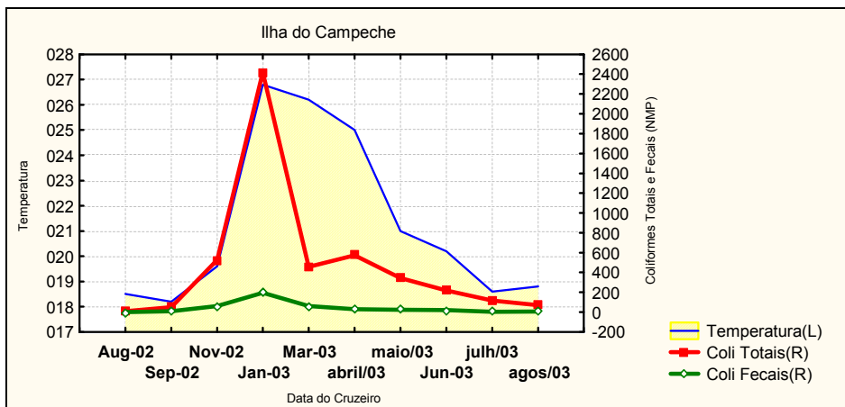
Figura 41a - Relação exibida entre os parâmetros Coliformes Totais e Fecais (NMP/100ml) e Temperatura Superficial da Água (°C), no ponto amostral "I. Campeche" (20 m), setor Centro, no período 2002-2003.
