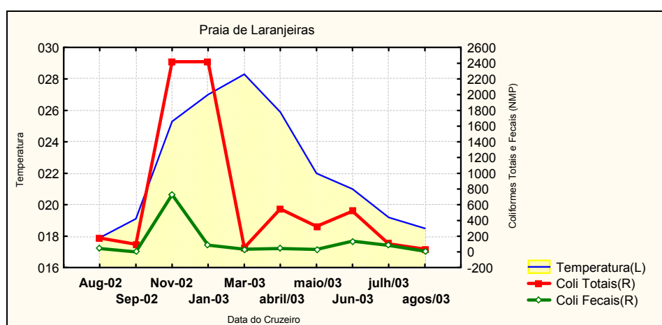
Figura 33a - Relação exibida entre os parâmetros Coliformes Totais e Fecais (NMP/100ml) e Temperatura Superficial da Água (°C), no ponto amostral “Laranjeiras”, setor Centro-Norte, no período 2002-2003
