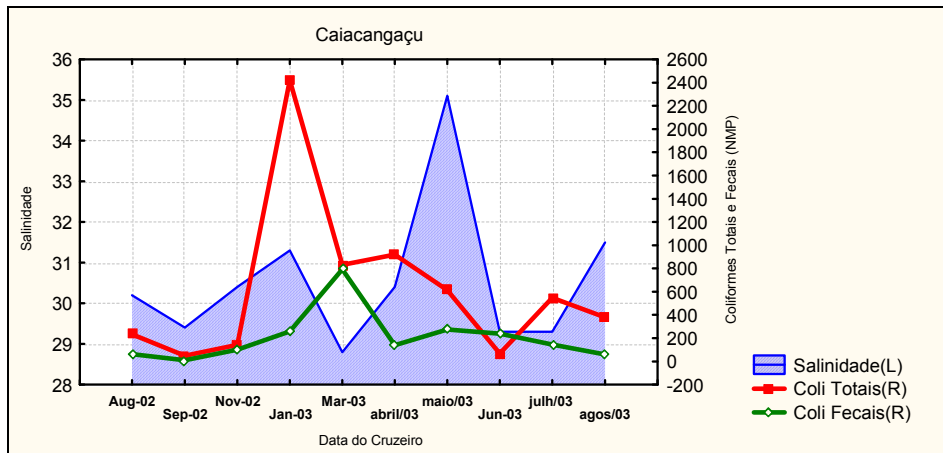
Figura 42b - Relação exibida entre os parâmetros Coliformes Totais e Fecais (NMP/100ml) e Salinidade (‰), no ponto amostral “Caiacangaçu”, setor Centro, no período 2002-2003
