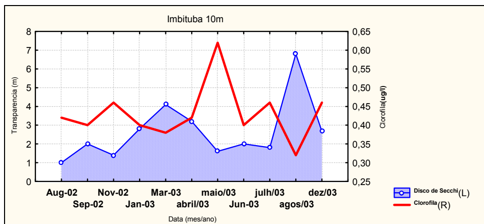
Figura 27f - Variação da concentração de clorofila "a" ( \mu\text{g/l} ) de superfície e da transparência (m) na coluna d'água entre 2002 e 2003, em "Imbituba" (10 m), do setor Centro-Sul do litoral de Santa Catarina
