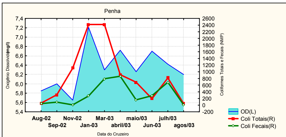
Figura 31c - Relação exibida entre os parâmetros Coliformes Totais e Fecais (NMP/100ml) e Oxigênio Dissolvido (mg/l), no ponto amostral “Penha” (5 m), setor Centro-Norte, no período 2002-2003
