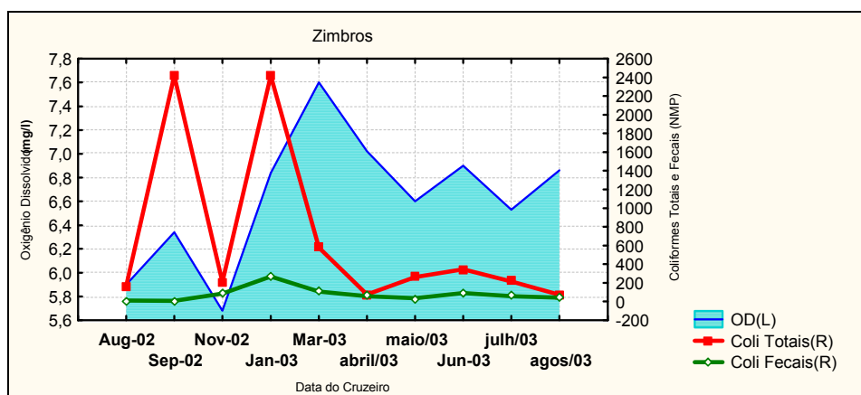
Figura 35c - Relação exibida entre os parâmetros Coliformes Totais e Fecais (NMP/100ml) e Oxigênio Dissolvido (mg/l), no ponto amostral “Zimbros”, setor Centro-Norte, no período 2002-2003
