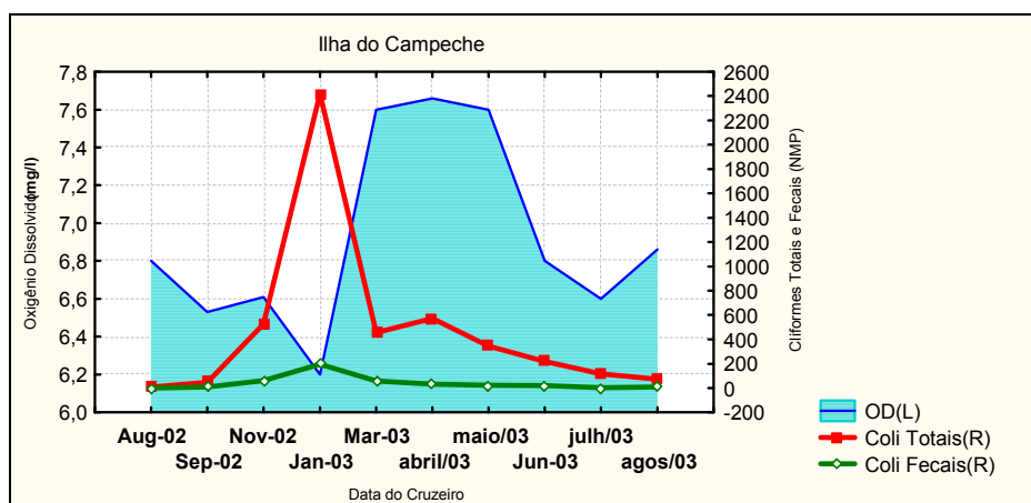
Figura 41c - Relação exibida entre os parâmetros Coliformes Totais e Fecais (NMP/100ml) e Oxigênio Dissolvido (mg/l), no ponto amostral "I. Campeche" (20 m), setor Centro, no período 2002-2003
