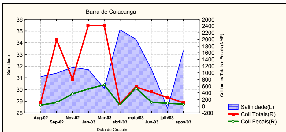
Figura 43b - Relação exibida entre os parâmetros Coliformes Totais e Fecais (NMP/100ml) e Salinidade (%), no ponto amostral "B. Caiacanga", setor Centro, no período 2002-2003
