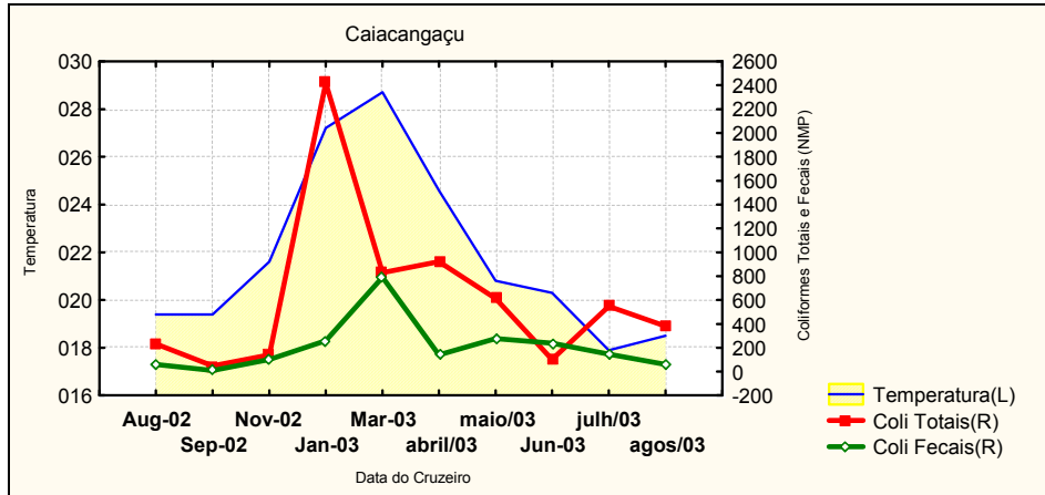
Figura 42a - Relação exibida entre os parâmetros Coliformes Totais e Fecais (NMP/100ml) e Temperatura Superficial da Água (°C), no ponto amostral “Caiacangaçu”, setor Centro, no período 2002-2003
