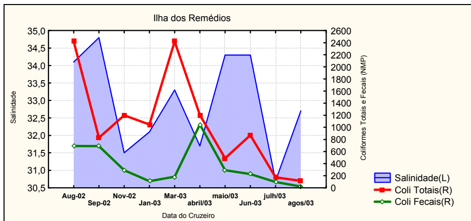
Figura 29b - Relação exibida entre os parâmetros Coliformes Totais e Fecais (NMP/100ml) e Salinidade (‰), no ponto amostral “Ilha dos Remédios”, setor Norte, no período 2002-2003
