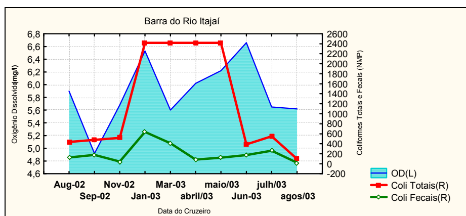
Figura 32c - Relação exibida entre os parâmetros Coliformes Totais e Fecais (NMP/100ml) e Oxigênio Dissolvido (mg/l), no ponto amostral “B. Itajaí-Açu”, setor Centro-Norte, no período 2002-2003
