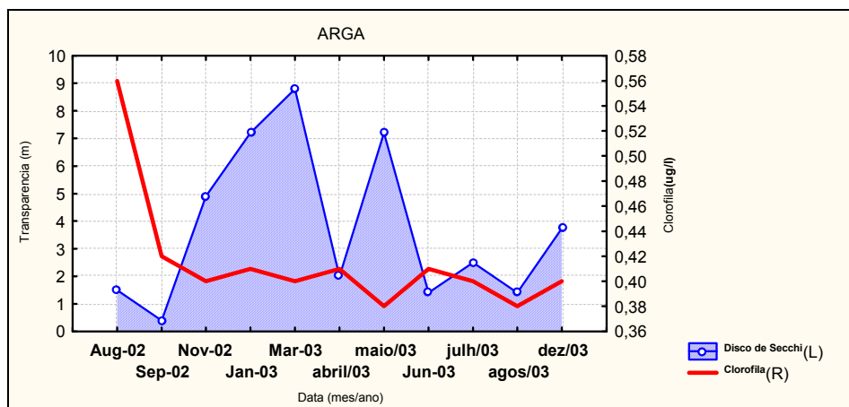
Figura 26b - Variação da concentração de clorofila "a" ( \mu\text{g/l} ) de superfície e da transparência (m) na coluna d'água entre 2002 e 2003, em "ARGA", do setor Centro do litoral de Santa Catarina
