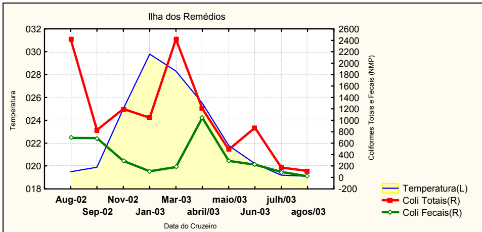
Figura 29a - Relação exibida entre os parâmetros Coliformes Totais e Fecais (NMP/100ml) e Temperatura Superficial da Água (°C), no ponto amostral “I. dos Remédios”, setor Norte, no período 2002-2003
