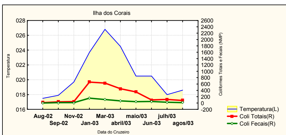
Figura 45a - Relação exibida entre os parâmetros Coliformes Totais e Fecais (NMP/100ml) e Temperatura Superficial da Água (°C), no ponto amostral “I. Corais”, setor Centro-Sul, no período 2002-2003
