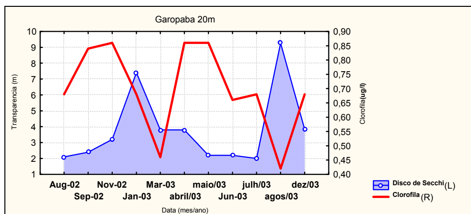
Figura 27d - Variação da concentração de clorofila "a" ( \mu\text{g/l} ) de superfície e da transparência (m) na coluna d'água entre 2002 e 2003, em "Garopaba" (20 m), do setor Centro-Sul do litoral de Santa Catarina
