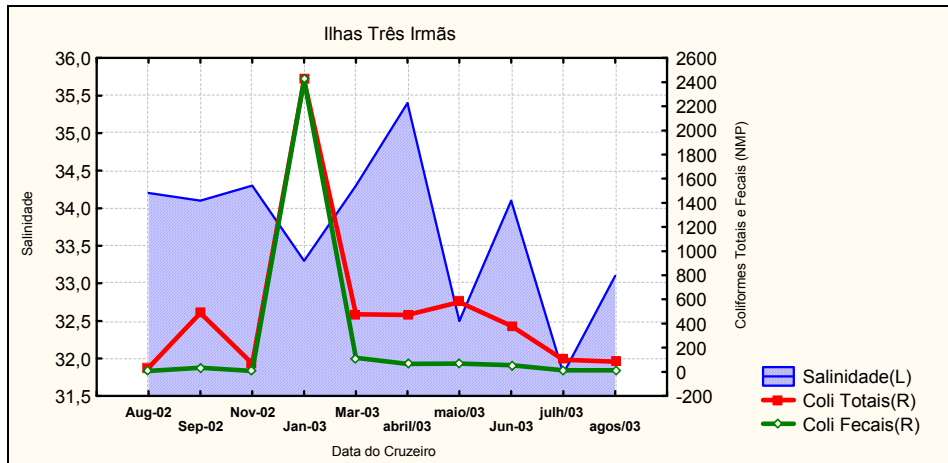
Figura 44b - Relação exibida entre os parâmetros Coliformes Totais e Fecais (NMP/100ml) e Salinidade (‰), no ponto amostral “I. Três Irmãs”, setor Centro, no período 2002-2003
