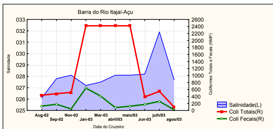
Figura 32b - Relação exibida entre os parâmetros Coliformes Totais e Fecais (NMP/100ml) e Salinidade (‰), no ponto amostral “B. Itajaí-Açu”, setor Centro-Norte, no período 2002-2003
