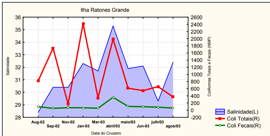
Figura 40b - Relação exibida entre os parâmetros Coliformes Totais e Fecais (NMP/100ml) e Salinidade (‰), no ponto amostral "I. Ratores Grande", setor Centro, no período 2002-2003
