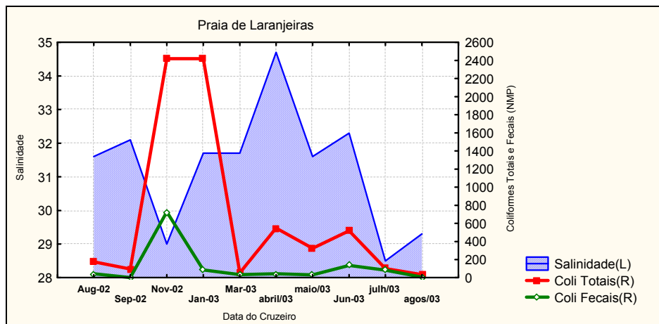
Figura 33b - Relação exibida entre os parâmetros Coliformes Totais e Fecais (NMP/100ml) e Salinidade (‰), no ponto amostral “Laranjeiras”, setor Centro-Norte, no período 2002-2003
