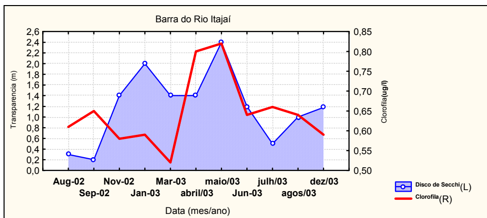
Figura 25d - Variação da concentração de clorofila "a" ( \mu\text{g/l} ) de superfície e da transparência (m) na coluna d'água entre 2002 e 2003, em "Barra Itajaí-Açú", do setor Centro-Norte do litoral de Santa Catarina
