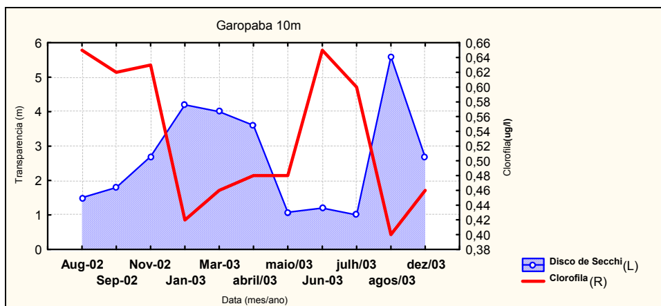
Figura 27c - Variação da concentração de clorofila "a" ( \mu\text{g/l} ) de superfície e da transparência (m) na coluna d'água entre 2002 e 2003, em "Garopaba" (10 m), do setor Centro-Sul do litoral de Santa Catarina
