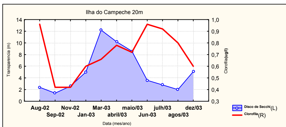
Figura 26f - Variação da concentração de clorofila "a" ( \mu\text{g/l} ) de superfície e da transparência (m) na coluna d'água entre 2002 e 2003, em "I. Campeche" (20 m), do setor Centro do litoral de Santa Catarina
