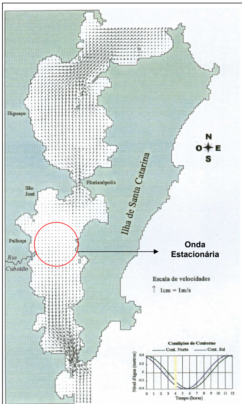
Figura 65 - Velocidade média induzida pela onda de maré M2, na Baía de Florianópolis, 04 horas após a maré alta, junto a barra de saída na Baía Sul Fonte: LAHIMAR/UFSC
