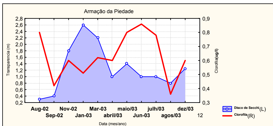
Figura 26c - Variação da concentração de clorofila "a" ( \mu\text{g/l} ) de superfície e da transparência (m) na coluna d'água entre 2002 e 2003, em "A. Piedade", do setor Centro do litoral de Santa Catarina
