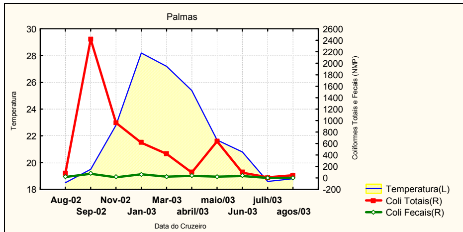
Figura 38a - Relação exibida entre os parâmetros Coliformes Totais e Fecais (NMP/100ml) e Temperatura Superficial da Água (°C), no ponto amostral “Palmas”, setor Centro, no período 2002-2003
