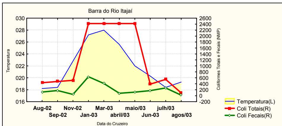
Figura 32a - Relação exibida entre os parâmetros Coliformes Totais e Fecais (NMP/100ml) e Temperatura Superficial da Água (°C), no ponto amostral “B. Itajaí-Açú”, setor Centro-Norte, no período 2002-2003
