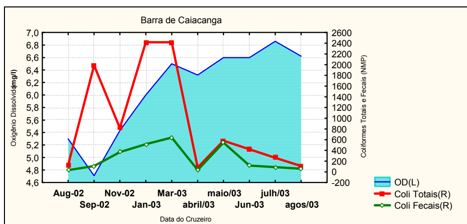
Figura 43c - Relação exibida entre os parâmetros Coliformes Totais e Fecais (NMP/100ml) e Oxigênio Dissolvido (mg/l), no ponto amostral "B. Caiacanga", setor Centro, no período 2002-2003
