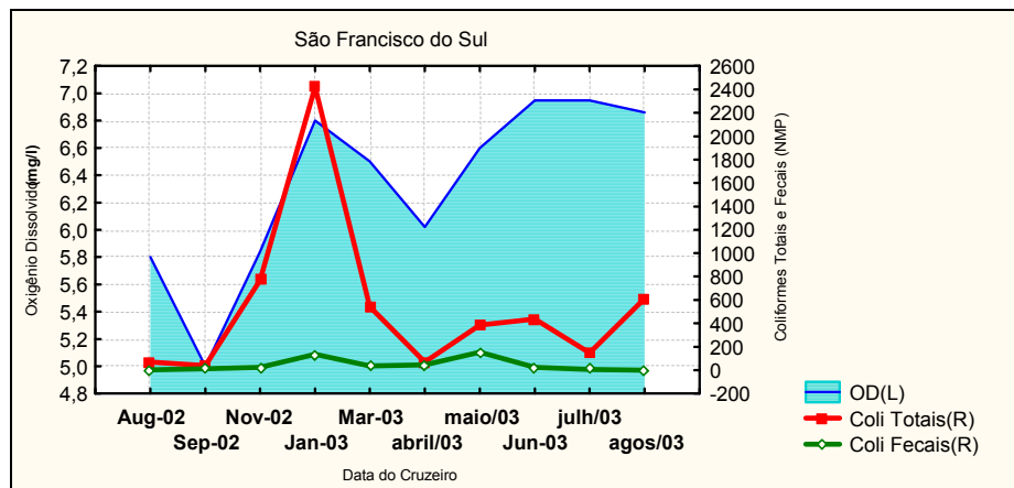
Figura 30c - Relação exibida entre os parâmetros Coliformes Totais e Fecais (NMP/100ml) e Oxigênio Dissolvido (mg/l), no ponto amostral “S. Francisco”, setor Norte, no período 2002-2003
