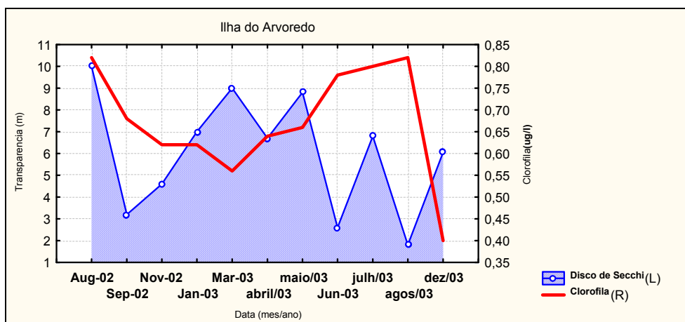
Figura 25h - Variação da concentração de clorofila "a" ( \mu\text{g/l} ) de superfície e da transparência (m) na coluna d'água entre 2002 e 2003, em "Ilha do Arvoredo", do setor Centro-Norte do litoral de Santa Catarina
