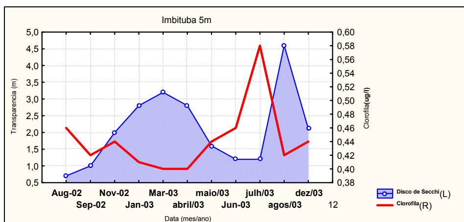
Figura 27e - Variação da concentração de clorofila "a" ( \mu\text{g/l} ) de superfície e da transparência (m) na coluna d'água entre 2002 e 2003, em "Imbituba" (5 m), do setor Centro-Sul do litoral de Santa Catarina
