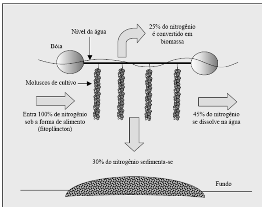
Figura 3 - Balanço do nitrogênio de origem orgânica num cultivo de mexilhões Fonte: Folke e Kautsky (1989 apud ARANA, 2000)
