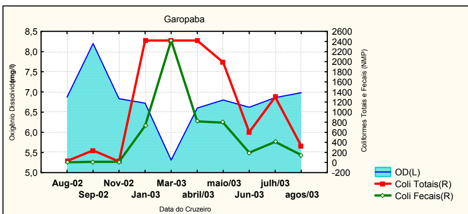
Figura 46c - Relação exibida entre os parâmetros Coliformes Totais e Fecais (NMP/100ml) e Oxigênio Dissolvido (mg/l), no ponto amostral "Garopaba" (5 m), setor Centro-Sul, no período 2002-2003
