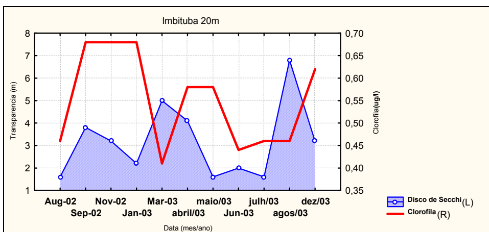
Figura 27g - Variação da concentração de clorofila "a" ( \mu\text{g/l} ) de superfície e da transparência (m) na coluna d'água entre 2002 e 2003, em "Imbituba" (20 m), do setor Centro-Sul do litoral de Santa Catarina
