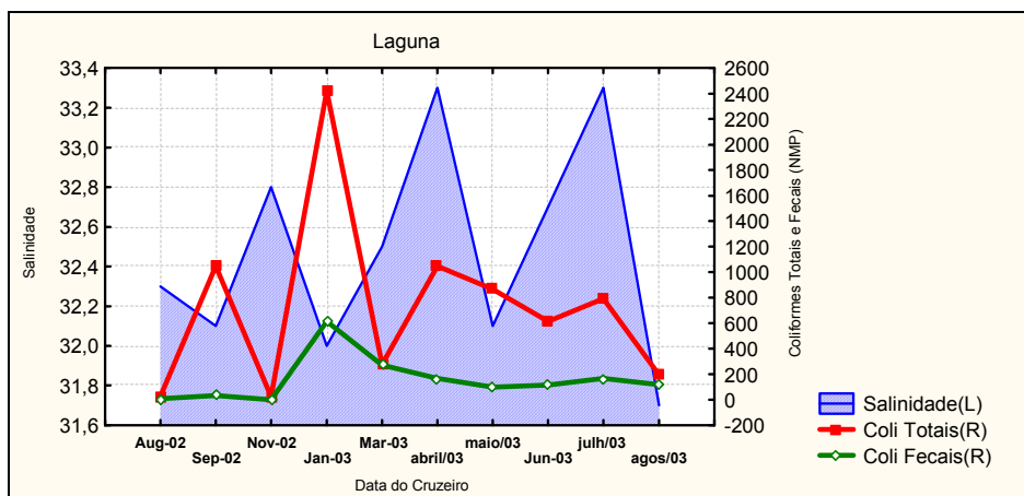
Figura 48b - Relação exibida entre os parâmetros Coliformes Totais e Fecais (NMP/100ml) e Salinidade (‰), no ponto amostral “Laguna”, setor Centro-Sul, no período 2002-2003
