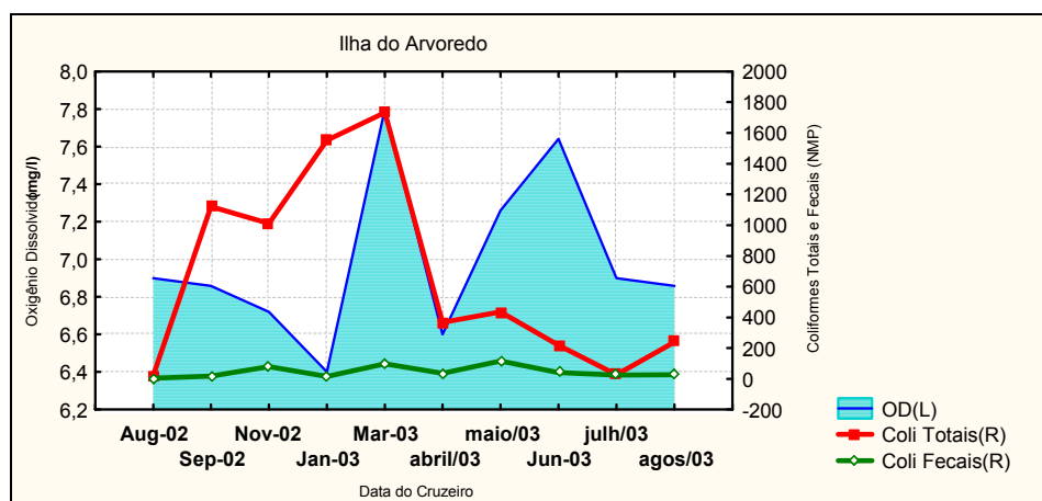
Figura 36c - Relação exibida entre os parâmetros Coliformes Totais e Fecais (NMP/100ml) e Oxigênio Dissolvido (mg/l), no ponto amostral “I. Arvoredo”, setor Centro-Norte, no período 2002-2003
