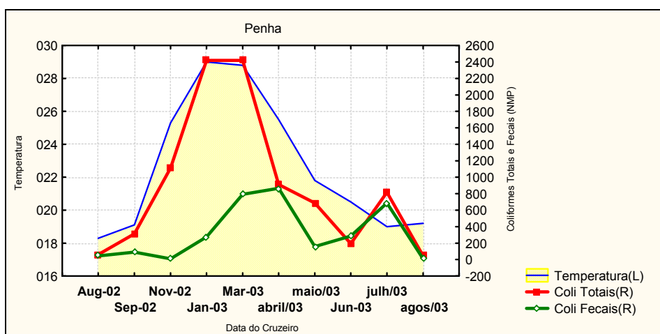
Figura 31a - Relação exibida entre os parâmetros Coliformes Totais e Fecais (NMP/100ml) e Temperatura Superficial da Água (°C), no ponto amostral “Penha” (5 m), setor Centro-Norte, no período 2002-2003
