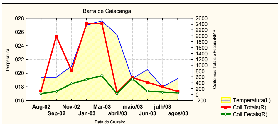
Figura 43a - Relação exibida entre os parâmetros Coliformes Totais e Fecais (NMP/100ml) e Temperatura Superficial da Água (°C), no ponto amostral "B. Caiacanga", setor Centro, no período 2002-2003
