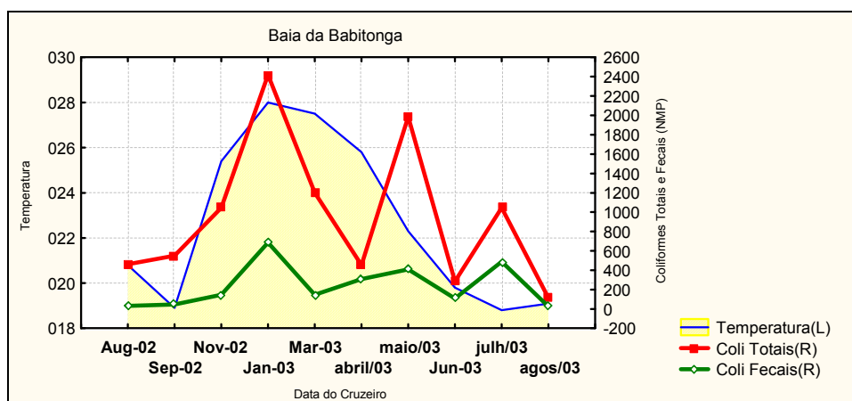
Figura 28a - Relação exibida entre os parâmetros Coliformes Totais e Fecais (NMP/100ml) e Temperatura Superficial da Água (°C), no ponto amostral "Baía da Babitonga", setor Norte, no período 2002-2003
