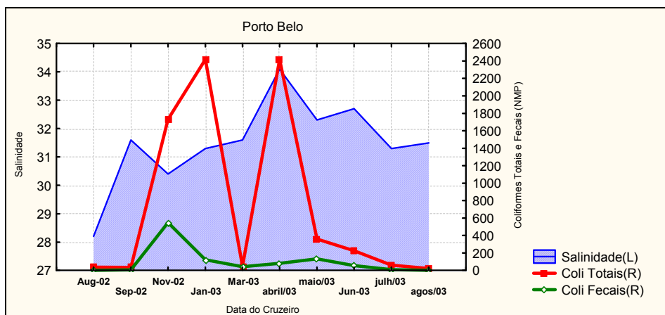
Figura 34b - Relação exibida entre os parâmetros Coliformes Totais e Fecais (NMP/100ml) e Salinidade (%), no ponto amostral “Porto Belo”, setor Centro-Norte, no período 2002-2003
