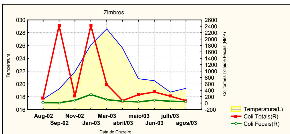
Figura 35a - Relação exibida entre os parâmetros Coliformes Totais e Fecais (NMP/100ml) e Temperatura Superficial da Água (°C), no ponto amostral “Zimbros”, setor Centro-Norte, no período 2002-2003
