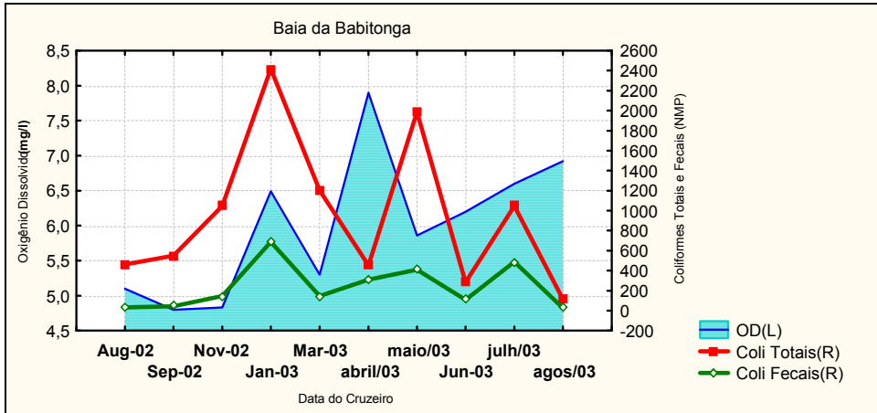
Figura 28c - Relação exibida entre os parâmetros Coliformes Totais e Fecais (NMP/100ml) e Oxigênio Dissolvido (mg/l), no ponto amostral “Baía da Babitonga”, setor Norte, no período 2002-2003
