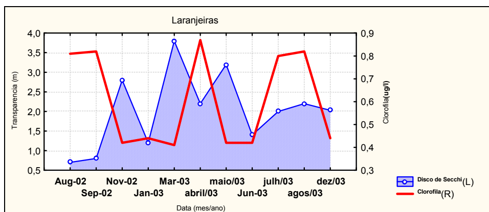
Figura 25e - Variação da concentração de clorofila "a" ( \mu\text{g/l} ) de superfície e da transparência (m) na coluna d'água entre 2002 e 2003, em "Laranjeiras", do setor Centro-Norte do litoral de Santa Catarina
