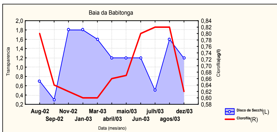
Figura 24a - Variação da concentração de clorofila “a” ( \mu\text{g/l} ) e de transparência da coluna d’água (m) entre 2002 e 2003, no ponto amostral “Baía da Babitonga”, setor Norte do litoral de Santa Catarina
