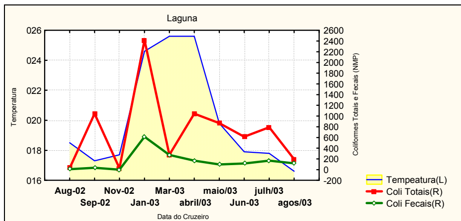
Figura 48a - Relação exibida entre os parâmetros Coliformes Totais e Fecais (NMP/100ml) e Temperatura Superficial da Água (°C), no ponto amostral "Laguna", setor Centro-Sul, no período 2002-2003
