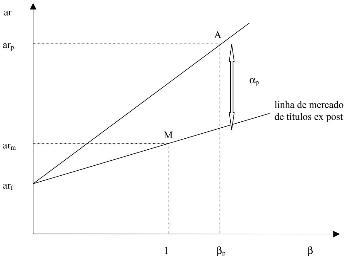
Figura 3 – Alfa de Jensen para o fundo A
