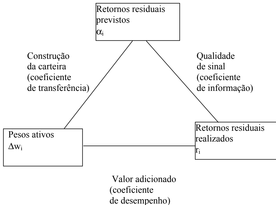
Figura 2 – O triângulo de correlação
