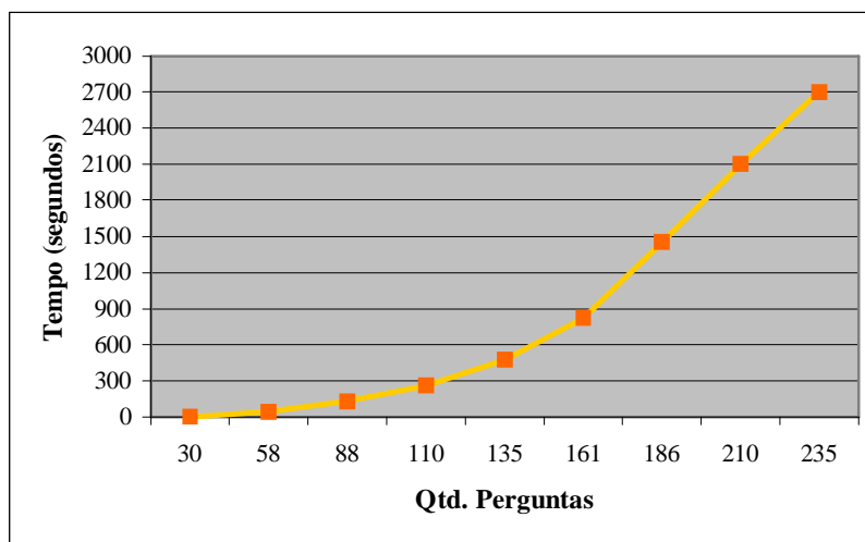
Figura 6.6 - Gráfico demonstrativo do Tempo de Gravação x Quantidade de Perguntas
