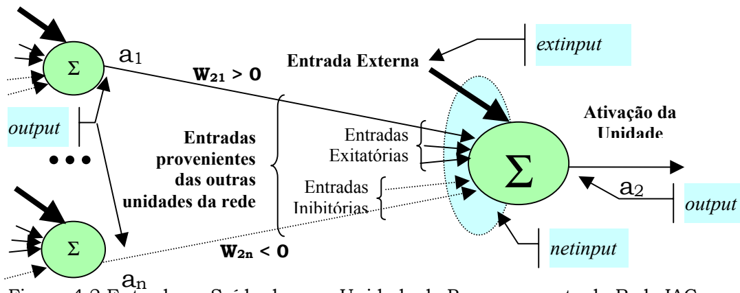
Figura 4.2 Entradas e Saída de uma Unidade de Processamento da Rede IAC
