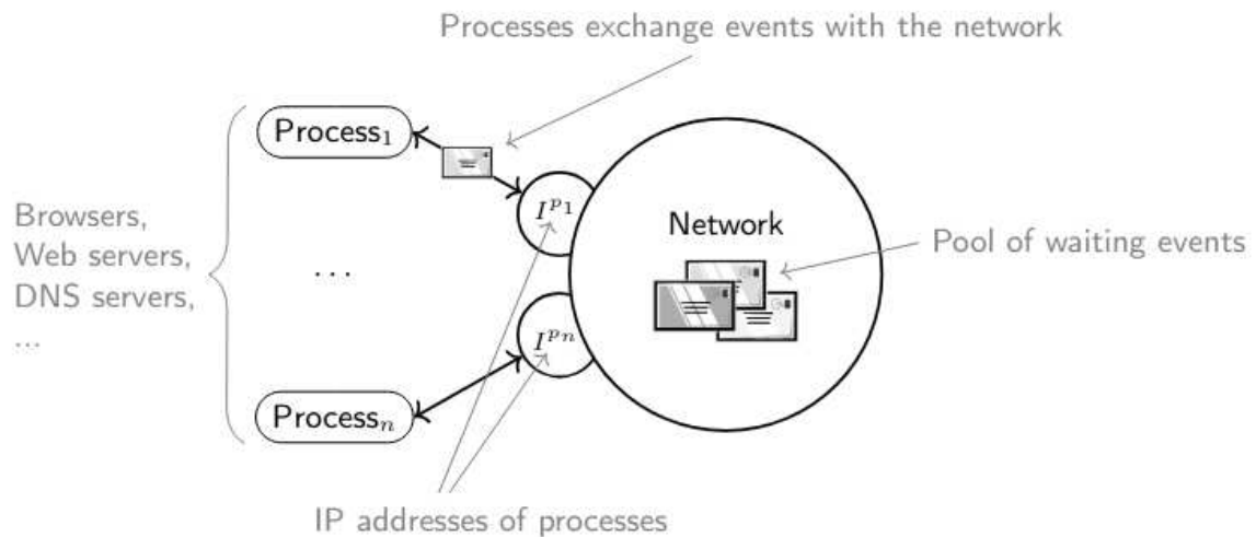
Figura 10 – Modelo WIM.
