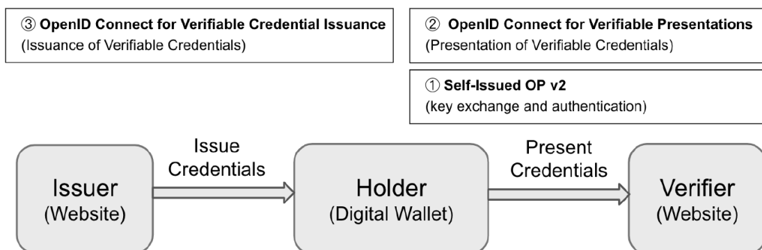
Figura 7 – Ecosystema do OIDC4VC.
