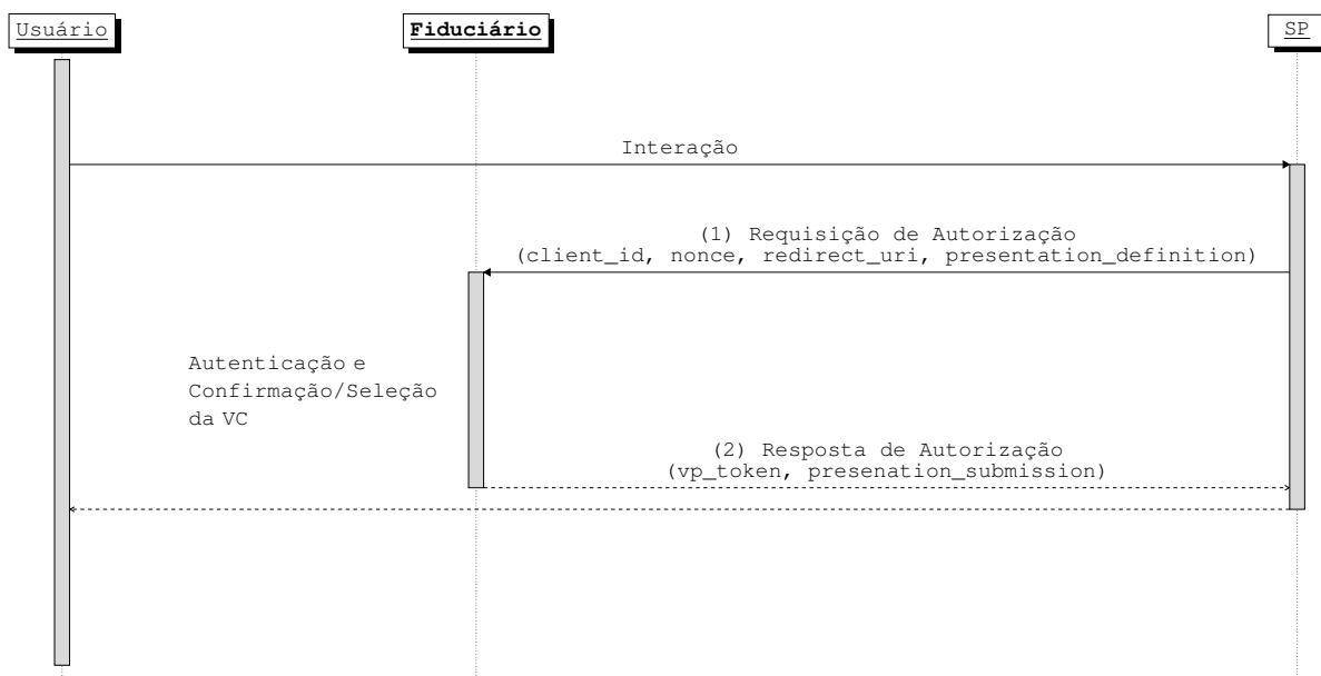
Figura 14 – Fluxo com Fiduciário no lugar da Carteira.
