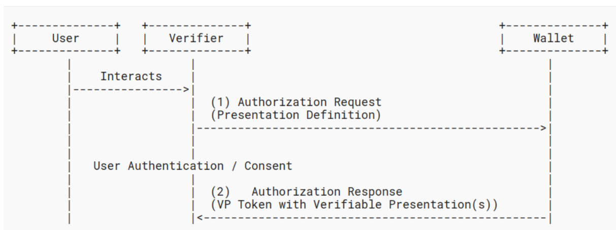
Figura 8 – Fluxo com Carteira e SP no mesmo dispositivo.
