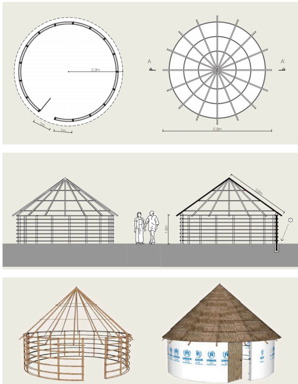
Figura 17: Dimensões e estrutura do Tukul. Fonte: adaptado de UNHCR (2016).
