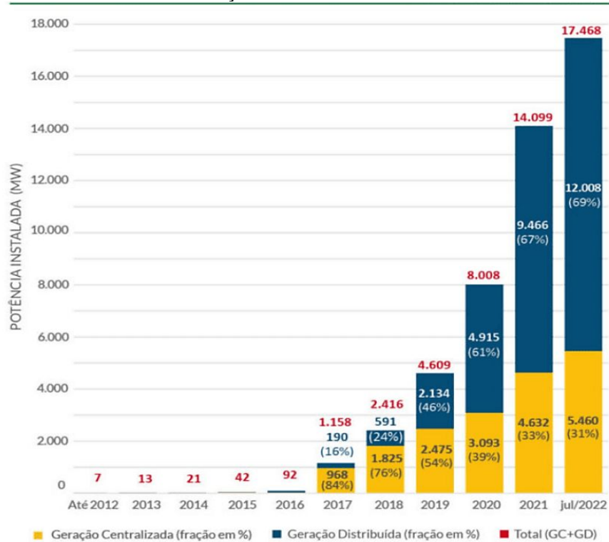
FIGURA 3 – Evolução da fonte solar fotovoltaica no Brasil
