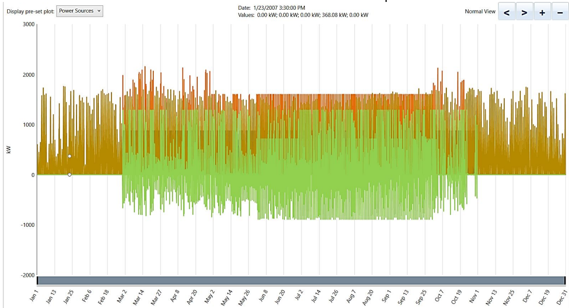
FIGURA 17 – Funcionamento Anual da Microrrede para a Fazenda B
