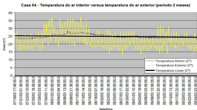
Figura 30: Temperaturas Casa 54. Fonte: AlmaVerde.
