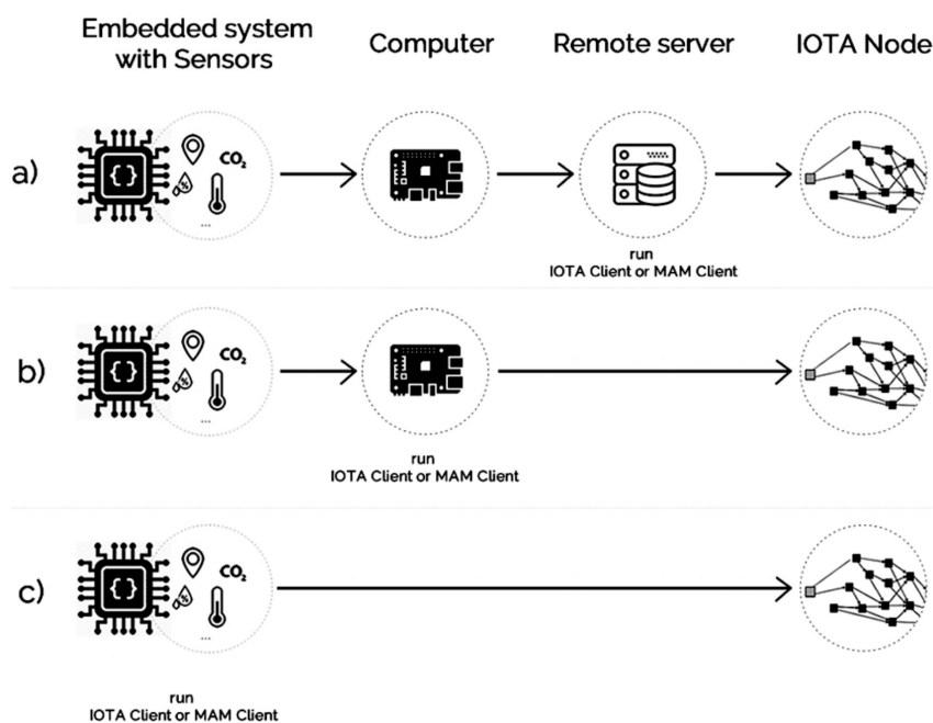
Figura 6 – Arquiteturas de rede possíveis para publicar dados de sensores no Tangle
