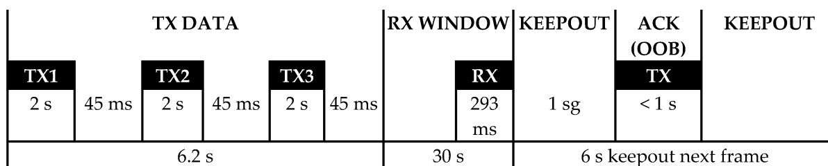
Figura 11 – Cronologia de uma comunicação Sigfox
