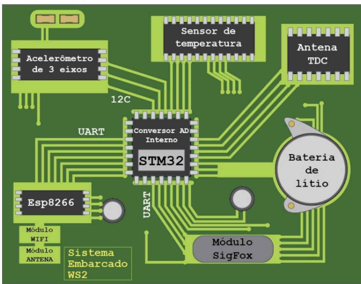
Figura 26 – WACS 2: ilustração dos componentes
