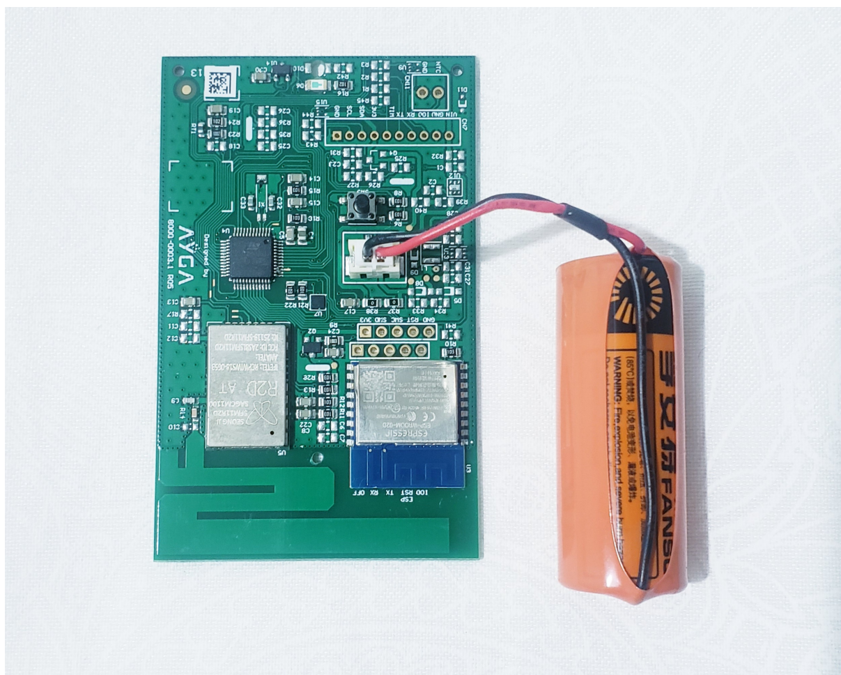
Figura 27 – WACS 2: foto real
