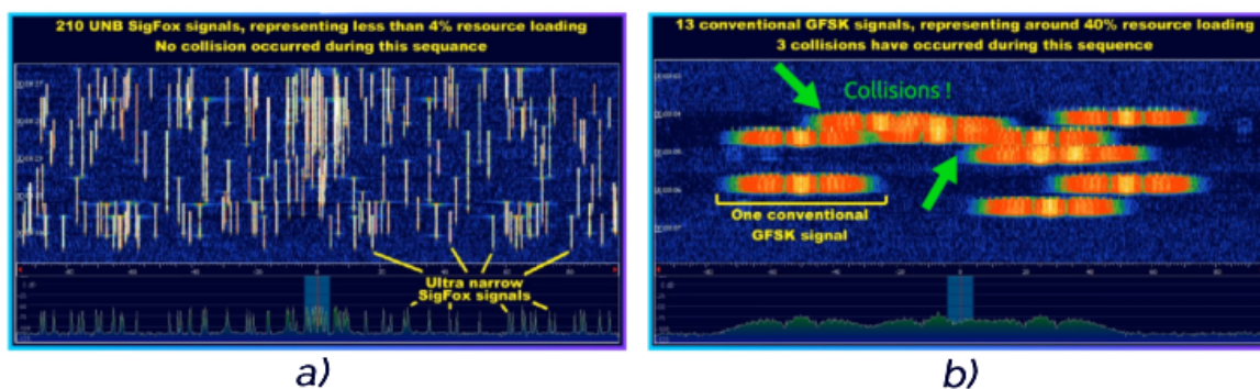
Figura 10 – Comparação de sinais Sigfox x 3G
