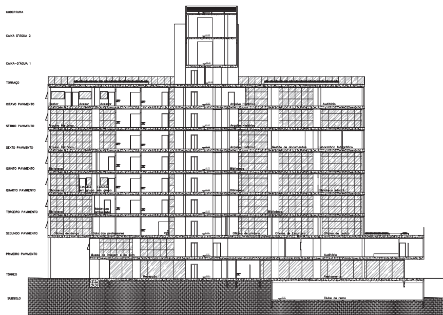
CORTE BB ESCALA 1:200
