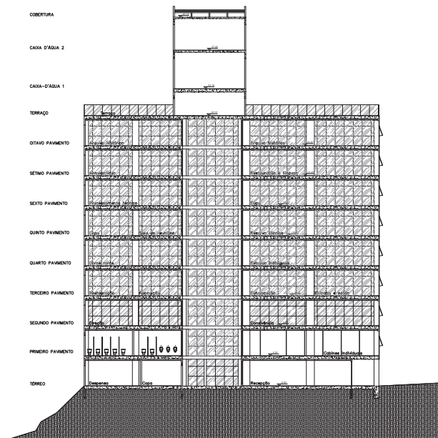
CORTE DD ESCALA 1:200
