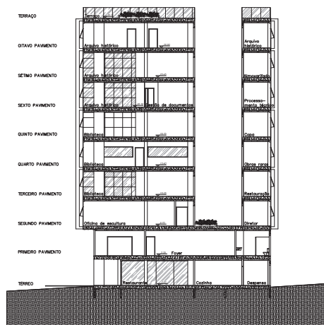
CORTE CC ESCALA 1:200
