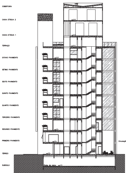
CORTE AA ESCALA 1:200
