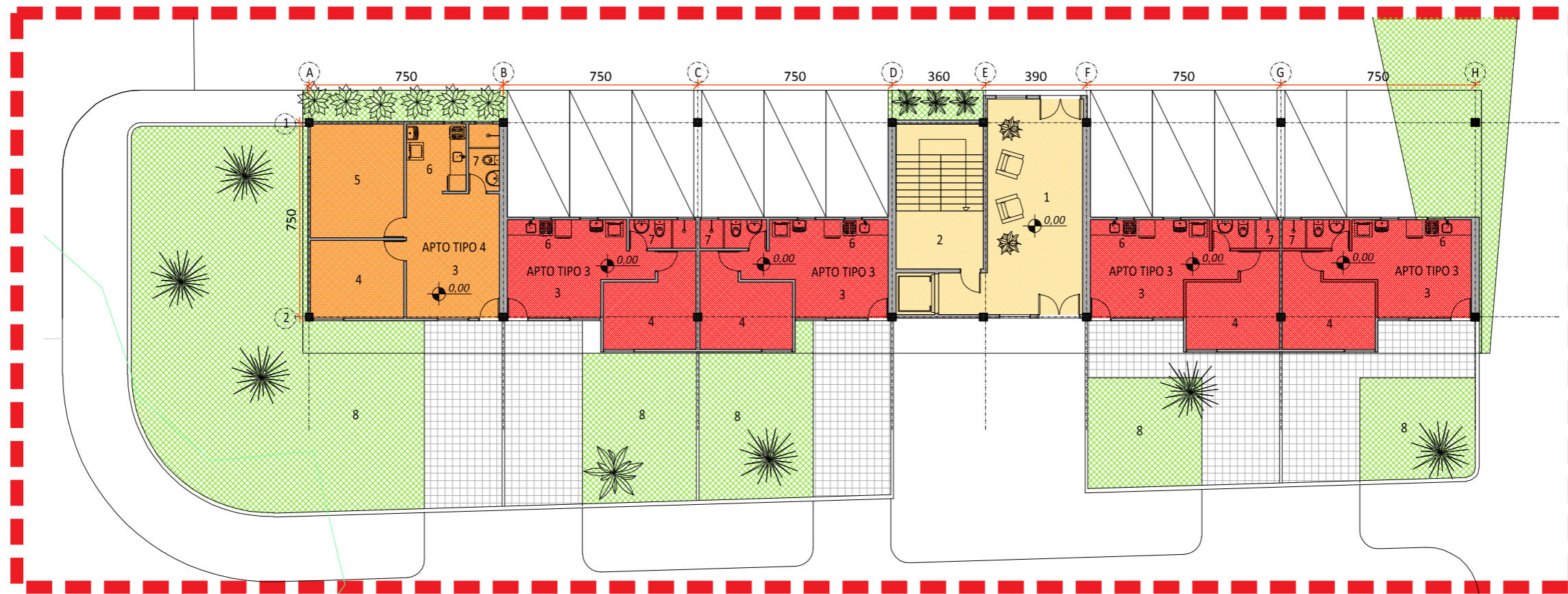
TÉRREO TIPO 2 esc.: 1:200
