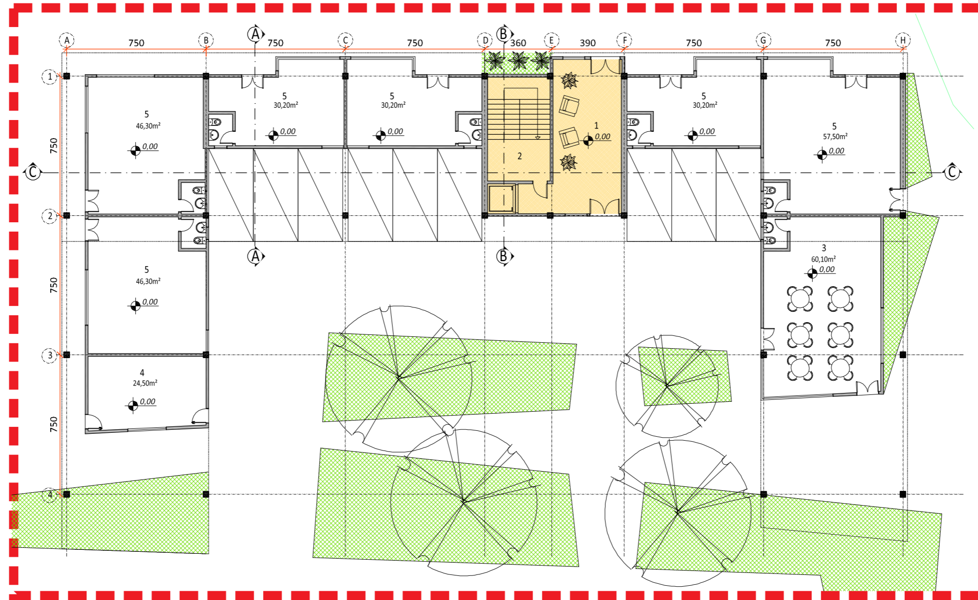
TÉRREO TIPO 1 esc.: 1:200
