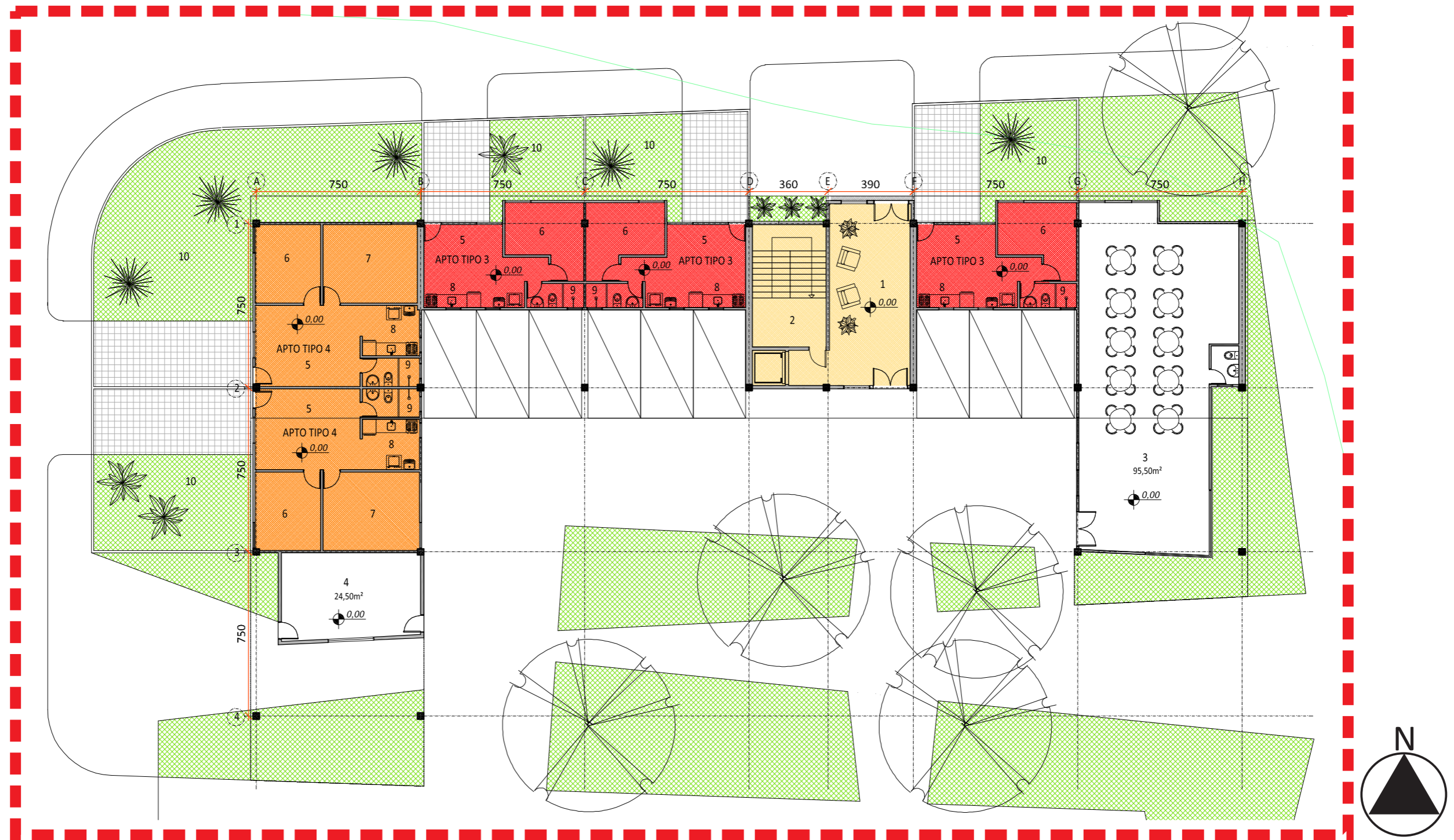
TÉRREO TIPO 4 esc.: 1:200
