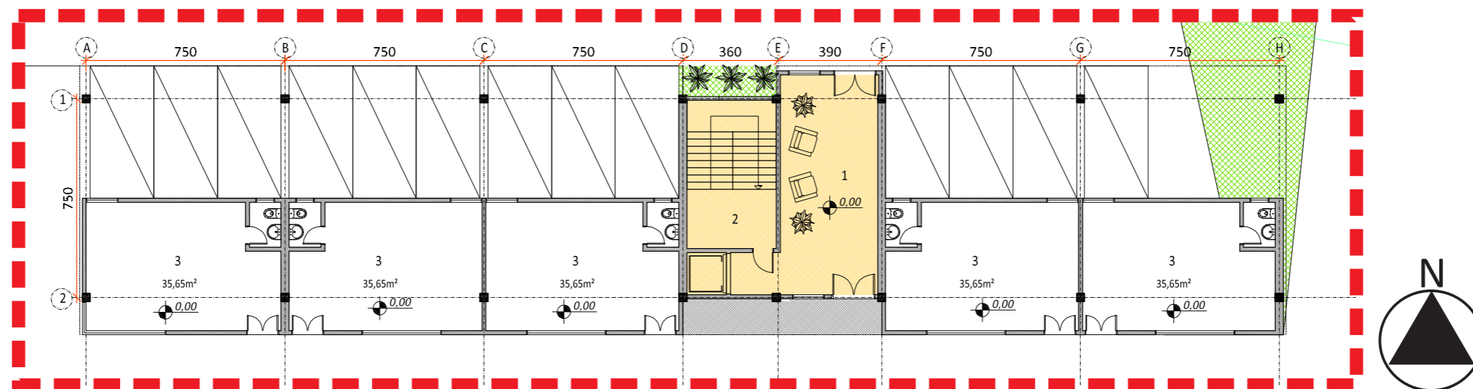
TÉRREO TIPO 3 esc.: 1:200
