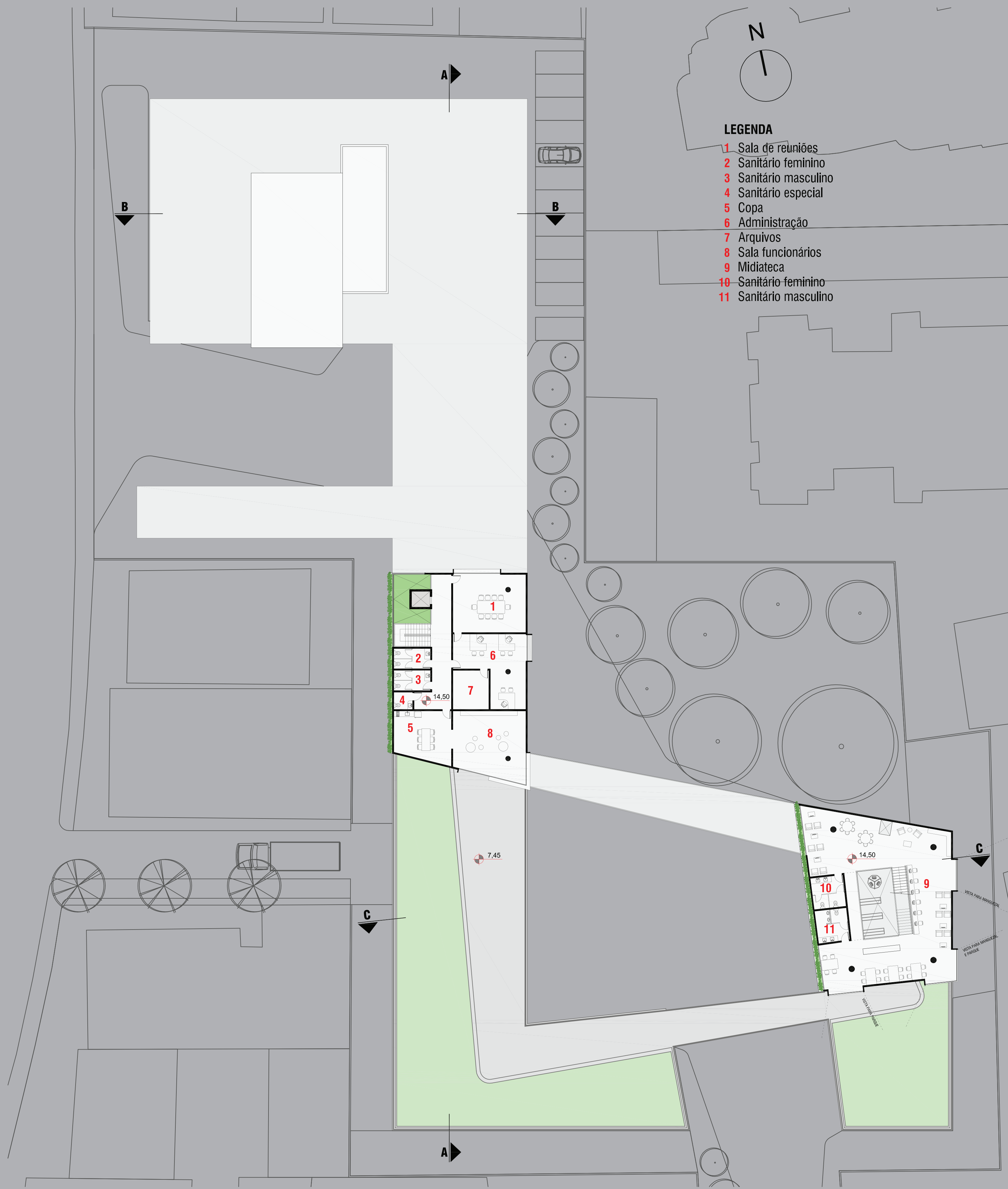
10 | PLANTA BAIXA - 4º PAVTO ESC 1:250
