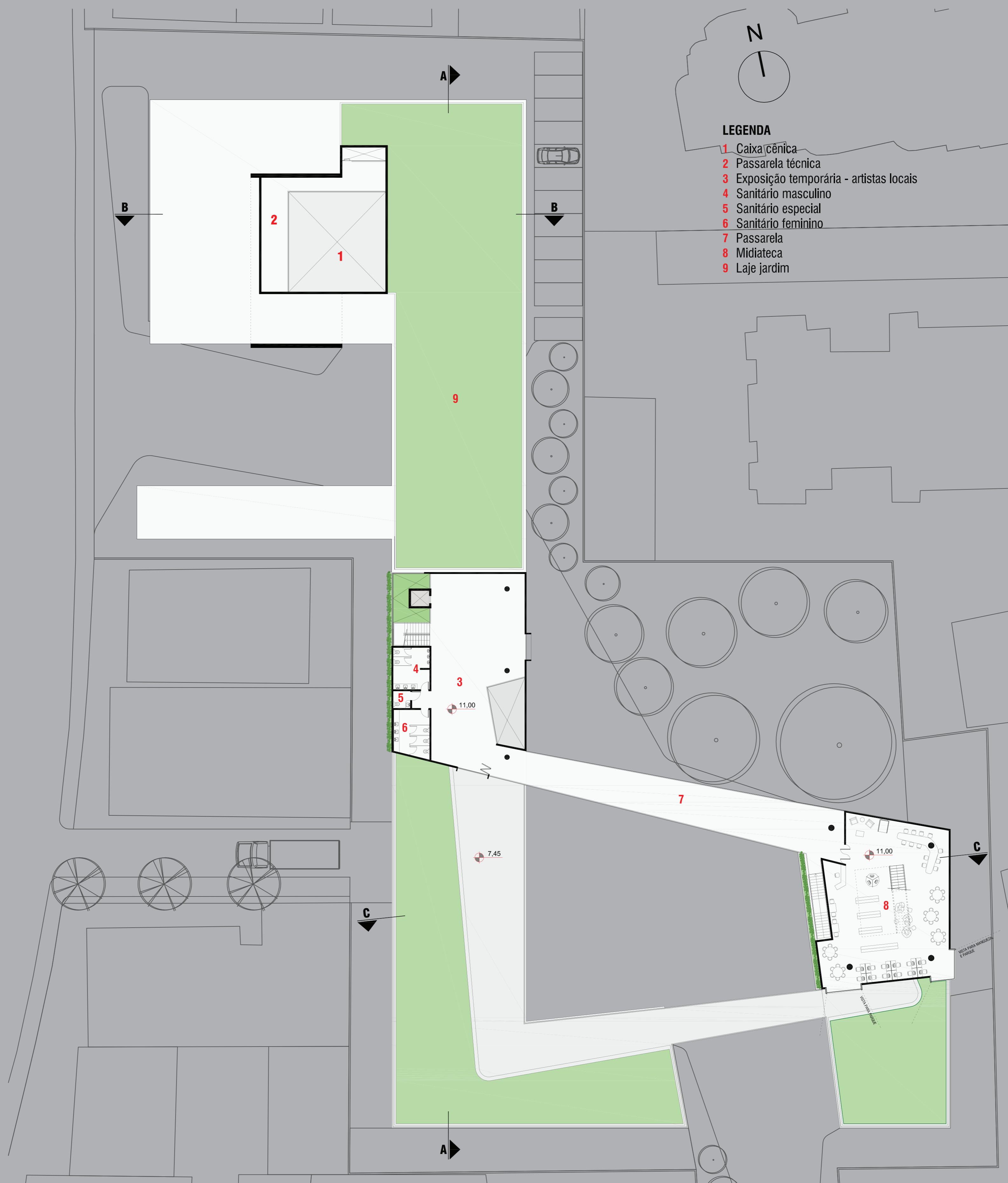
09 | PLANTA BAIXA - 3º PAVTO ESC 1:250
