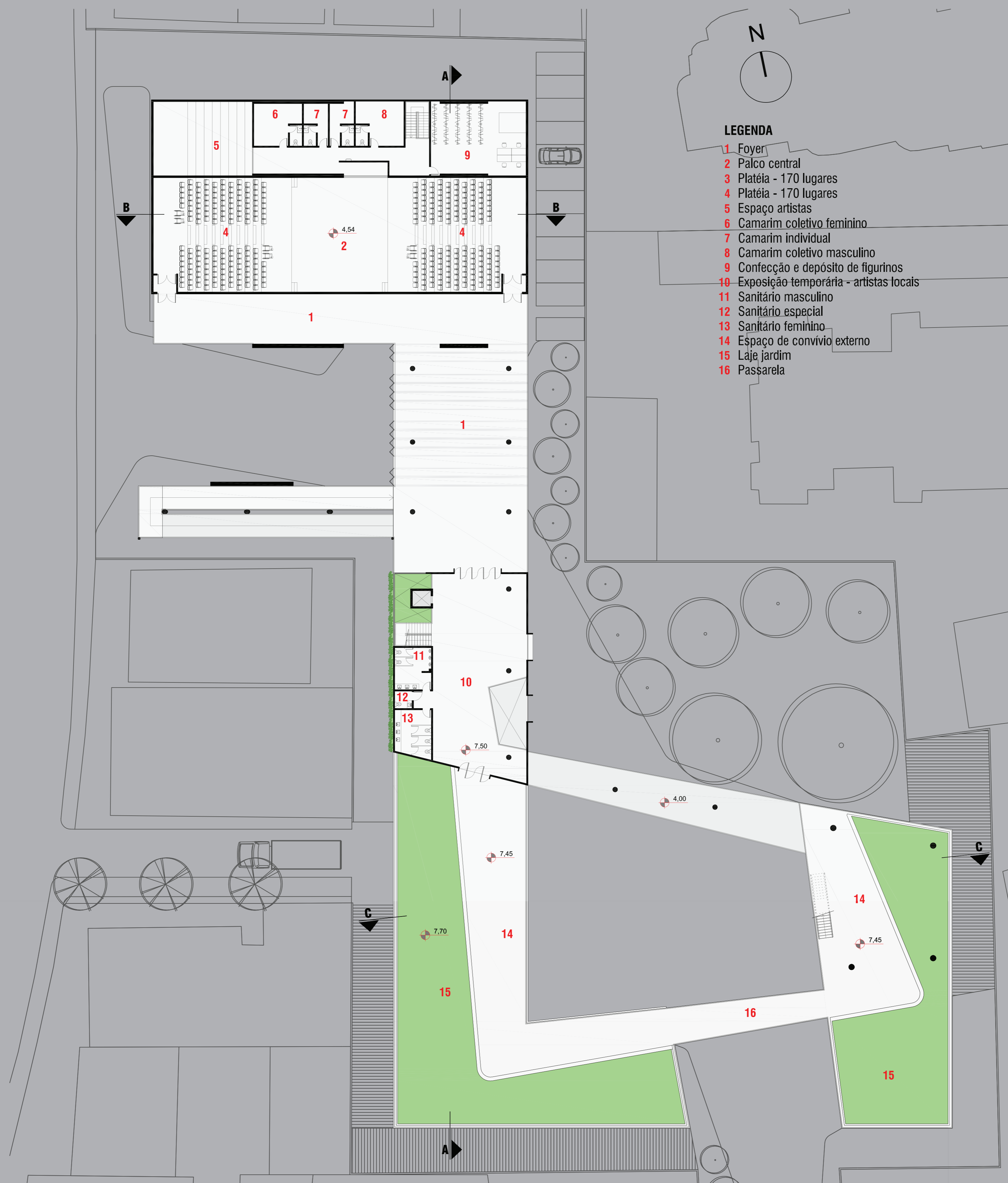
08 | PLANTA BAIXA - 2º PAVTO ESC 1:250
