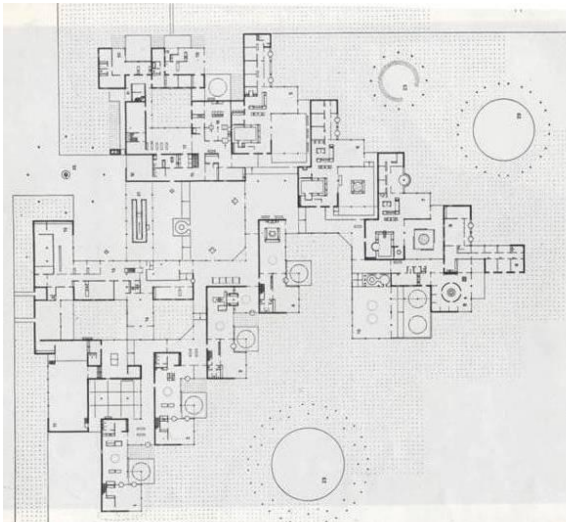
Planta Baixa
