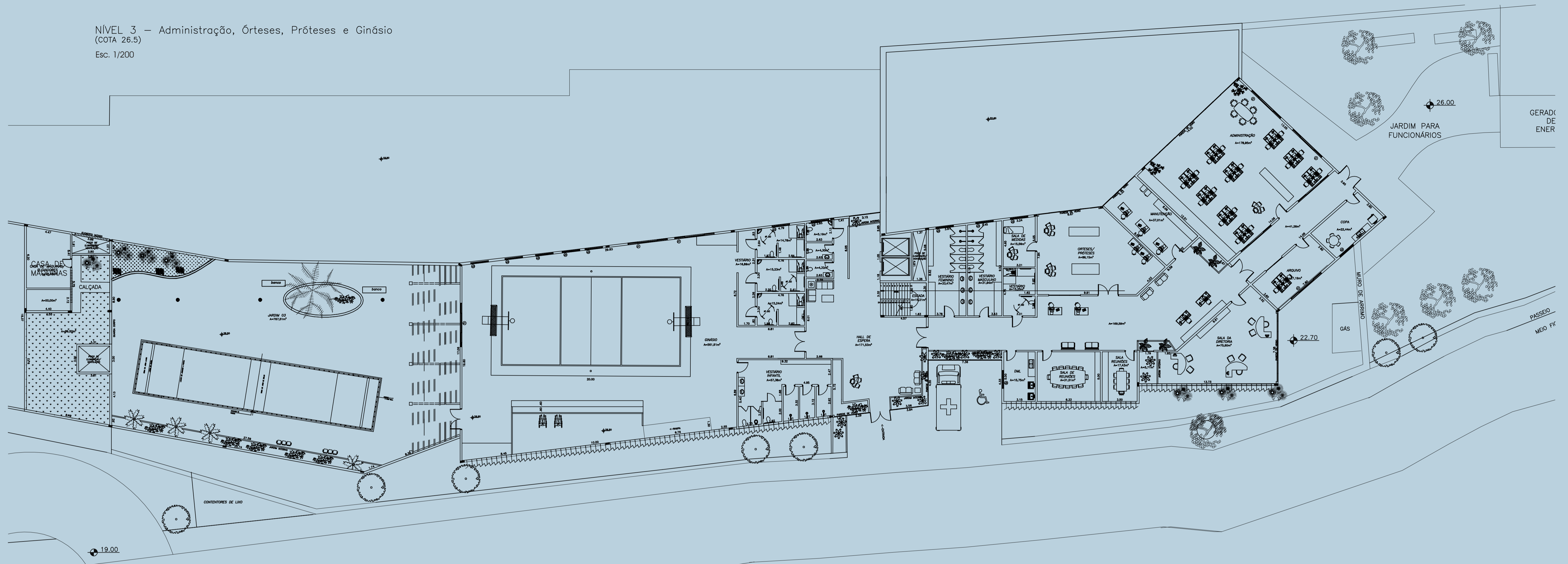
NÍVEL 4 – Biblioteca, Auditório e Administração (COTA 30.5) Esc. 1/200
