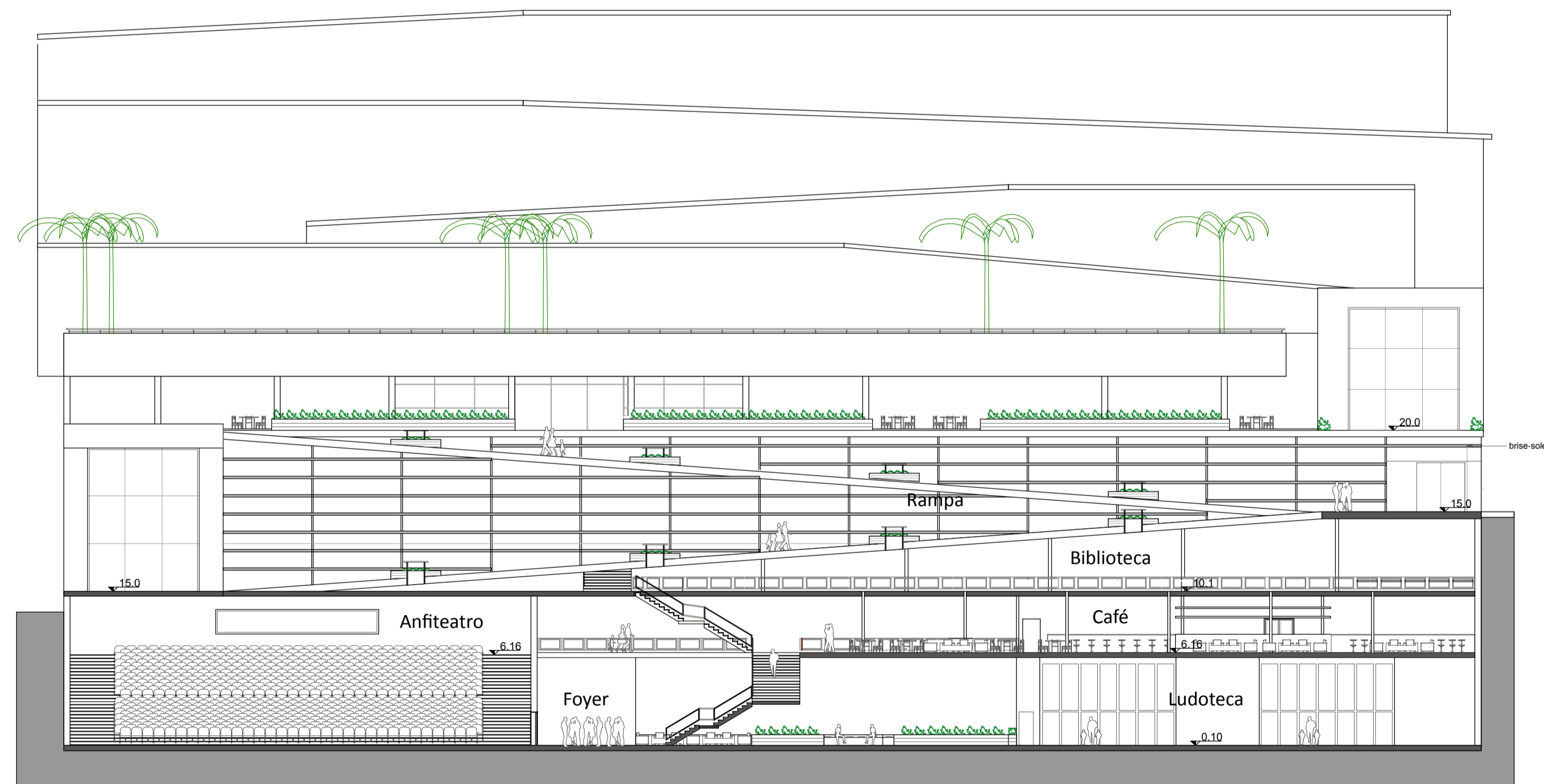
CORTE TRANSVERSAL CC ESCALA _____ 1/250
