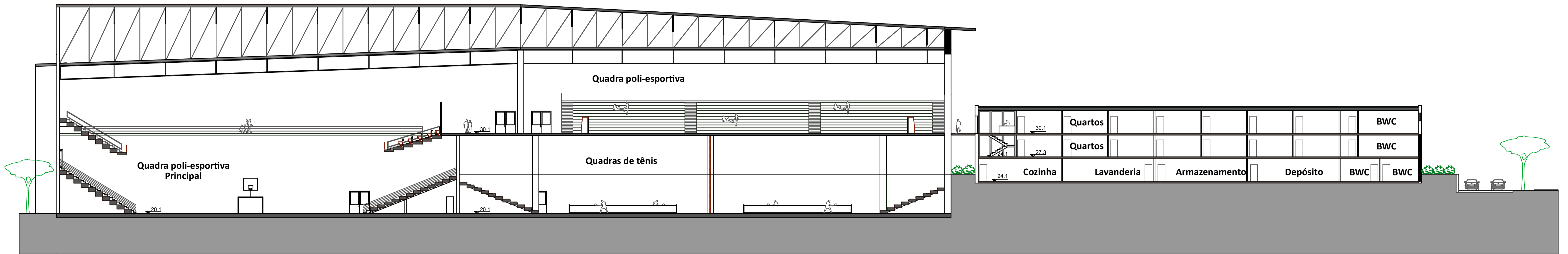
CORTE TRANSVERSAL BB ESCALA _____ 1/250
