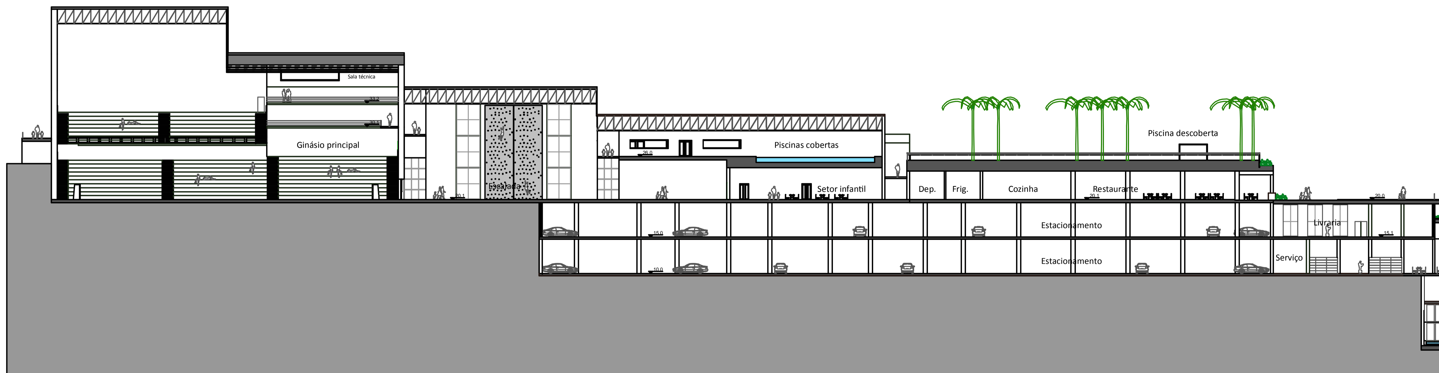
CORTE LONGITUDINAL AA ESCALA _____ 1/250
