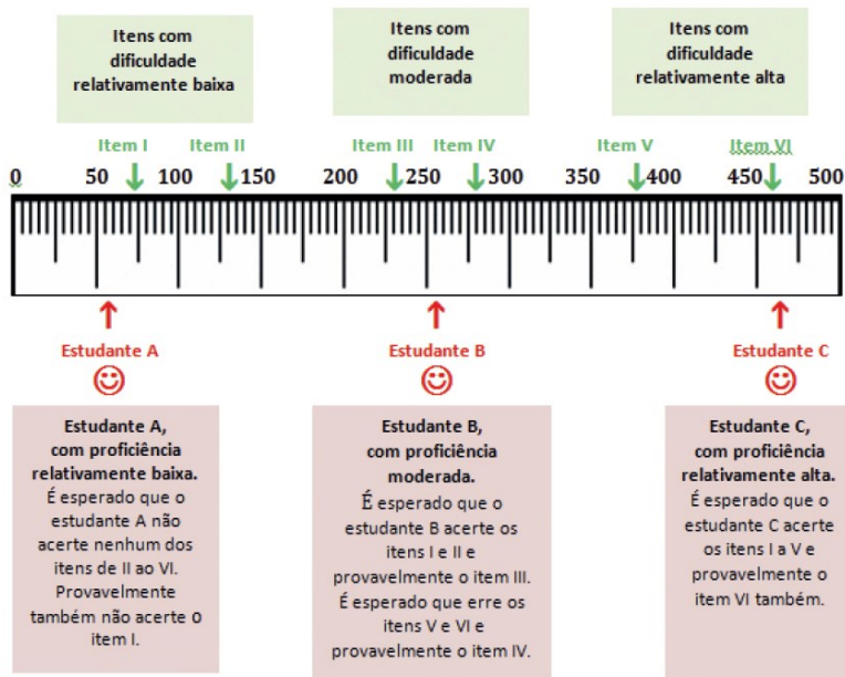
Figura 3 - Representação de uma escala de proficiência hipotética, mostrando as relações entre a posição dos itens e das proficiências dos estudantes.
