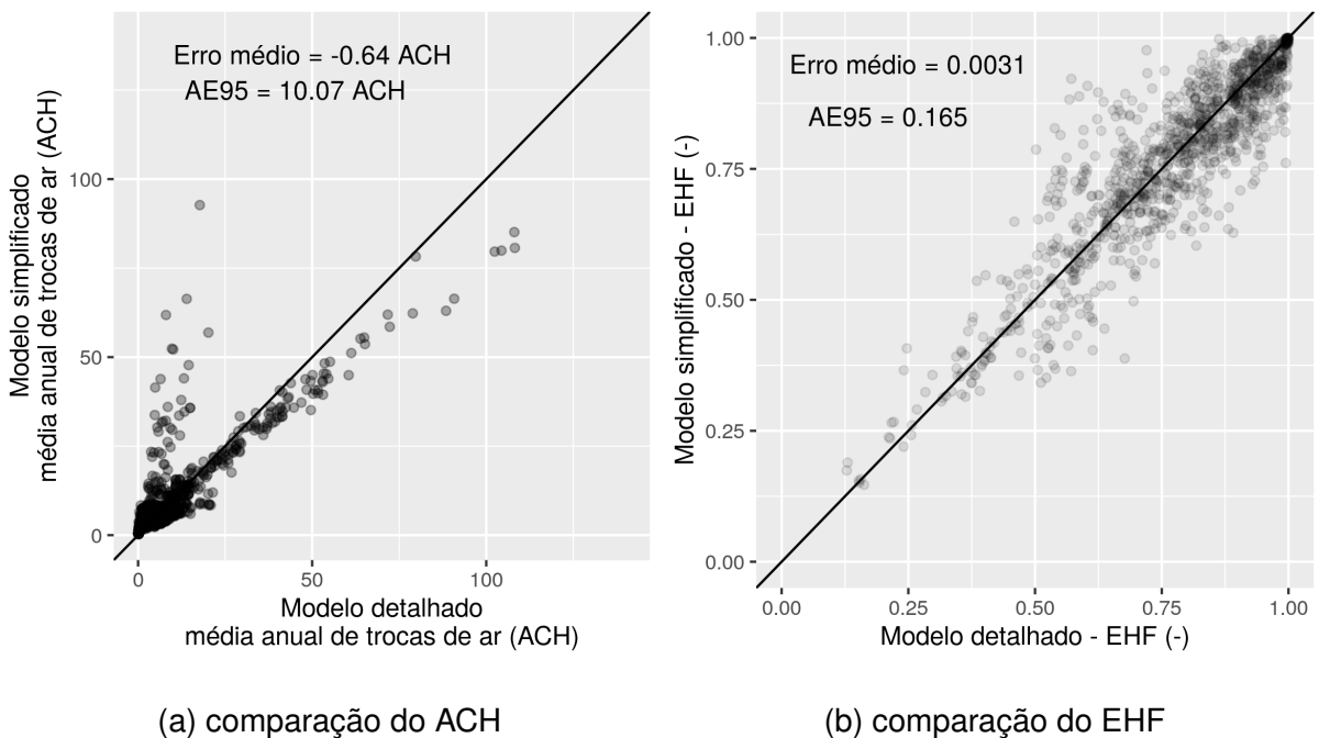
Figura 21 – Comparação entre os resultados de ACH e EHF para coeficiente de vazão mássica de ar com valor igual 0,1 \text{ kg/sPa}^n em 1 Pa
