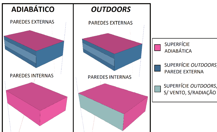
Figura 9 – Modelagem com parede adiabática e outdoors
