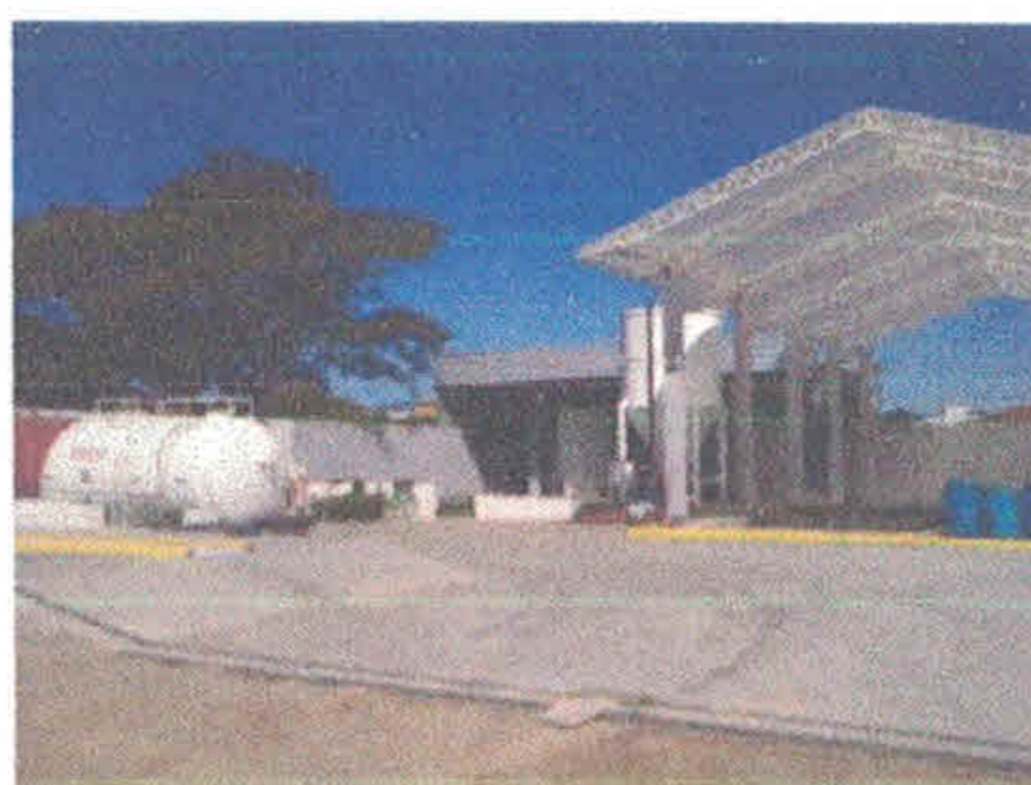
USTE – Unidade Solar de Tratamento de Efluentes
