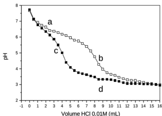
Figura 5. Curva de titulação potenciométrica do efluente antes e após incubação com a lacase imobilizada por 24 horas utilizando como titulante solução de HCl 0,01 M. O (□) representa o efluente sem tratamento e o (■) após tratamento. Os pontos das curvas representam as médias de 3 repetições
