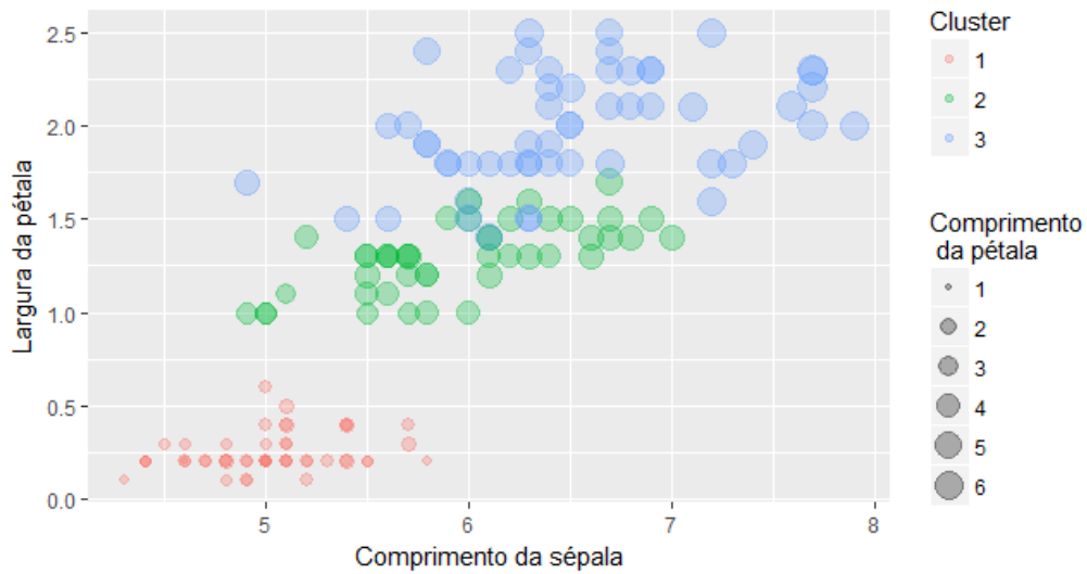
Figura 9. Representação dos clusters da Iris obtidos com dissimilaridade pelo cosseno
