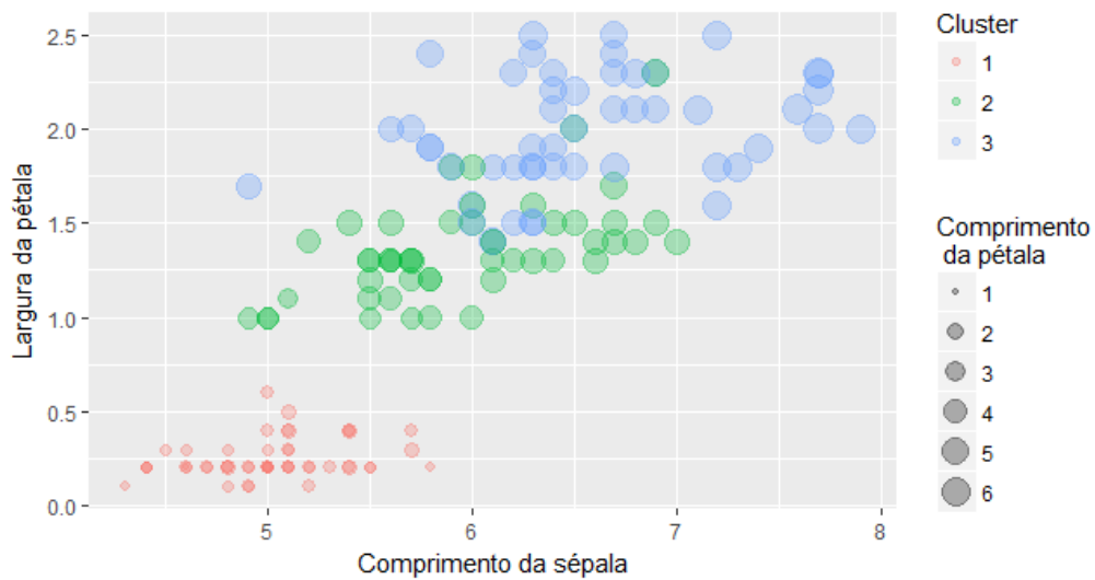
Figura 10. Representação dos clusters da Iris obtidos com dissimilaridade por correlação
