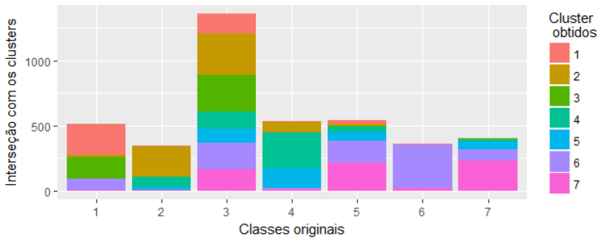
Figura 27. Interseção dos grupos de Denver e os clusters obtidos com dissimilaridade por correlação
