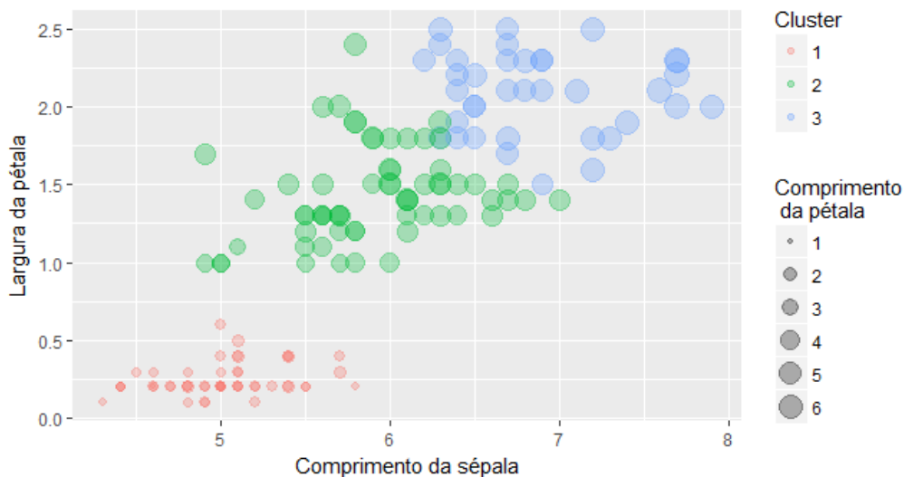
Figura 8. Representação dos clusters da Iris obtidos com métrica Manhattan
