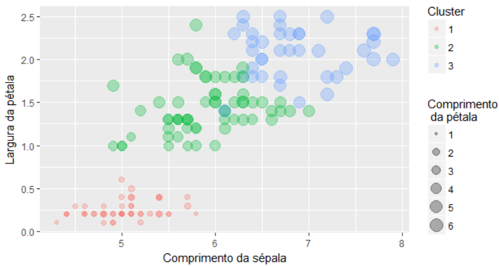
Figura 7. Representação dos clusters da Iris obtidos com distância euclidiana ao quadrado
