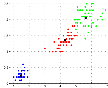
h) 8ª iteração
