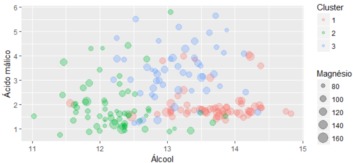
Figura 13. Representação dos clusters dos vinhos obtidos com distância euclidiana ao quadrado
