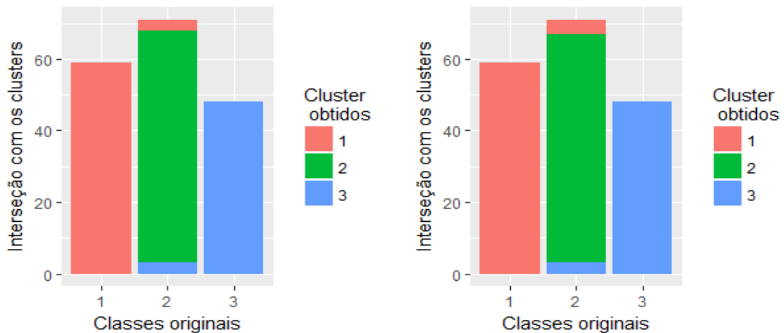
(a) Interseção das classes de vinho e os clusters obtidos com distância euclidiana ao quadrado (b) Interseção das classes de vinho e os clusters obtidos com distância Manhattan
