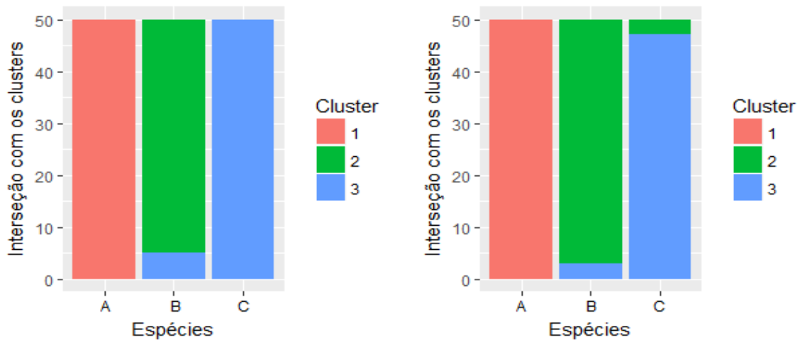
(c) Interseção das espécies da Iris e os clusters obtidos com dissimilaridade pelo cosseno (d) Interseção das espécies da Iris e os clusters obtidos com dissimilaridade por correlação
