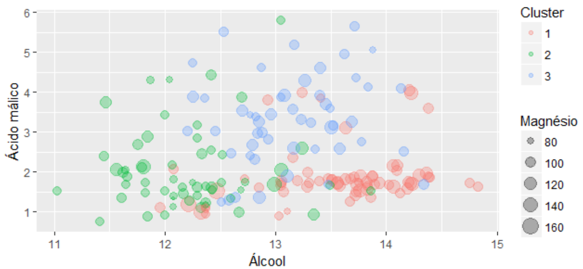
Figura 15. Representação dos clusters dos vinhos obtidos com dissimilaridade pelo cosseno
