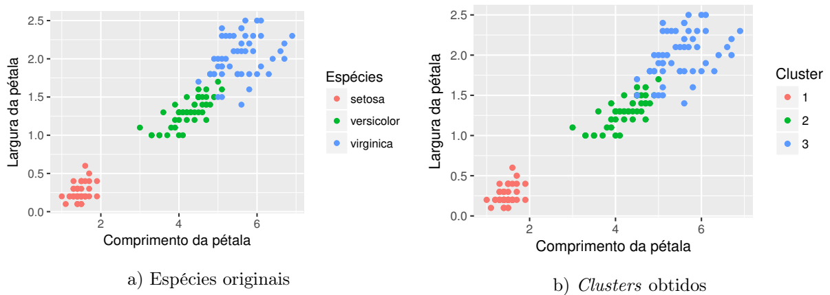
Figura 6. Comparação das espécies da flor Iris com dos clusters obtidos pelo método k-means com a dissimilaridade por correlação
