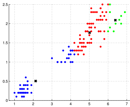
a) 1ª iteração
