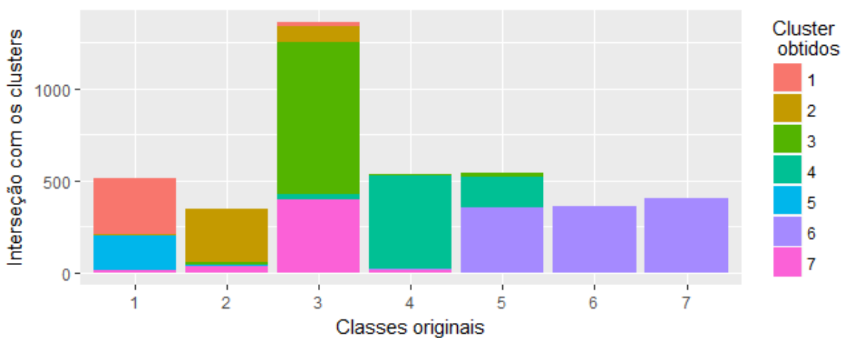
Figura 24. Interseção dos grupos de Denver e os clusters obtidos com distância euclidiana ao quadrado
