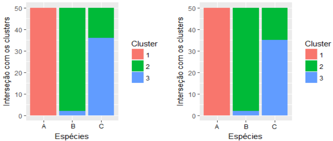
(a) Interseção das espécies da Iris e os clusters obtidos com distância euclidiana ao quadrado (b) Interseção das espécies da Iris e os clusters obtidos com distância Manhattan
