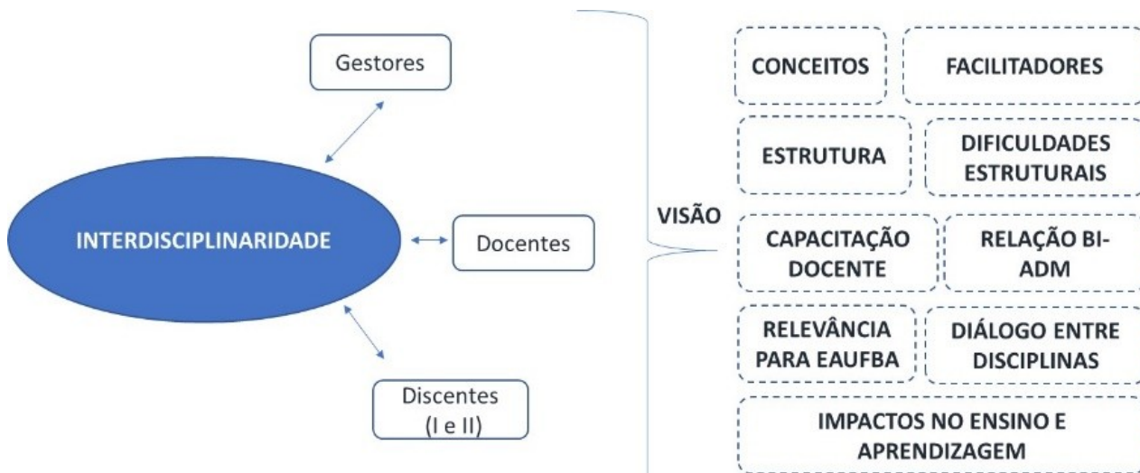
Figura 2- Modelo conceitual
