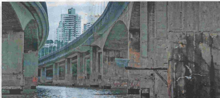
Ponte Colombo Salles (à dir.), construída em 1974 e que nunca passou por reforma, revela cenário assustado vista de baixo
