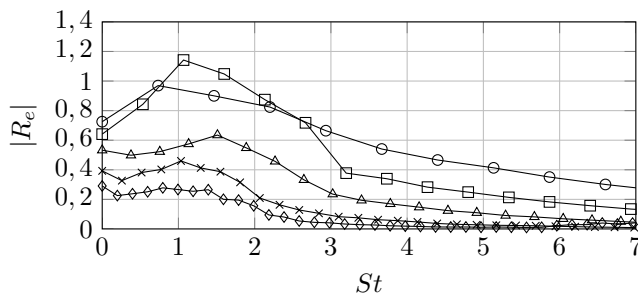
Figura 22: Resultado de |R_e| em relação ao número de Strouhal ( St ) com vários escoamentos sugados. Os pontos com ○, □, △, × e ◇ apresentam os resultados para M = 0,05 e Re = 1378,73 , M = 0,07 e Re = 1930,23 , M = 0,1 e Re = 2757,42 , M = 0,15 e Re = 2057,71 e M = 0,20 e Re = 5514,82 respectivamente.
