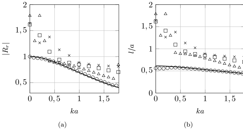
Figura 11: Resultados de |R_r| (11a) e l/a (11b) para duto sem escoamento. As linhas contínuas representam os resultados do modelo analítico exato de Levine e Schwinger (1948) e os pontos \circ , \triangle , \square e \times apresentam os resultados para 20, 15, 10 e 5 elementos de discretização para representar o raio do duto respectivamente.
