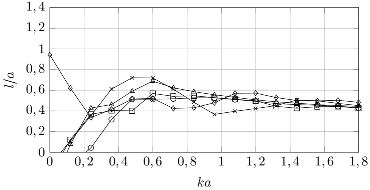
Figura 20: Resultados de l/a em função de ka para diferentes números de Mach com escoamento sugado. com vários escoamentos sugados. Os pontos com \circ , \square , \triangle , \times e \diamond apresentam os resultados para M = 0,05 e Re = 1378,73 , M = 0,07 e Re = 1930,23 , M = 0,1 e Re = 2757,42 , M = 0,15 e Re = 2057,71 e M = 0,20 e Re = 5514,82 respectivamente.
