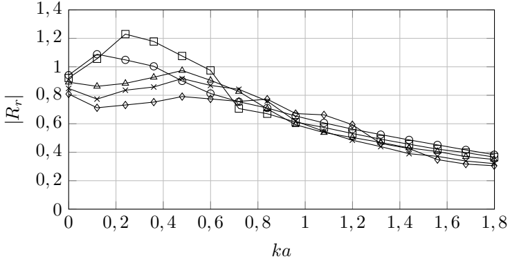
Figura 19: Resultados de |R_r| em função de ka para vários números de Mach de escoamento sugado. Os pontos com \circ , \square , \triangle , \times e \diamond apresentam os resultados para M = 0,05 e Re = 1378,73 , M = 0,07 e Re = 1930,23 , M = 0,1 e Re = 2757,42 , M = 0,15 e Re = 2057,71 e M = 0,20 e Re = 5514,82 respectivamente.
