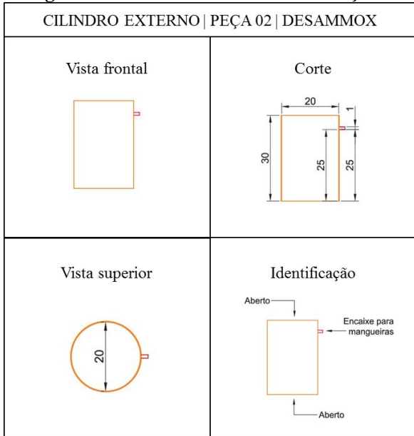
Figura 2.4. Reator DESAMMOX – Peça 02
