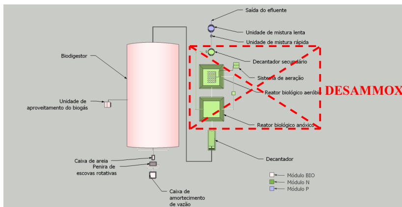
Figura. Representação esquemática de um pacote tecnológico desenvolvido para o tratamento de efluentes da suinocultura.
