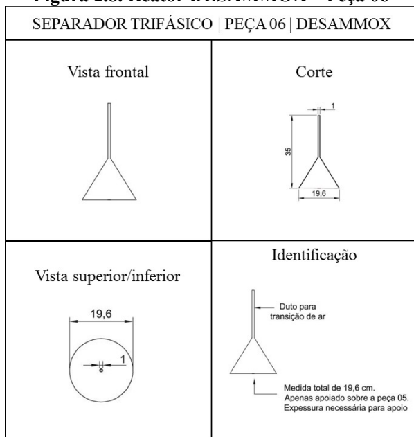
Figura 2.8. Reator DESAMMOX – Peça 06
