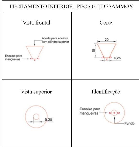
Figura 2.3. Reator DESAMMOX – Peça 01
