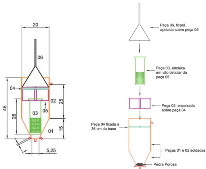
Figura 2.2. Vista frontal detalhada do projeto e esquema de montagem do reator DESAMMOX. Unidade de medida em centímetros.
