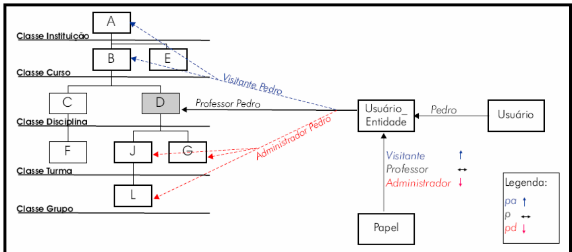
Figura 7 - Propagação de papéis por chaveamento.
