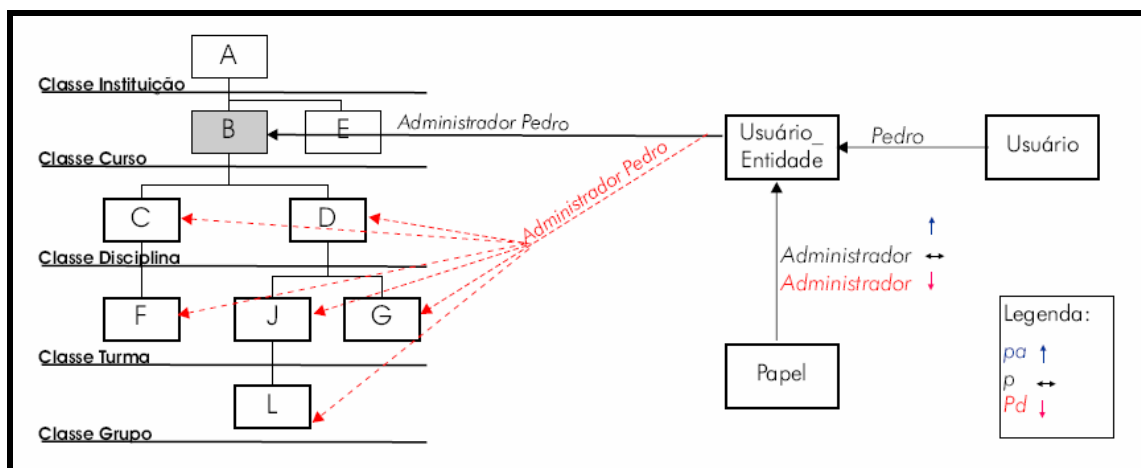
Figura 6 - Propagação de papéis por herança.
