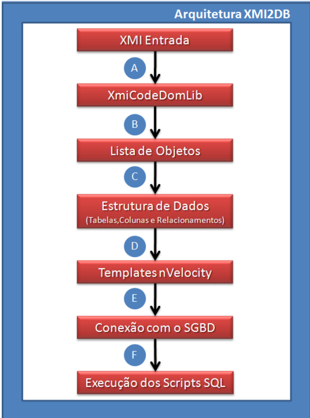
Figura 6: Arquitetura da ferramenta no caminho XMI->DB
