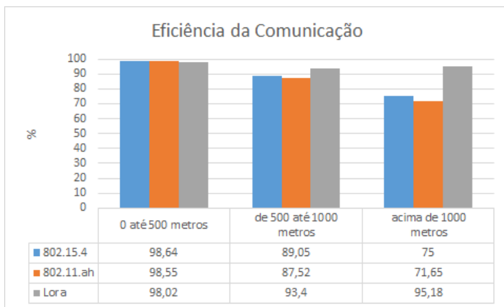
Figura 17 – Comparativo Eficiência - Cenário 1
