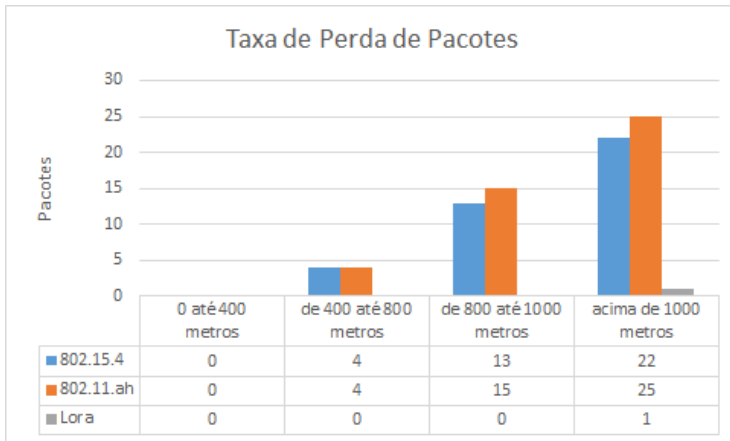
Figura 19 – Comparativo TPP - Cenário 2
