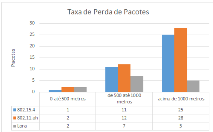
Figura 16 – Comparativo TPP - Cenário 1
