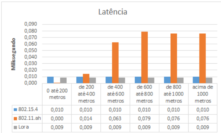
Figura 27 – Comparativo Latência - Cenário 4
