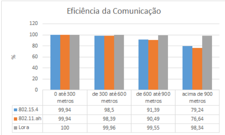
Figura 23 – Comparativo Eficiência - Cenário 3
