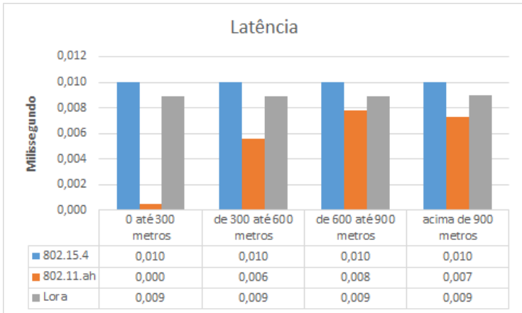
Figura 24 – Comparativo Latência - Cenário 3
