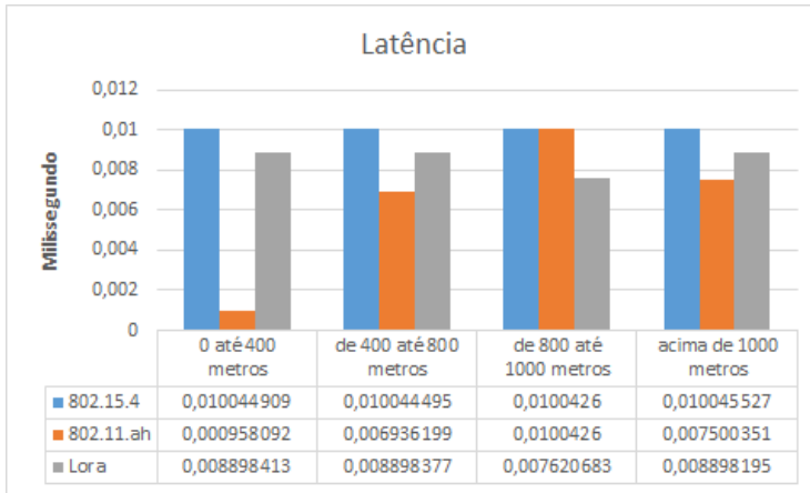
Figura 21 – Comparativo Latência - Cenário 2
