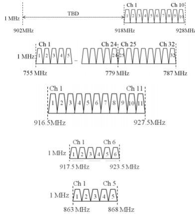
Figura 4 – Atribuição de canais do padrão 802.11ah
