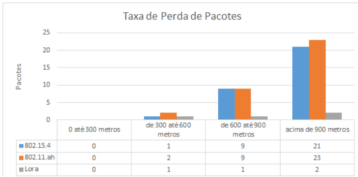
Figura 22 – Comparativo TPP - Cenário 3
