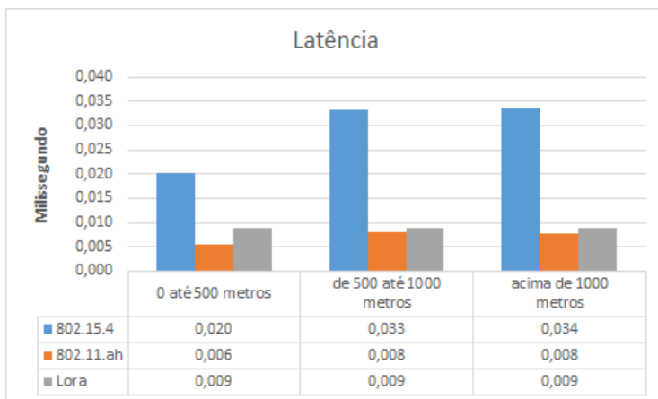
Figura 18 – Comparativo Latência - Cenário 1
