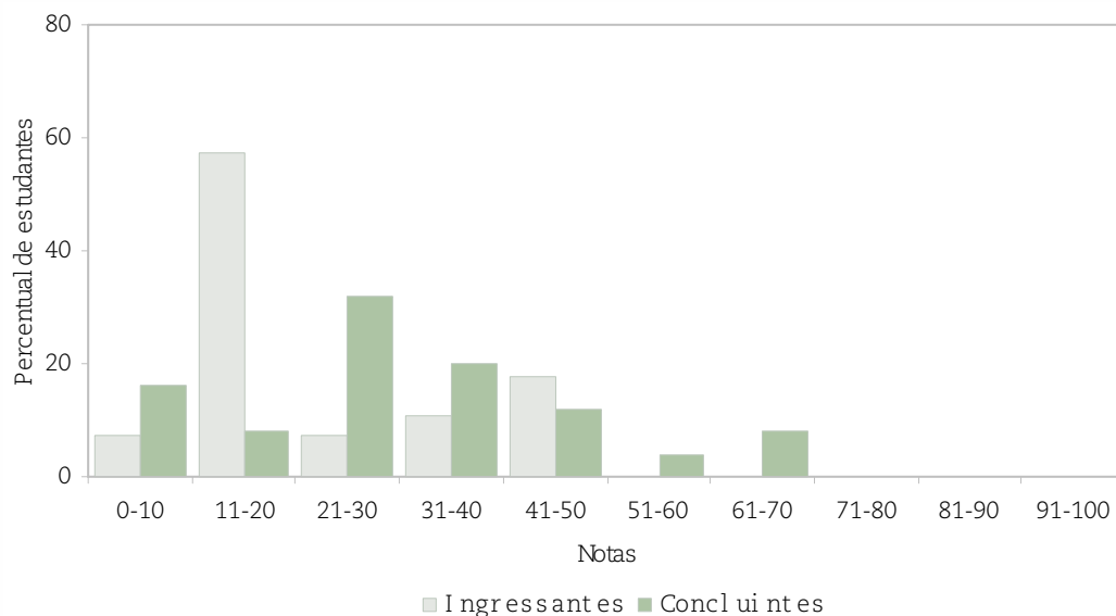
Percentual de notas obtidas pelos alunos na parte de Componente Específico da prova de Química
