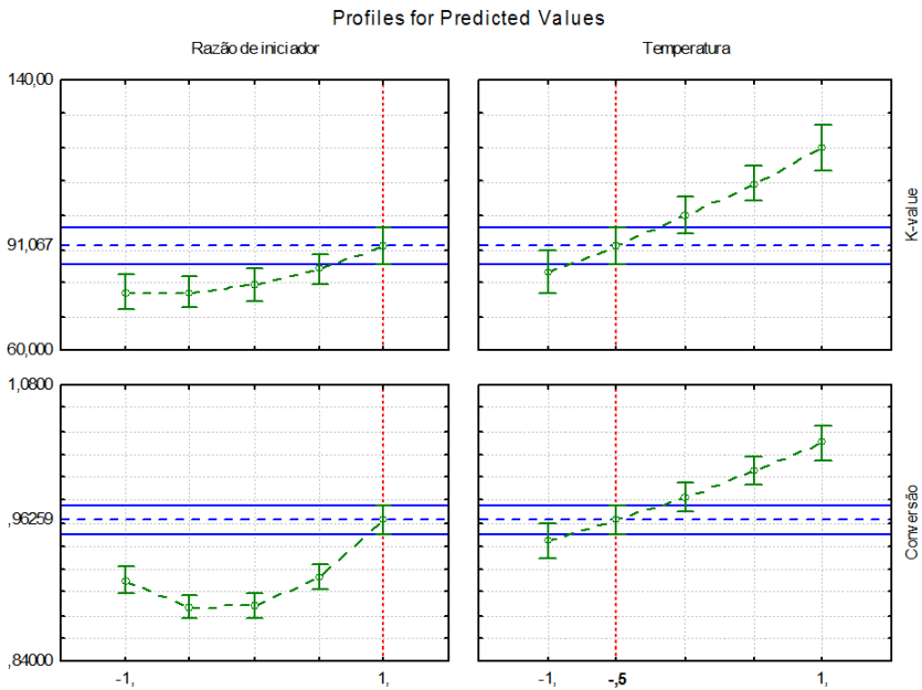
Figura 4.7 – Gráfico de interação entre respostas para ponto (+1;-0,5) do planejamento.
