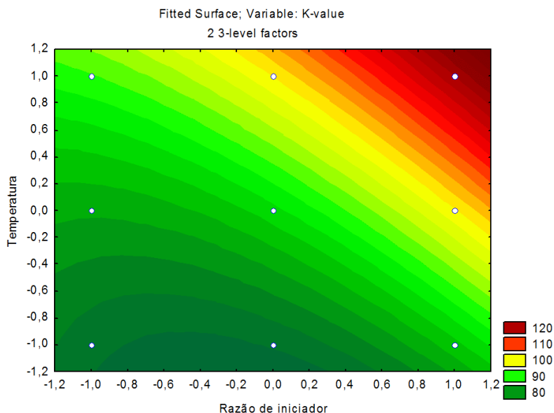
Figura 4.2 – Superfície de resposta para a massa molar viscosimétrica.
