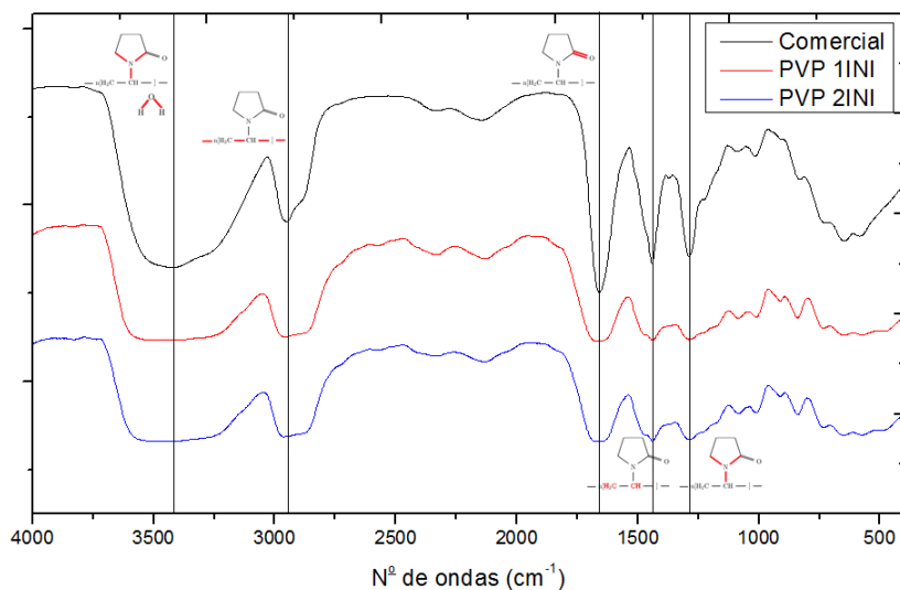
Figura A.2 – Gráfico dos espectros de FTIR da poli(pirrolidona vinílica).
