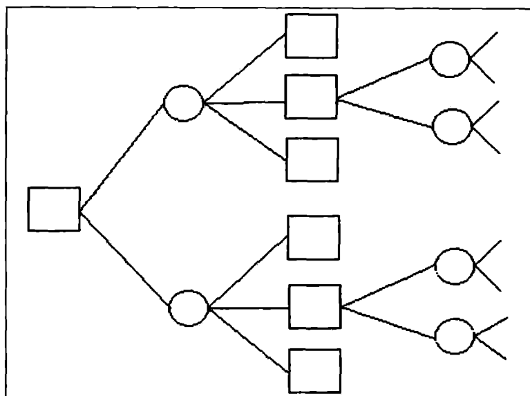
Figura 7: Estrutura de uma árvore de decisão fonte: Kassai et al (2000, p. 113)
