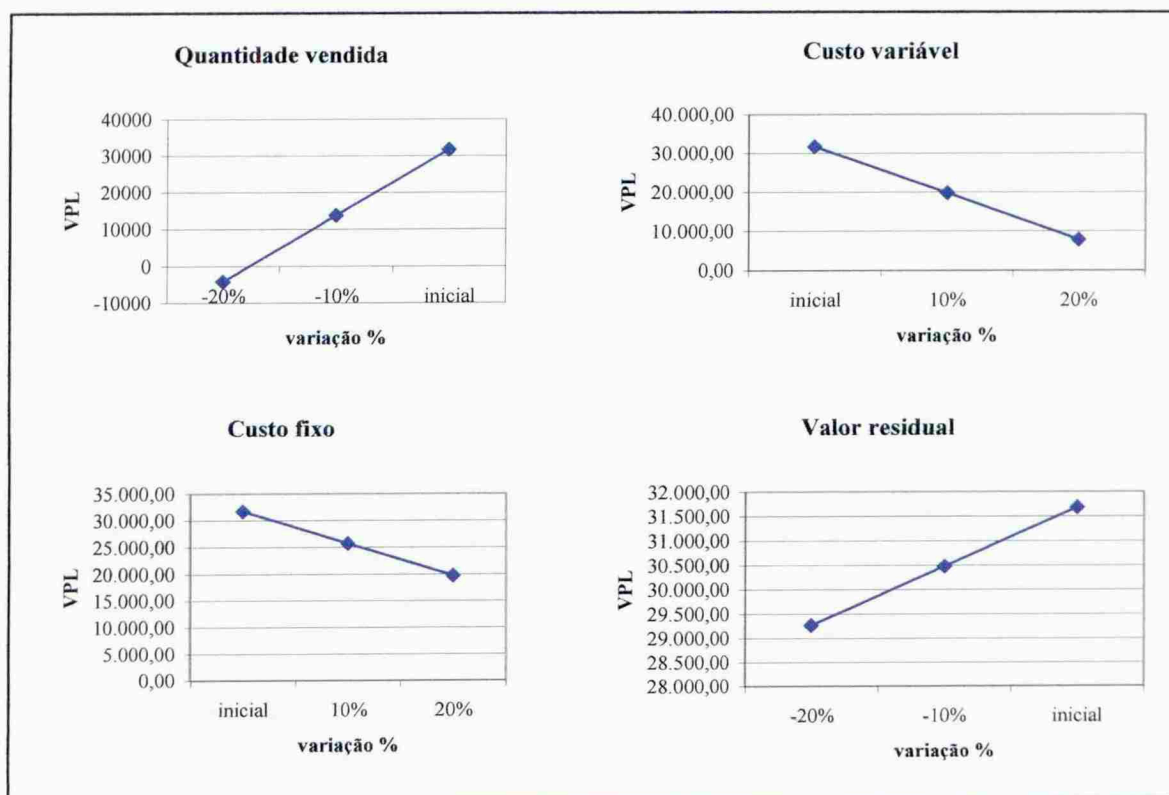
Gráfico 1: gráficos evidenciando a variação do VPL. Fonte: elaborado pela autora com base em Sanvicente (1987, p.71)
