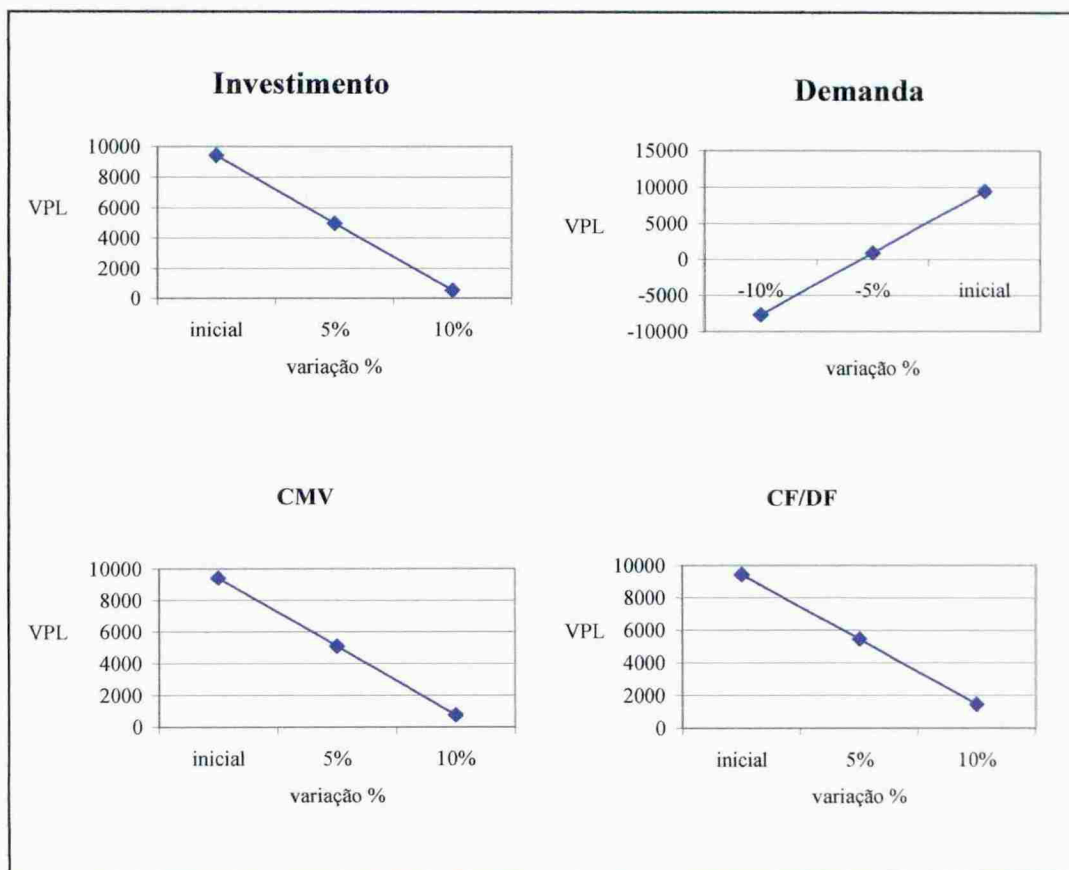
Gráfico 3: gráficos evidenciando a variação do VPL
