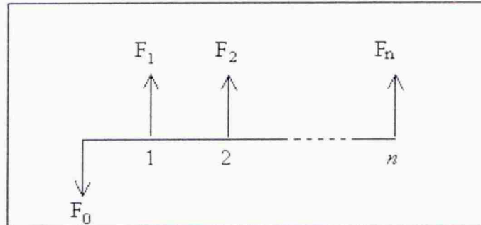
Figura 1: Fluxo de caixa de um projeto de investimento. fonte: Hirschfeld (1992, p.387)
