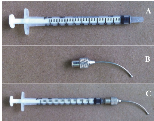
Fig.1. Seringa utilizada no método da gavagem. (A) Seringa plástica de insulina. (B) Ponta de seringa Luer. (C) Conjunto de seringa com ponta para a gavagem.
