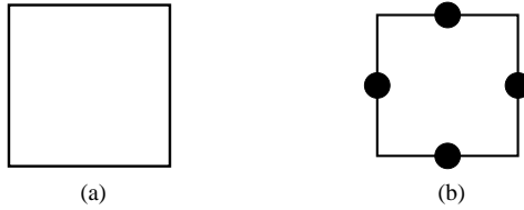
Figura 62: (b) ilustra a associação de um vértice a cada lado do módulo quadrado em (a).
