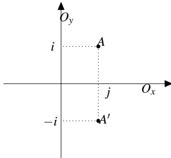
Figura 40: Ponto A de coordenadas \{j, i\} e seu simétrico em relação à O_x , A' , de coordenadas \{j, -i\} .
